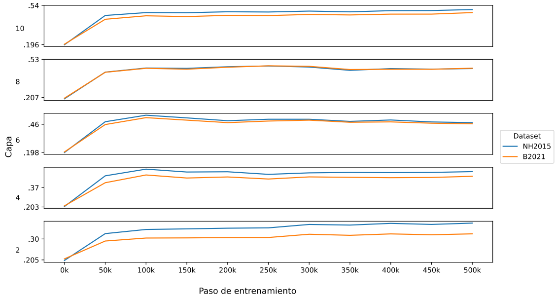
Figura 5.13: \rho de Spearman del análisis de RSA en el conjunto de datos B2021 y NH2015 para cada capa a lo largo del preentrenamiento.
