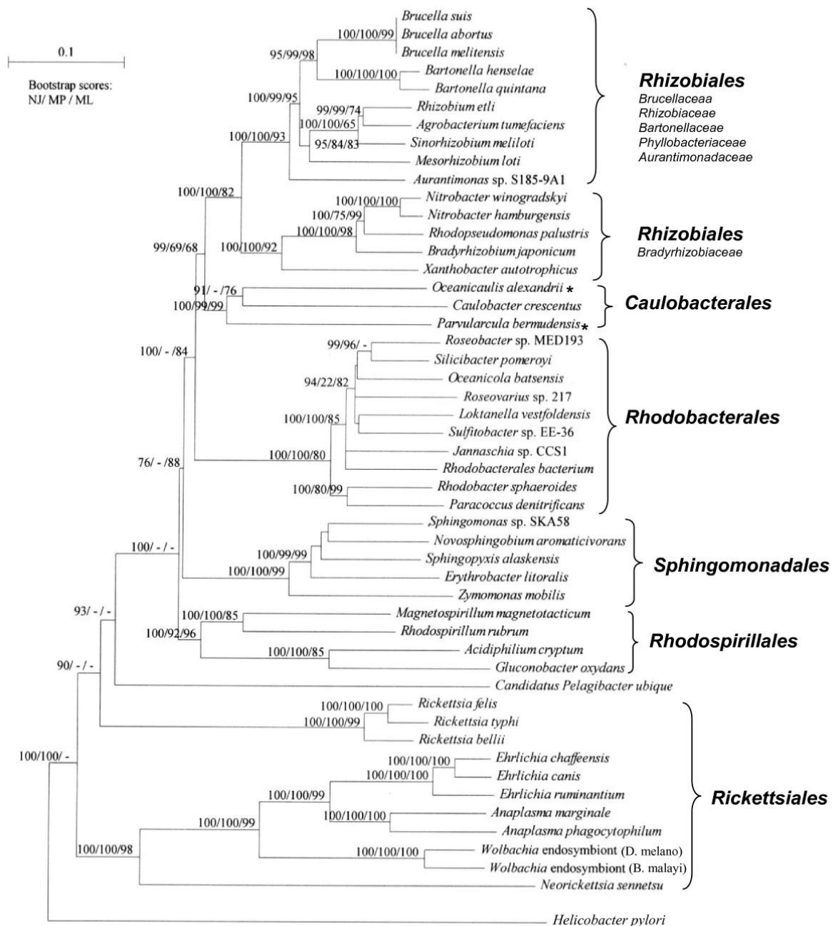
Figura 1. Árbol filogenético de la clase \alpha -proteobacteria. Construido mediante el método Neighbor-joining a partir de la selección de 12 proteínas conservadas. Extraído de Gupta, R.S., Mok, A, 2007 [28].
