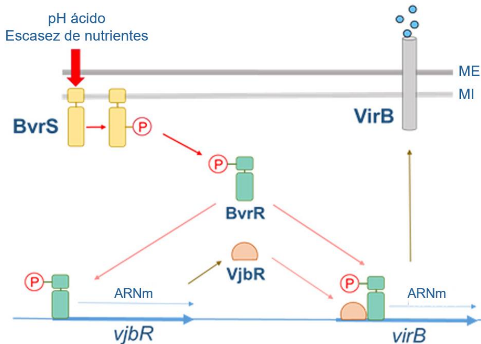
Figura 3. Regulación del operón virB por el sistema BvrS/BvrR. Regulación tanto directa como indirecta (mediante la expresión de VjbR) del sistema de secreción de tipo IV codificado por el operón virB . Los círculos celestes representan proteínas efectoras siendo secretadas hacia el exterior. ME: membrana externa. MI: membrana interna. ARNm: ARN mensajero. Adaptado de Altamirano-Silva et al , 2018 [65].
