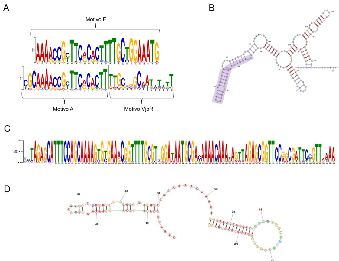
Figura 14. Identificación del elemento EBC. A) Motivo E obtenido a partir de la reevaluación de los motivos A y VjbR. B) TPP riboswitch presente en el extremo 5'UTR del locus bab1_1770 . La región resaltada presenta un ajuste significativo al motivo E. Modelo extraído de la base de datos "RiboD". C) Motivo EBC identificado al analizar mediante el software MEME aquellos promotores con presencia (con un buen nivel de ajuste) de los motivos E, B y C. D) Estructura de ARN predicha para la secuencia río arriba del locus bab1_1279 identificada con un alto nivel de ajuste al motivo EBC. Estructura secundaria obtenida mediante el uso del software "RNAstructure".
