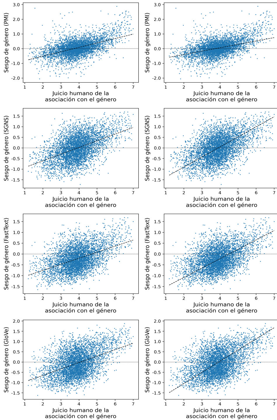
Figura 4.3: Relación entre el sesgo de género textual y de acuerdo al juicio humano en las palabras de Lewis y Lupyán [2020]. Cada punto representa una palabra objetivo. Las rectas representan un ajuste lineal de los datos. En la segunda fila el ajuste pondera cada punto por el error estándar de la estimación de sesgo textual (los intervalos de confianza asociados no se muestran para mayor claridad).
