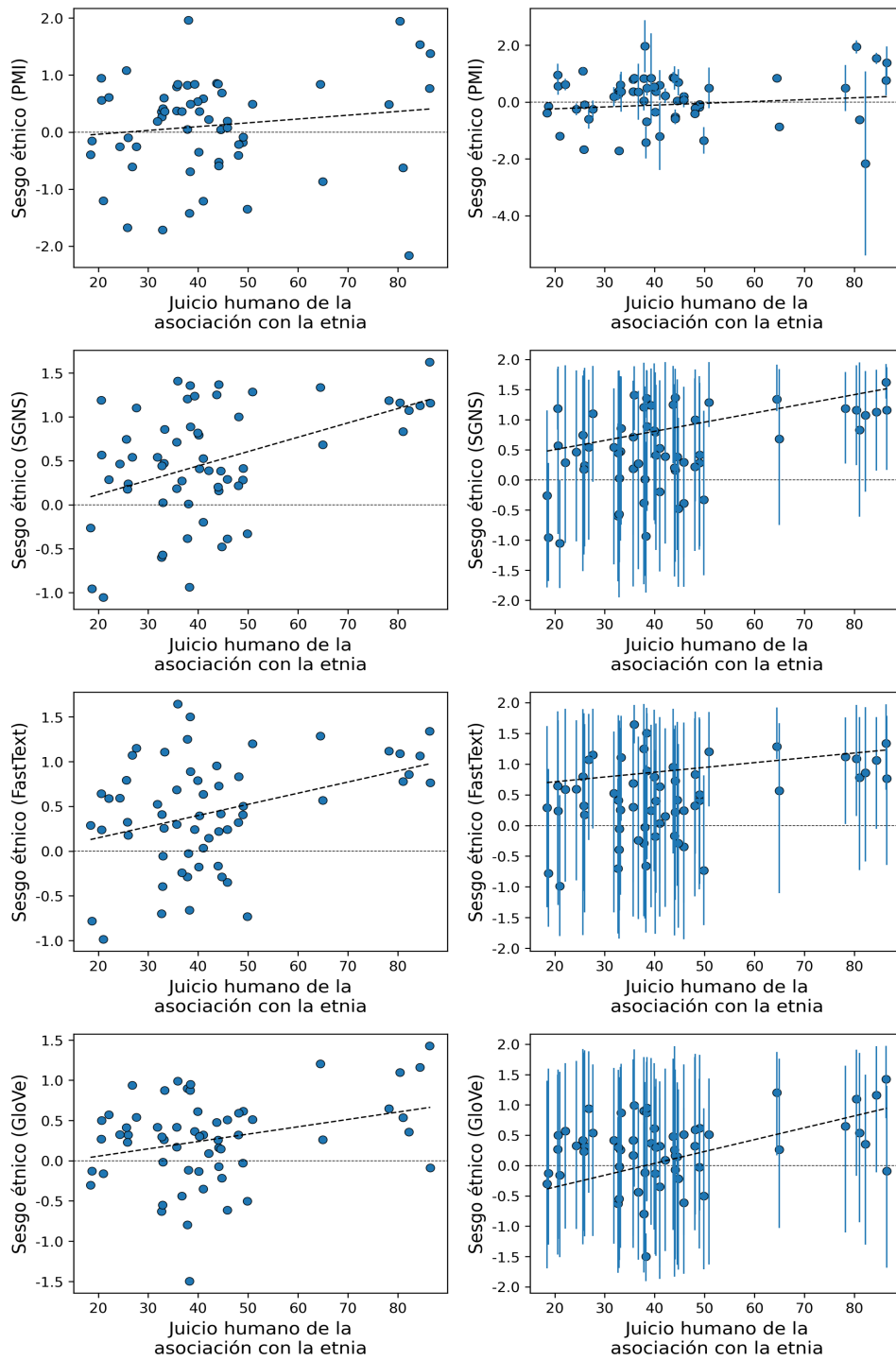
Figura 4.5: Relación entre el sesgo étnico textual y de acuerdo al juicio humano en las palabras de Kozlowski et al. [2019]. Cada punto representa una palabra objetivo. Las rectas representan un ajuste lineal de los datos. En la segunda fila el ajuste pondera cada punto por el error estándar de la estimación de sesgo textual (los intervalos de confianza se indican con barras de error).
