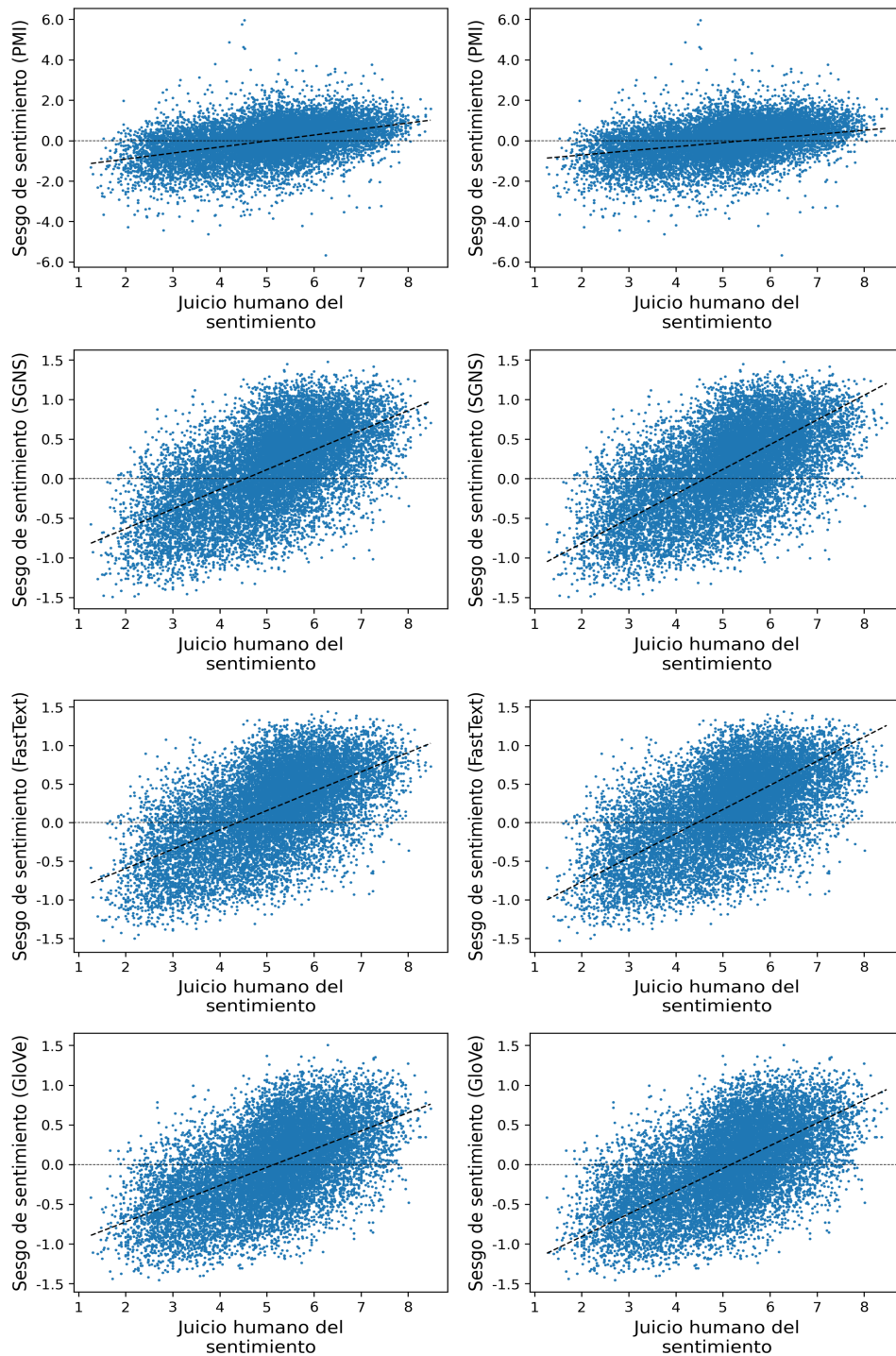
Figura 4.4: Relación entre el sesgo de sentimiento textual y de acuerdo al juicio humano en las palabras de Toney y Caliskan [2021]. Cada punto representa una palabra objetivo. Las rectas representan un ajuste lineal de los datos. En la segunda fila el ajuste pondera cada punto por el error estándar de la estimación de sesgo textual (los intervalos de confianza asociados no se muestran para mayor claridad).
