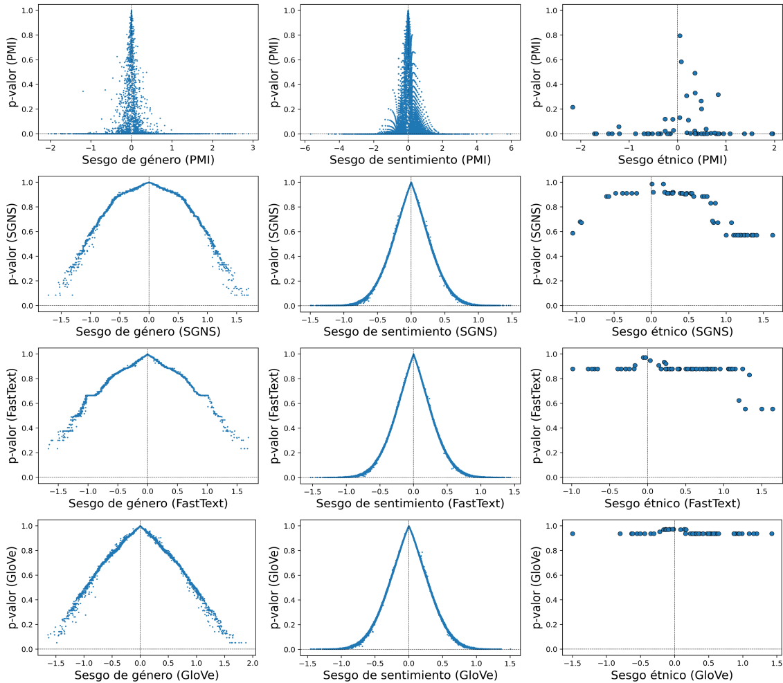
Figura 4.1: p-valores (eje vertical) en función del valor del sesgo (eje horizontal) para cada tipo de sesgo y cada método de medición.
