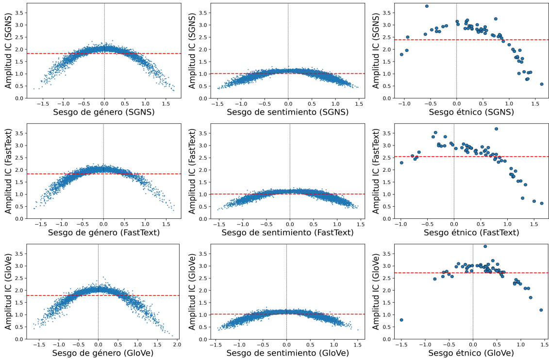
Figura 4.2: Amplitud de los intervalos de confianza al 95 % de \text{Bias}_{\text{WE}} (eje vertical) en función del valor del sesgo (eje horizontal), para cada tipo de sesgo y cada método de entrenamiento de embeddings . En rojo se indica el promedio.
