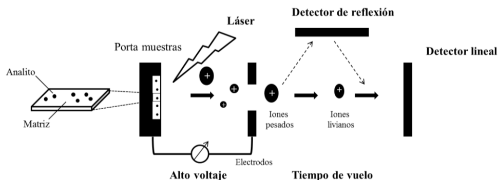
Figura 3.5: Esquema del recorrido de los iones en un equipo MALDI-TOF.
