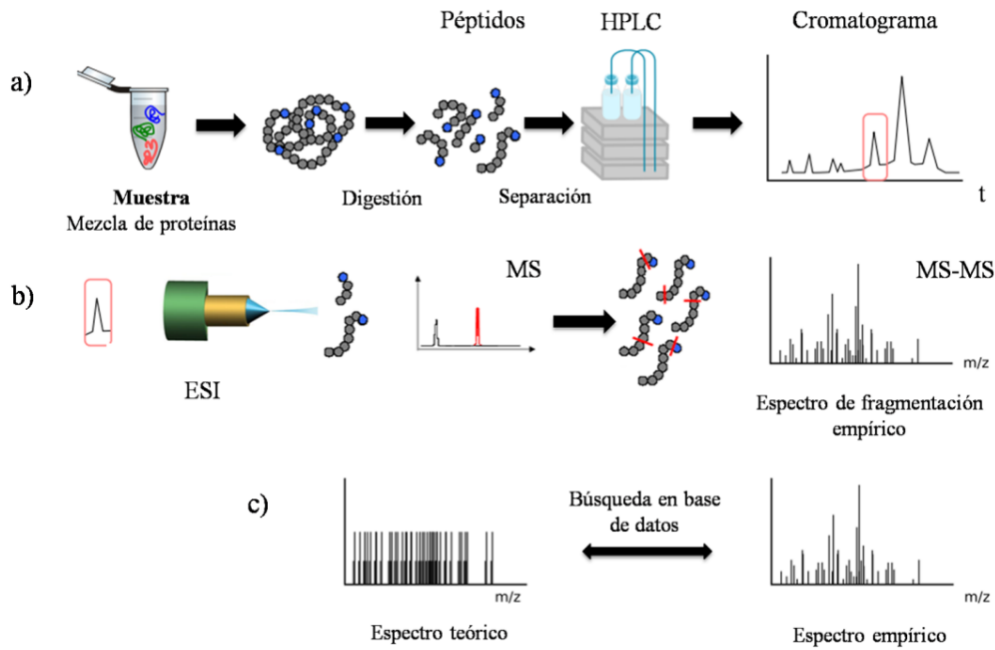
Figura 3.9: Etapas en un experimento de proteómica. a) En primer lugar la muestra de proteínas es digerida en péptidos que se separan cromatográficamente, frecuentemente por HPLC. A medida que eluyen los péptidos, son introducidos en el espectrómetro de masa generando su correspondiente espectro. b) Cada péptido puede seleccionarse y fragmentarse obteniendo un segundo espectro de fragmentación MS-MS característico. c) Por último el motor de búsqueda compara los espectros empíricos con espectros teóricos asignando una puntuación de acuerdo al grado de coincidencia entre ambos espectros.
