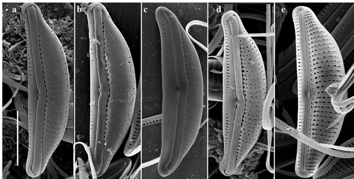
Figura 2.11: Imágenes de MEB de células de H. luciae en el medio f/2-P. Escala= 5 \mu m.
