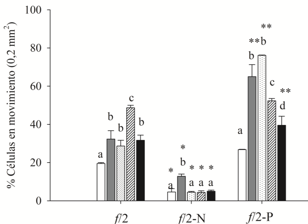
Figura 2.18: Porcentaje de células en movimiento cultivadas en el medio f/2 , f/2-N y f/2-P luego de 4 (barras blancas), 9 (barras grises), 13 (barras punteadas), 15 (barras rayadas) y 20 (barras negras) días de crecimiento. Letras distintas indican diferencias significativas ( P < 0,05 ) dentro de cada tratamiento. Los asteriscos indican diferencias significativas (un asterisco, P < 0,05 y dos asteriscos, P < 0,01 ) respecto f/2 . Los valores corresponden a la media \pm DS ( n=20 ).
