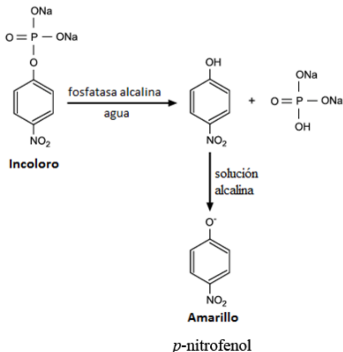
Figura 5.4: Fosfato de p -nitrofenilo como sustrato para la medición de la actividad fosfatasa alcalina.
