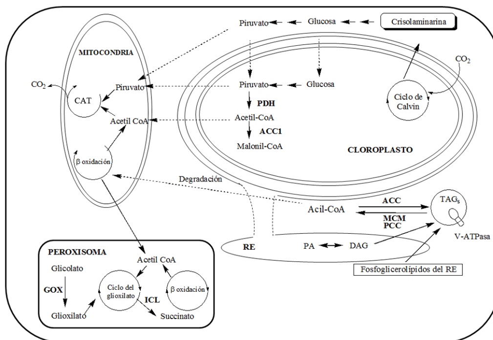
Figura 4.21: Esquema del metabolismo de la acumulación de lípidos. ACC1: acetil CoA carboxilasa, DAG: diacilglicérido, GOX: glicolato oxidasa, ICL: isocitrato liasa, PA: ácido fosfatídico, RE: retículo endoplasmático, TAGs: triacylglicérido, PCC: propionilCoA carboxilasa, MCM: metilmalonilCoA mutasa.
