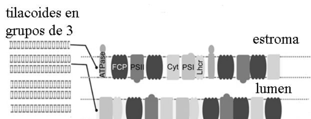
Figura 4.19: Diagrama de la organización de la membrana del tilacoide de la diatomea modelo Phaeodactylum tricornutum mostrando los dos fotosistemas (FSI y FSII), el complejo citocromos b_6/f , los complejos antena asociados al FSII (FCP-Lhcf) y PSI (Lhcr) y la ATP sintetasa. Modificado a partir de Herbstová et al. (2017).
