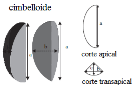
Figura 5.3: Valores morfométricos analizados en el trabajo, a: eje apical, b: eje pervalvar, c: eje transapical. Imagen modificada de Sun & Liu (2003).
