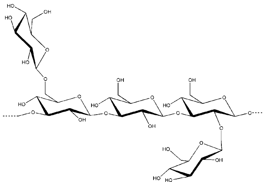
Figura 3.2: Estructura de la crisolaminarina, polisacárido de reserva de las diatomeas compuesto por una cadena principal de (1→3)-β-D-glucano, que puede presentar ramificaciones en β-(1→6) y/o β-(1→2). En esta figura se ejemplifica con ramificaciones simples de glucosa.
