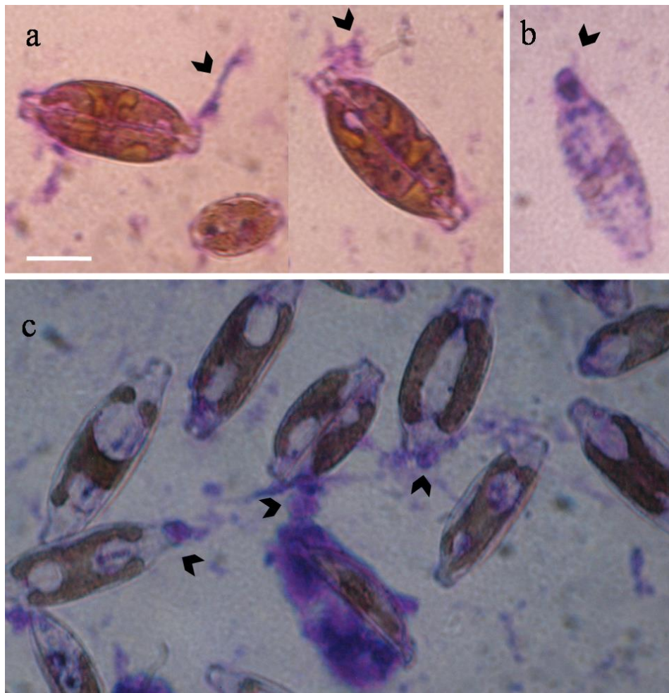
Figura 2.20: Tinción de mucílago extracelular de células de H. luciae cultivadas durante 10 días en los medios, a) f/2 , b) f/2-N y c) f/2-P . Las flechas negras señalan la huella mucilaginosa. Escala= 10 \mu\text{m} .
