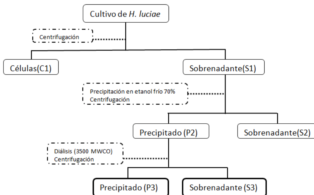
Figura 5.6: Esquema general de la obtención de las fracciones de la cosecha.
