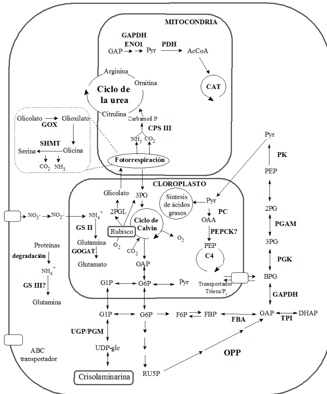
Figura 4.20: Esquema del metabolismo de los hidratos de carbono y la fotorrespiración propuesto para H. luciae . 2PG: 2-fosfoglicerato, 2PGL: 2-fosfoglicolato, 3PG: 3-fosfoglicerato, AcCoA: acetil-CoA, BPG: 1,3 difosfoglicerato, CPS III: carbamoil-fosfato sintetasa 3, DHAP: dihidroxiacetona fosfato, ENO1: \alpha -enolasa 1, F6P: fructosa-6- fosfato, FBA: fructosa-1,6-bisfosfato aldolasa, FBP: fructosa-1,6-bisfosfato, G1P: glucosa-1-fosfato, G6P: glucosa-6-fosfato, GAP: gliceraldehído-3-fosfato, GAPDH: gliceraldehído-3-fosfato deshidrogenasa, GOGAT: glutamato sintetasa, GOX: glicolato oxidasa, GS: glutamino sintetasa, P i : fósforo inorgánico, PC: piruvato carboxilasa, PDH: piruvato deshidrogenasa, PEP: fosfoenolpiruvato, PGAM: fosfoglicerato mutasa, PGK: fosfoglicerato quinasa, PK: piruvato quinasa, OAA: oxalacetato, OPP: vía oxidativa de las pentosas fosfato, Pyr: piruvato, RU5P: ribulosa-5-fosfato, Rubisco: ribulosa-1,5-bifosfato carboxilasa, SHMT: serina hidroximetil transferasa, TPI: triosa fosfato isomerasa, UGP/PGM: UDP-Glucosa-pirofosforilasa / fosfoglucomutasa, UDPglc: UDP-Glucosa.
