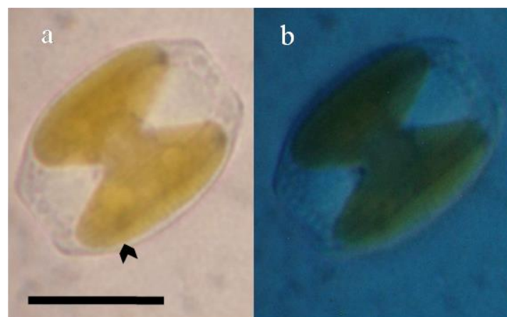
Figura 1.11: Imágenes de microscopio óptico de Halamphora luciae (a) sin filtro y (b) con filtro DIC (contraste por interferencia diferencial). Se observa el cloroplasto en forma de H (flecha negra). Escala: 10 \mu m.
