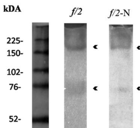
Figura 2.26: Zimograma (SDS-PAGE 10 % co-polimerizado con gelatina) de las enzimas proteasas de H. luciae cultivada en medio f /2 y f /2-N. Los marcadores de peso molecular (MPM) se muestran en la primera calle. Las flechas indican las bandas asociadas con la actividad proteasa. El gel fue revelado con azul de Coomasie.
