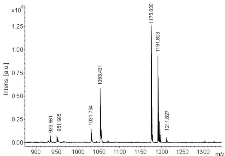
Figura 4.4: Espectro de masa MALDI de las s-EPS-P liberadas por H. luciae .
