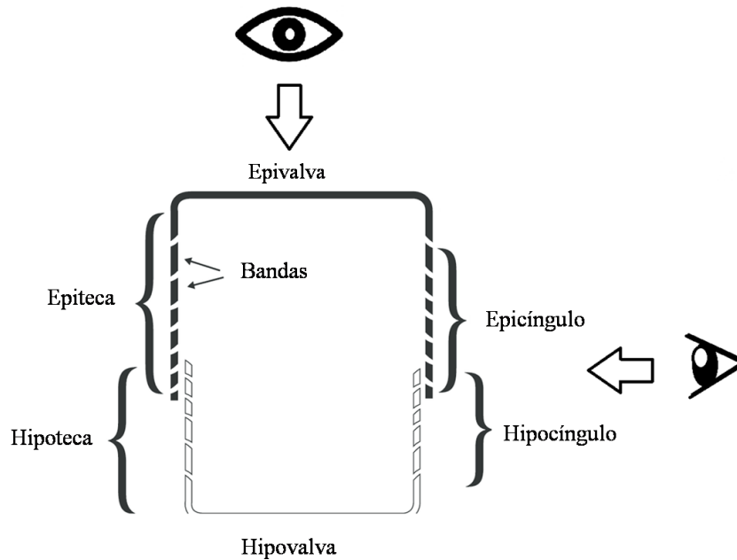
Figura 1.2: Representación del frústulo y sus elementos en vista cingular (esquema modificado de Hasle & Sylvertsen 1997). En la figura se indican las vistas valvar y cingular, dependiendo si el frústulo es observado desde arriba o desde alguno de sus lados.
