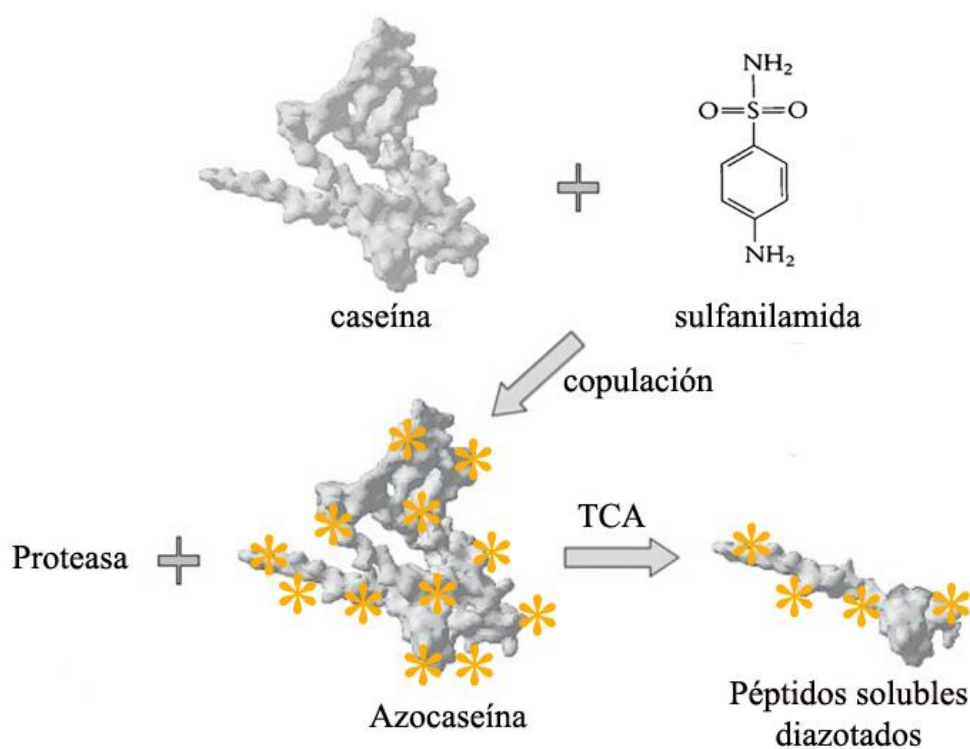
Figura 5.5: Medición de la actividad proteasa utilizando una azoproteína (azocaseína) obtenida mediante la reacción de copulación con sulfanilamida. La actividad enzimática puede cuantificarse espectrofotométricamente midiendo la aparición de péptidos coloreados solubles en TCA.
