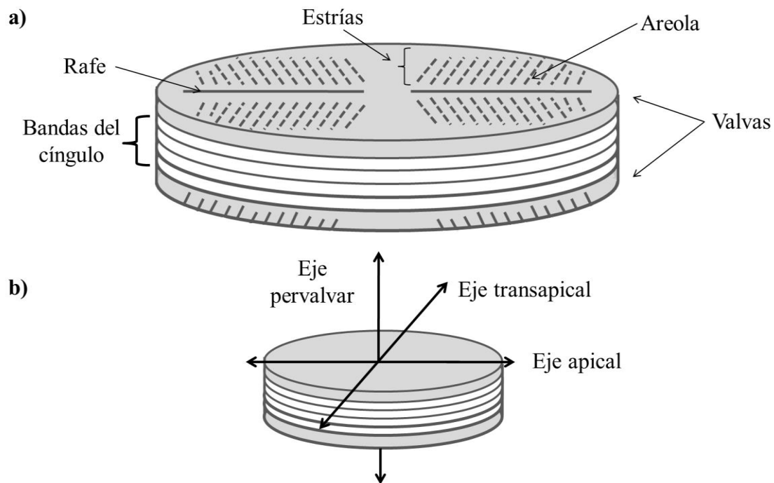
Figura 1.4: Esquema del frústulo de una diatomea pennada con rafe, a) elementos del frústulo, b) ejes de simetría en una diatomea pennada: apical, transapical y pervalvar.
