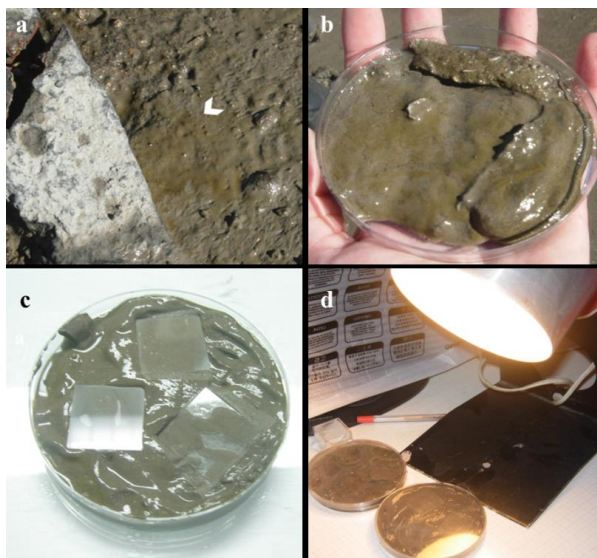
Figura 5.2: Aspecto de los sedimentos en el sitio de muestreo. (a) La flecha indica un área pigmentada donde se encontraban las diatomeas, (b) fraccionamiento de las muestras de los sedimentos en una caja de Petri, (c) colocación de los cubreobjetos sobre el papel de filtro y (d) aislamiento de las diatomeas bentónicas por fototactismo en el laboratorio.
