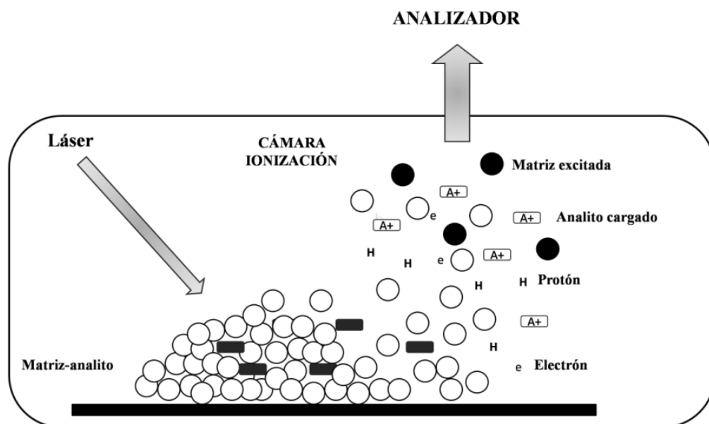
Figura 3.7: Proceso de ionización en UV-MALDI. La mezcla de matriz-analito es bombardeada con un láser UV que excita a la matriz (círculo blanco), la cual a su vez transfiere esta energía al analito (rectángulo negro). De esta forma se produce la ionización y desorción de los analitos (rectángulo blanco) como especies monocargadas (Figura adaptada de El-Aneed et al. 2009).
