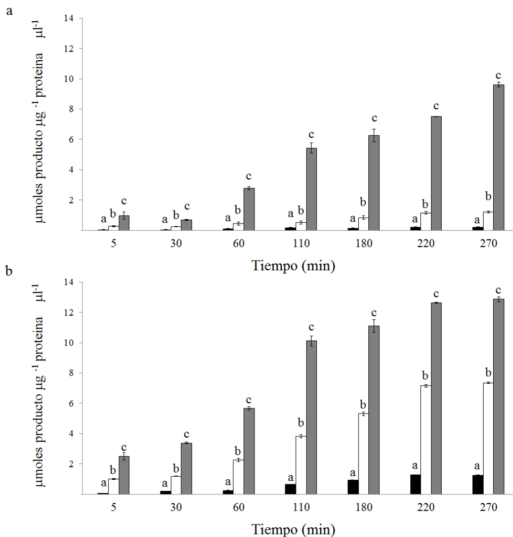
Figura 2.23: Efecto del envejecimiento del cultivo en la actividad de la fosfatasa alcalina (µmoles de producto µg -1 proteína µl -1 ) de células de H. luciae cultivadas previamente en a) medio completo y b) medio carente de fósforo, durante 5 (barras negras), 10 (barras blancas) y 20 días (barras grises). Letras distintas indican diferencias de la actividad entre cada tiempo del ensayo. Los valores corresponden a la media ± DS ( n = 3).
