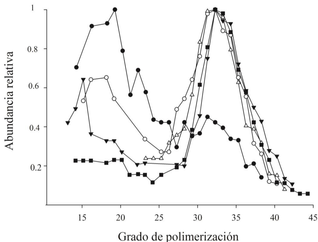
Figura 4.12: Distribución del grado de polimerización de los polímeros de las células de H. luciae cultivadas 5 (círculos negros), 10 (círculos blancos), 15 (triángulos negros), 25 (triángulos blancos) y 35 (cuadrados negros) días. La abundancia relativa se basó en el polímero que presentaba el ion de mayor intensidad, representado como una unidad en la curva.
