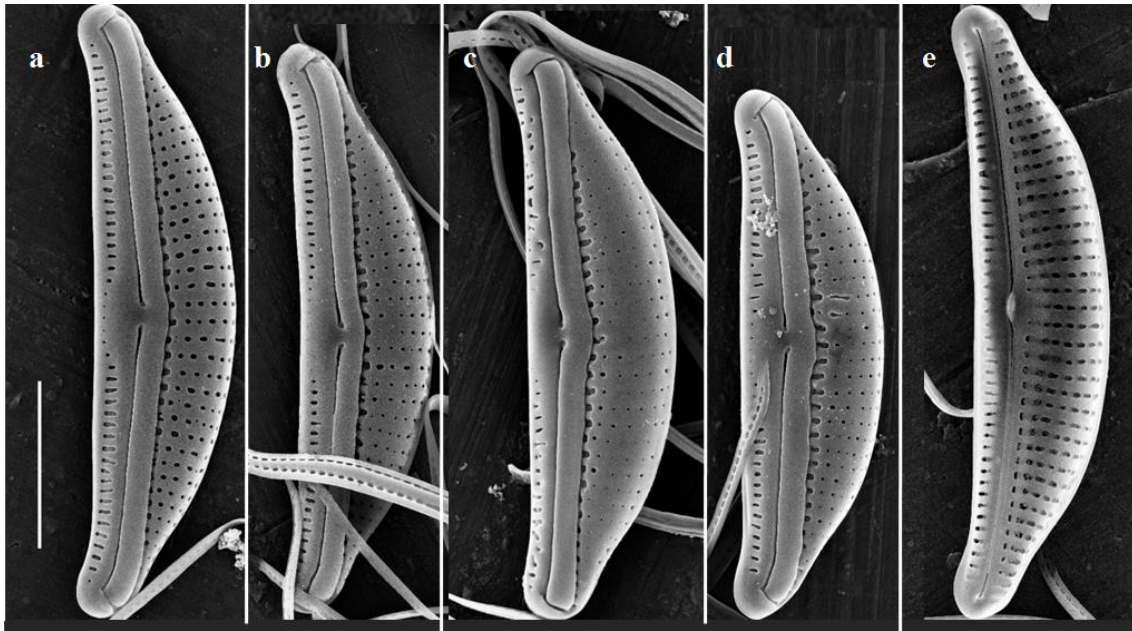
Figura 2.10 Imágenes de MEB de células de H. luciae en el medio f/2-N. Escala= 5 \mu m.
