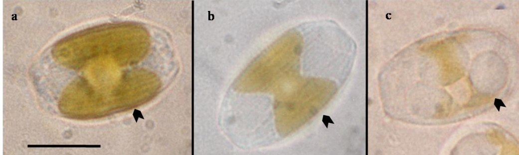
Figura 2.7: Imágenes de microscopia óptica de células de Halamphora luciae cultivada en medio a) f/2 , b) f/2-P y c) f/2-N , y cosechadas a los 10 días. Las flechas negras indican los cloroplastos. Escala=10 \mu\text{m} .
