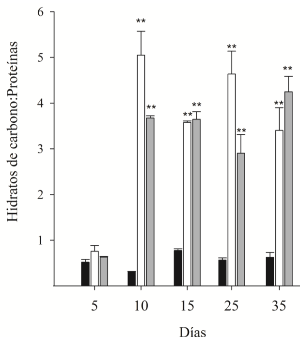
Figura 4.8: Relación hidratos de carbono: proteínas en células H. luciae crecidas en medio f/2 (negro), f/2 -N (blanco) y f/2 -P (gris). Los asteriscos indican diferencias significativas ( P < 0,01 ) respecto del control para cada día.
