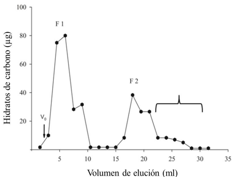
Figura 4.1: Perfil de elución del producto S3 de las s-EPS de cultivos en medio completo f /2 en la columna empacada con Bio-Gel P-2. La llave indica el rango de elución donde se detectaron sales. La flecha señala el V_0 .
