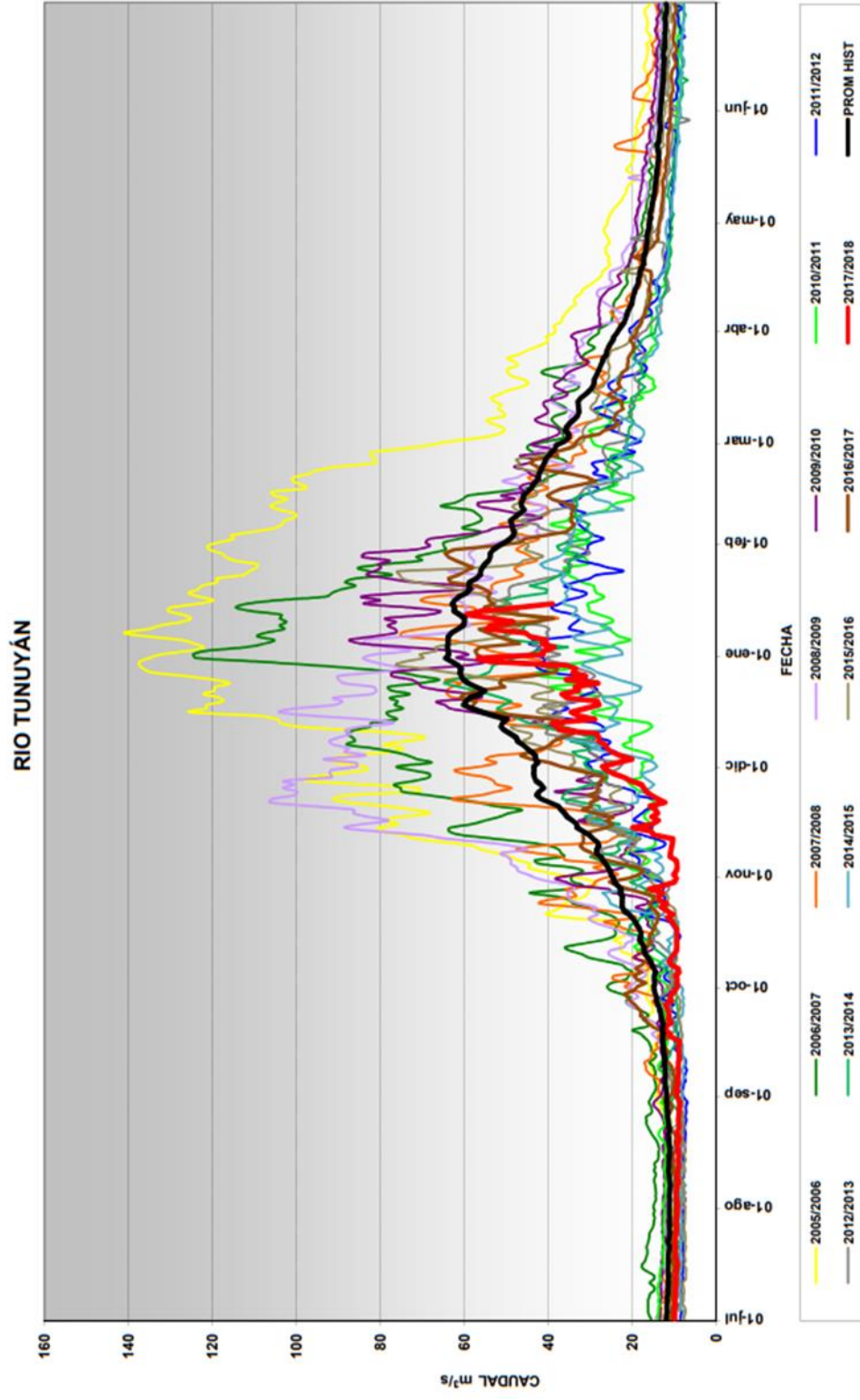
Figura 2 Anexo: Caudales medios diarios ( m^3 s^{-1} ) para el río Tunuyán.
