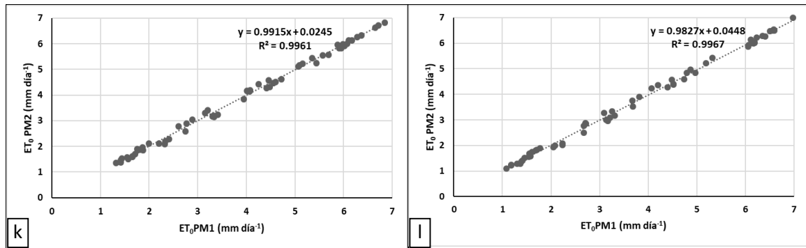
Figura 5: ET_0 diarios mensuales calculados a partir del promedio de valores diarios de ET_0 ( ET_0PM1 ) versus valores de ET_0 aplicando la fórmula de PM con valores medios mensuales de las variables que intervienen ( ET_0PM2 ), para las estaciones a) Cha; b) ElMar, c) LasCat, d) LasVio, e) Mobs, f) Per, g) Joc, h) Rus, i) LosCam, j) 3P, k) Jun, l) Maero.
