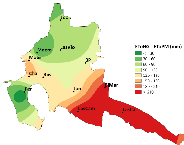
Figura 10: Diferencia en los valores de la ET_0 anual (mm) por HG y PM para el Oasis Norte de Mendoza. (Interpolación por el método "Multivariate b-spline interpolation" en QGIS)
