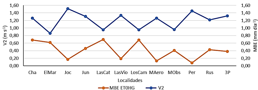
Fig 15: Relación entre la velocidad del viento a 2 m ( V_2 ) en m s -1 y el MBE de ET_0HG .
