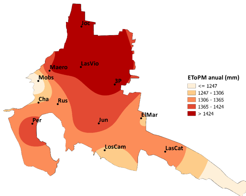
Figura 6: Valores anuales de ET_0PM ( mm\ año^{-1} ) para el Oasis Norte de Mendoza (Interpolación por el método "Multivariate b-spline interpolation" en QGIS).
