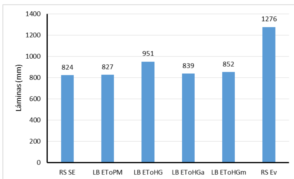
Figura 24: Comparación de las láminas de riego superficial aplicadas en ensayos experimentales sin estrés hídrico (RS SE); laminas brutas (LB) teóricas de riego según ET_0 obtenido por ET_0PM , ET_0HG , ET_0HG\alpha y ET_0HGm y lámina bruta aplicada por los productores (RS Ev).
