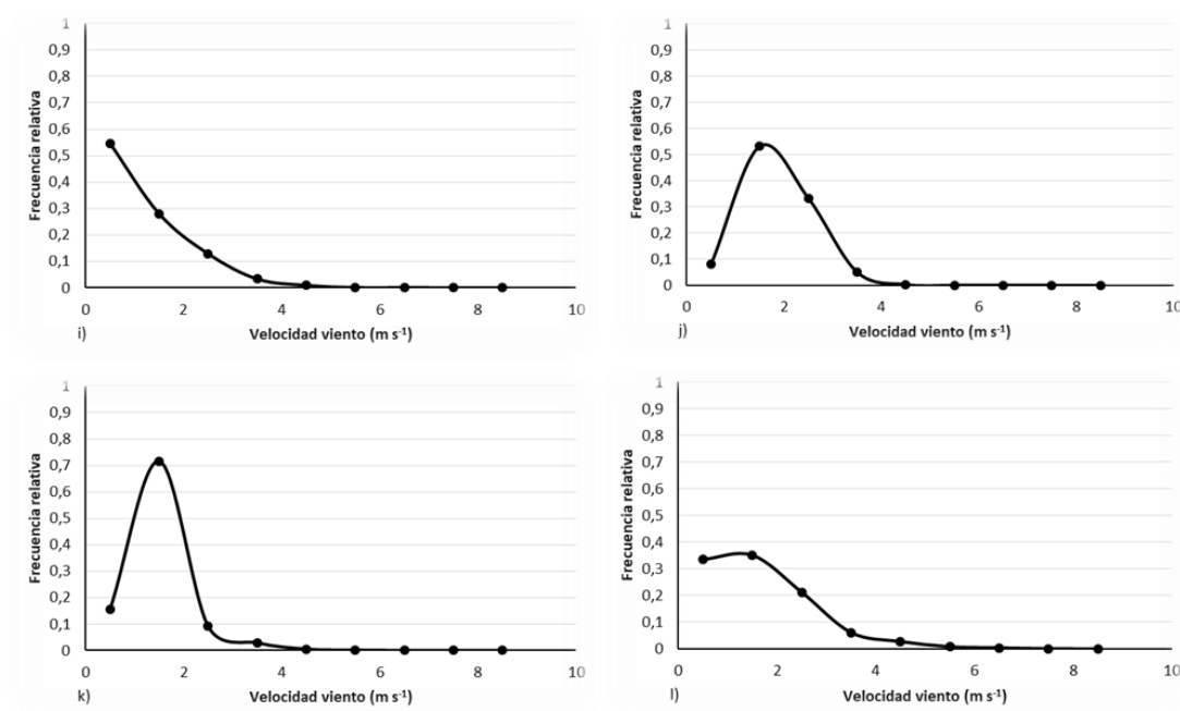
Figura 16: Curvas de distribución de frecuencia relativas de la velocidad del viento diaria ( \text{m s}^{-1} ) a 2 m de altura para el periodo de estudio en a) Cha; b) ElMar; c) Joc; d) Jun; e) LasCat; f) LasVio; g) LosCam; h) Maero; i) Mobs; j) Per; k) Rus; l) 3P.
