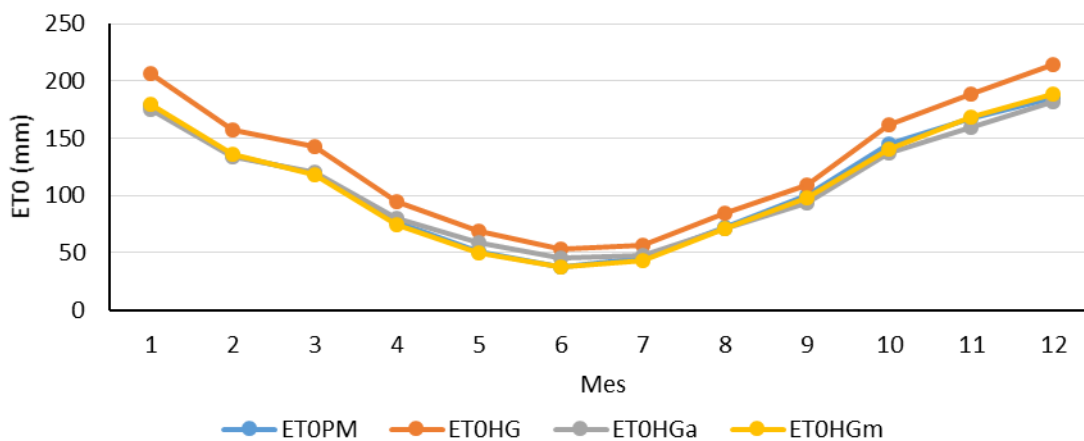
Fig. 13: Marcha de los valores mensuales de ET_0 en mm\ mes^{-1} para la estación de ElMar en el periodo de validación 2012-2014.
