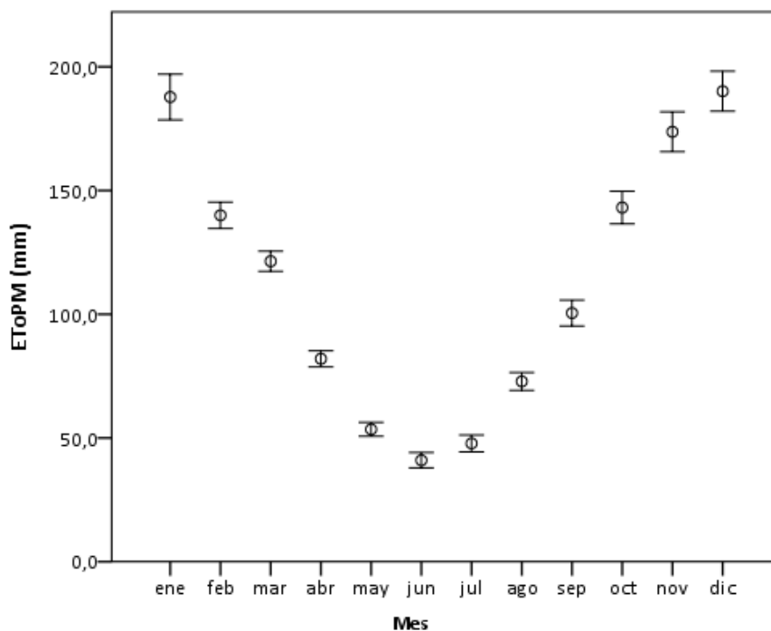
Figura 8: Valores medios mensuales de ET 0 PM para las estaciones del Oasis Norte de Mendoza, el círculo indica la media y las barras los valores extremos.
