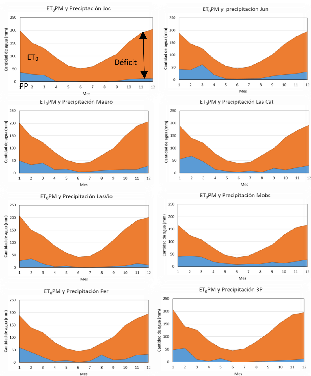
Figura 7: Marcha mensual de ET_0PM y precipitación PP (azul) mensual en milímetros para las estaciones de Joc, Jun, Maero, LasCat, LasVio, Mobs, Per y 3P. El área en color naranja indica el déficit de agua estimado entre el forzante atmosférico y la precipitación (sin tener en cuenta la cantidad de agua remanente que pueda quedar producto del riego).
