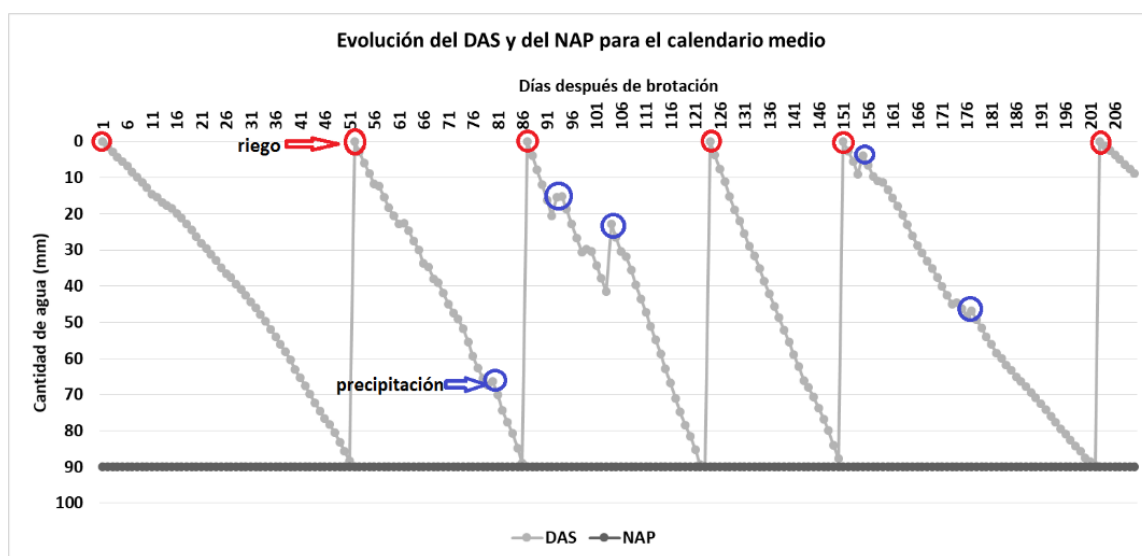
Figura 4: Evolución del déficit de agua en el suelo (DAS) y del nivel de agotamiento permisible (NAP). Se marcan en rojo los momentos de riego y en azul los eventos de precipitación.
