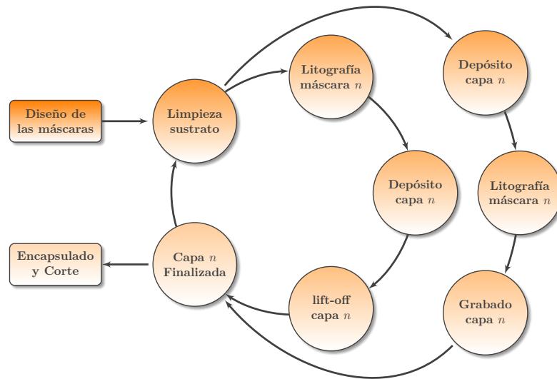
Figura 2.7: Diagrama general para la transferencia de los diseños y fabricación de una o más capas. Este esquema contempla el uso de las técnicas de lift-off o grabado según se requiera dependiendo de las características de los materiales empleados para esa capa.
