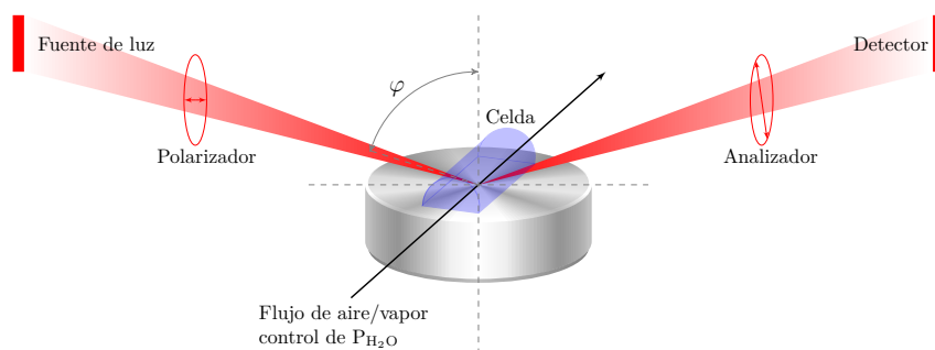
Figura 2.5: Esquema de los componentes principales del equipos de elipsometría utilizado para determinar las constantes elipsométricas, \Delta(\lambda) y \Psi(\lambda) , de las cuales se obtienen el espesor, índice de refracción, coeficiente de absorción, distribución y tamaño de poros y cuellos de las PDM.
