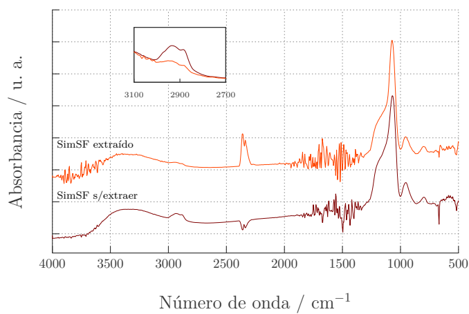
Figura A.8: Espectro de absorción en el IR para una SimSF sintetizada con el tratamiento simplificado antes y después de extraer el surfactante. Desaparece la banda de estiramiento C-H correspondiente al surfactante luego de la extracción.
