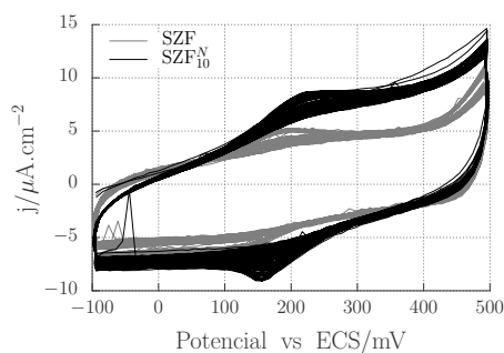
a. Respuesta utilizando como sonda negativa [\text{Fe}(\text{CN})_6]^{4-/3-} 1 mM.
