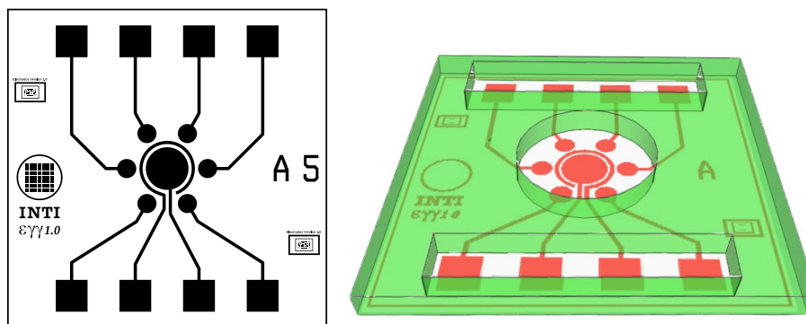
Figura 5.2: Segundo diseño de los sensores. Izquierda: Diseño de un sensor con 6 electrodos de trabajo, contraelectrodo, electrodo de referencia y marcas de alineación. Derecha: Modelo en 3D para un sensor con celda electroquímica. En rojo los electrodos y en verde la resina que forma la celda, el espesor de la misma es de aproximadamente 100\ \mu\text{m} y puede contener un volumen aproximado de 2\ \mu\text{l} .
