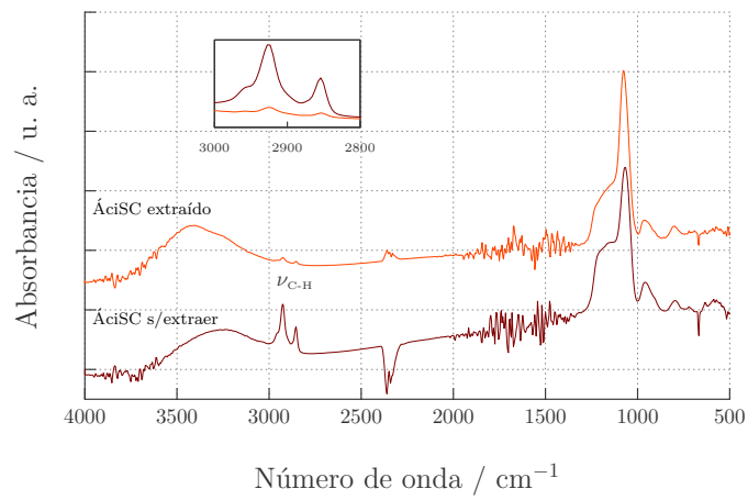
Figura A.28: Espectro de absorción en el IR para una ÁciSC antes y después de extraer el surfactante.
