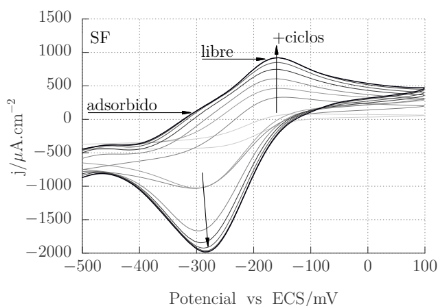
Figura 4.5: Solución de ARu 10 mM a pH = 5,5 en KCl 100 mM sobre SF. Se observa el aumento la señal a medida que la sonda ingresa en la estructura porosa. Los voltagramas fueron tomados a 50 \text{ mV s}^{-1} y el número de ciclos electroquímicos aumenta del gris claro al negro.
