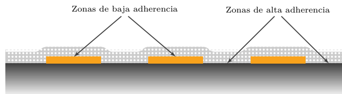
Figura 3.6: Esquema de un corte transversal de los sensores donde se observan los microelectrodos y la PDM depositada sobre ellos. Las flechas indican las zonas de baja y alta adherencia.
