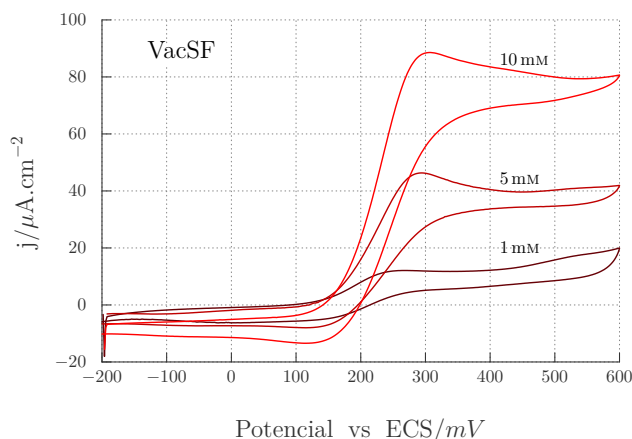
Figura 4.8: Voltagramas de SF sintetizada por el método de alto vacío para FcOH 1, 5 y 10 mM en solución de KCl 100 mM tomados a una velocidad de barrido de 20 \text{ mV s}^{-1} . Se observa que se alcanza una densidad corriente límite ( j_l ) para cada una de las concentraciones de la sonda.
