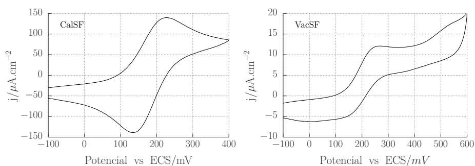
Figura 3.25: Voltamétrías para FcOH 1 mM en 100 mM de KCl realizada a 50 \text{ V s}^{-1} . Izquierda: sobre sistemas SF calcinados. Derecha: sobre sistemas SF condensados por el método de alto vacío y extraído con 2-propanol y agua acidificada.
