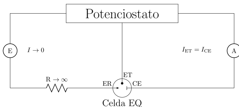
Figura 2.17: Esquema eléctrico correspondiente al armado experimental utilizado para realizar las voltametrías cíclicas.
