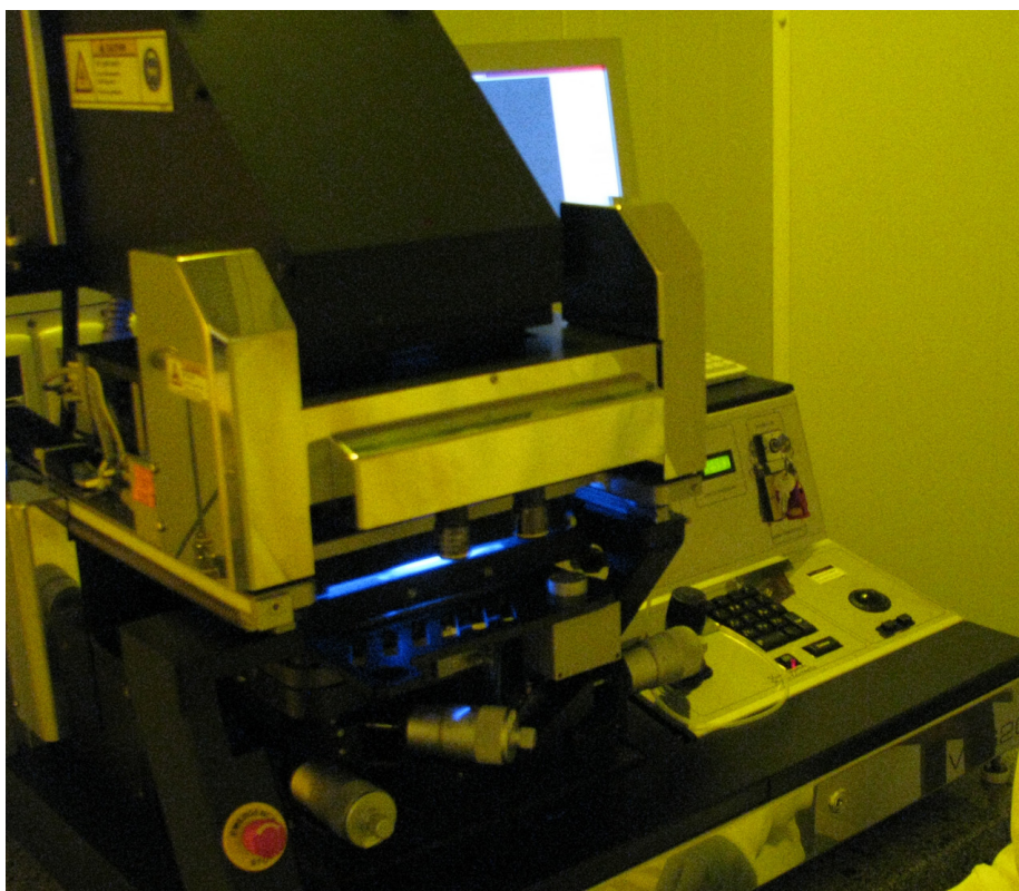
Figura 2.10: Alineadora de máscaras EVG 620 semiautomática de doble cara, con lámpara de Hg de 350 W y capacidad para obleas de hasta 150 mm .
