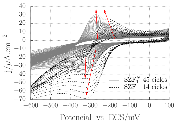
Figura 4.31: Voltagramas cíclicos de ARu sobre películas funcionalizadas con APTES (SZF 1 N ) y sin funcionalizar (SZF) donde se destaca la diferente cinética de adsorción para cada sistema.
