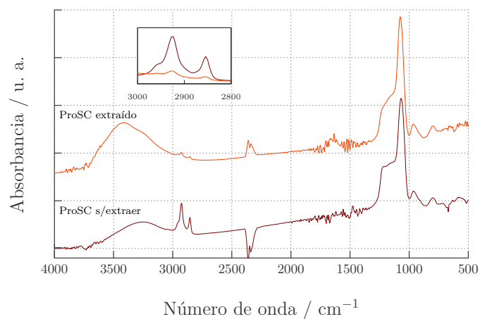
Figura A.15: Espectro de absorción de IR correspondiente a una ProSC antes y después de la extracción con 2-propanol.
