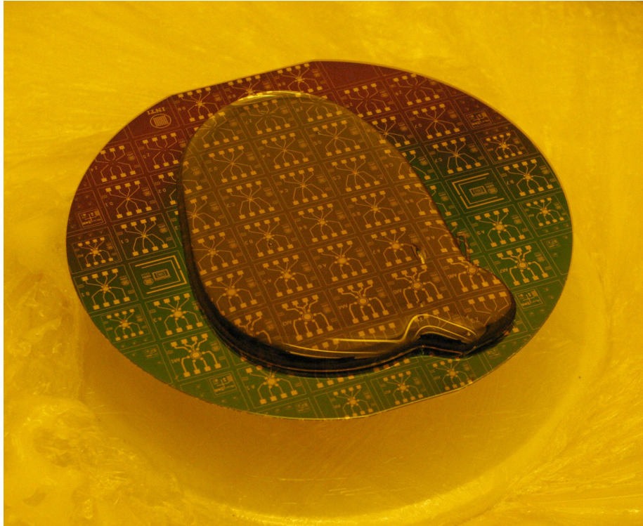
Figura 5.6: Depósito por spin-coating de la resina epoxi para encapsular los multisensores. Se destaca la alta viscosidad de la misma, lo que permite formar paredes de hasta 100 \mu\text{m} de espesor.
