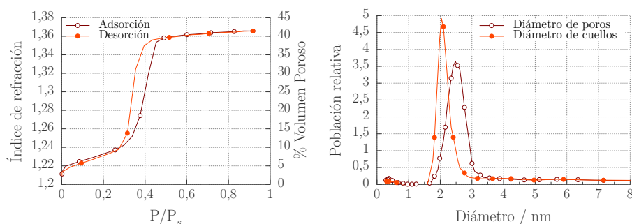
a. Elipsoporosimetría de una CalSC sobre sustrato de silicio sintetizada por el método clásico de calcinación.
