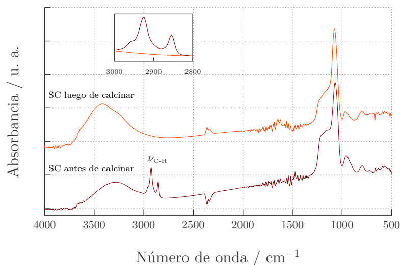
Figura 3.16: Espectro de absorción para una SC antes y después de calcinar, donde se puede apreciar la aparición de una banda fuerte ( \nu_{C-H} ), la cual correspondiente al surfactante CTAB.
