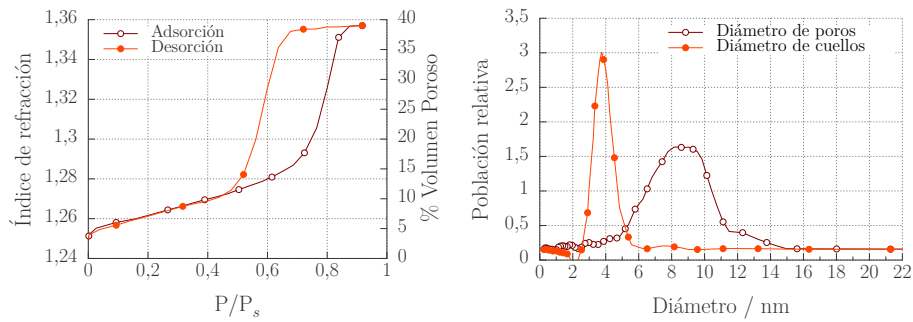
a. Elipsoporosimetría de una SF tratamiento 7 días en alto vacío. b. Distribución de tamaño de poro y cuello.
