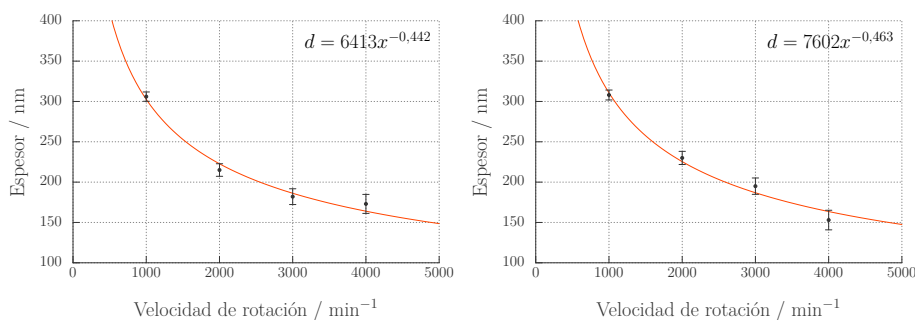
Figura 3.3: Control del espesor en función de la velocidad angular para valores comprendidos entre 1000 y 4000 \text{min}^{-1} en sistemas calcinados estructurados con F127 (izquierda) y CTAB (derecha). Todas las mediciones fueron llevadas a cabo por EPA.
