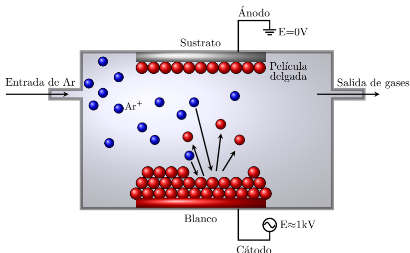
Figura 1.11: Representación esquemática del depósito de una película delgada por el proceso de pulverización catódica o sputtering .
