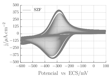
c. Respuesta sobre una SZF sin funcionalizar utilizando como sonda positiva [\text{Ru}(\text{NH}_3)_6]^{3+} 1 mM.
