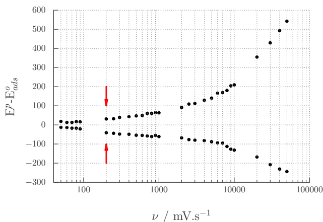
Figura 4.12: Desplazamiento de los potenciales en función de la velocidad de barrido. Las flechas rojas indican la velocidad característica para el cambio de régimen, de capa delgada a control difusional.
