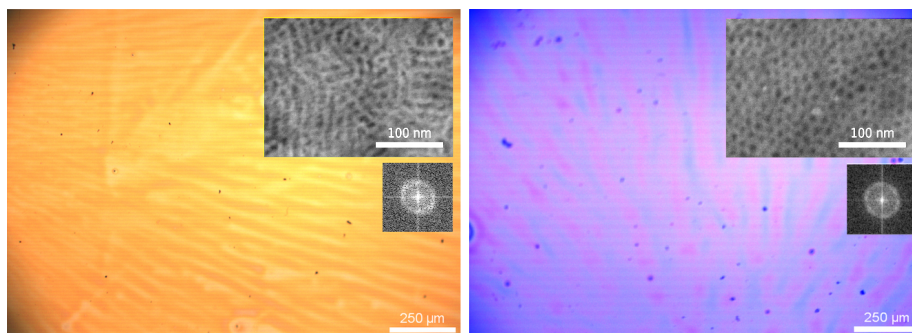
Figura A.10: Microscopías ópticas para ProSF. Izquierda: sobre sustrato de Au. Derecha: sobre sustrato de Si. En los respectivos recuadros se observa el detalle por MEB junto a la transformada de Fourier del arreglo nanoporoso.
