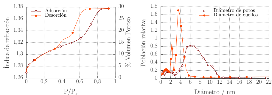
a. Isoterma de adsorción/desorción de agua realizada por PEA para una SimSF. b. Distribución de tamaño de poro y cuello.
