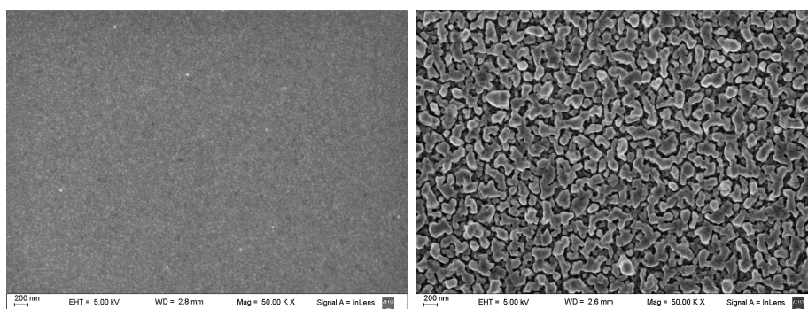
Figura 5.14: Microscopías de barrido electrónico donde se comparan los electrodos sin calcinar (izquierda) con aquellos sometidos a tratamiento térmico (derecha) . Se observa en las películas calcinadas un aumento en el tamaño de las partículas de Au.
