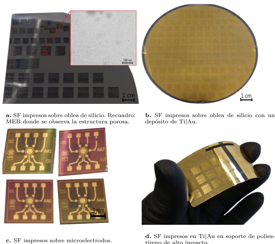
Figura 6.2: Fotografías de películas mesoporosas de \text{SiO}_2 impresas por inyección de tinta a partir de soles modificados y diseños arbitrarios. Los poros fueron moldeados con F127 y la condensación se realizó por el método de alto vacío. La extracción se llevó a cabo con 2-propanol y agua a \text{pH}=2 .
