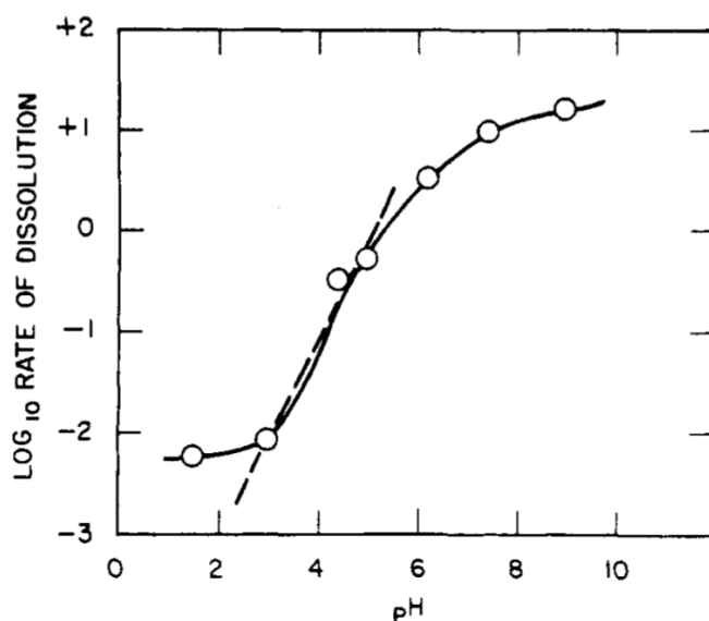
Figura 4.2: Velocidad de disolución de la sílice en función de pH. Gráfico extraído de The chemistry of silica Wiley 1ª edición, 1979. 224
