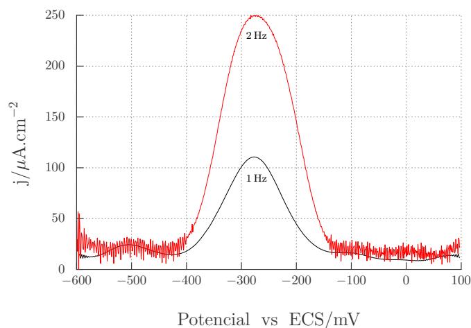
Figura 4.14: Voltametría de corriente alterna para una película saturada con ARu. Se aplicó una perturbación de 10 mV y una frecuencia de 1 y 2 Hz en solución de KCl 100 mM usando como referencia ECS.
