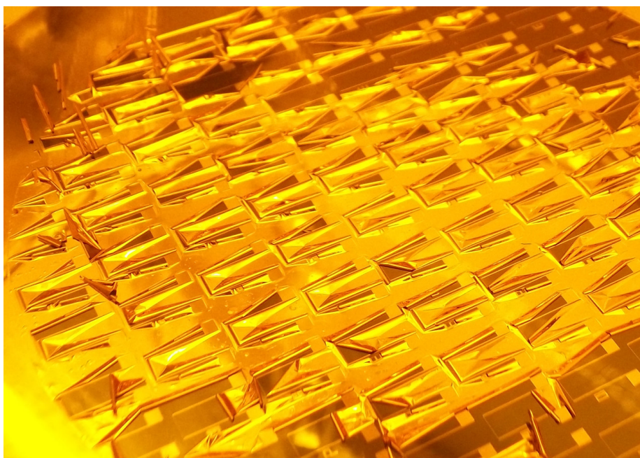
Figura 5.10: Proceso de decapado o lift-off . Fotografía correspondiente a los electrodos del primer diseño, donde se muestra como a medida que se disuelve la fotorresina se va levantando el metal que está sobre ella.
