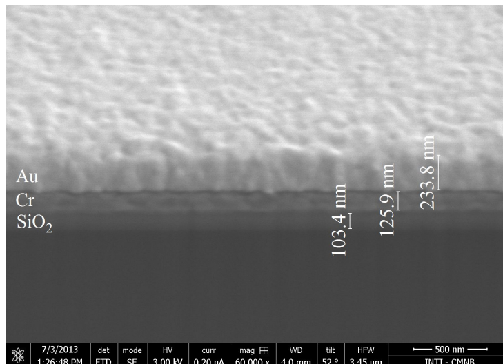
Figura 5.8: Corte transversal de los electrodos, donde se observan detalles de la bicapa Cr|Au depositada sobre una oblea de silicio con un depósito aislante de SiO 2 .
