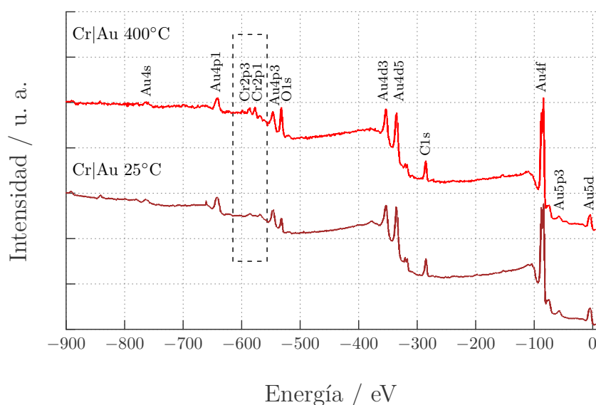
Figura 5.15: Espectroscopía de fotoelectrones emitidos por rayos (XPS) correspondiente a películas delgadas de Cr|Au con y sin tratamiento térmico. Obsérvese los picos correspondiente al cromo y el aumento de la intensidad relativa del pico correspondiente al oxígeno, sugiriendo la difusión de Cr_xO_y hacia la superficie de los electrodos.
