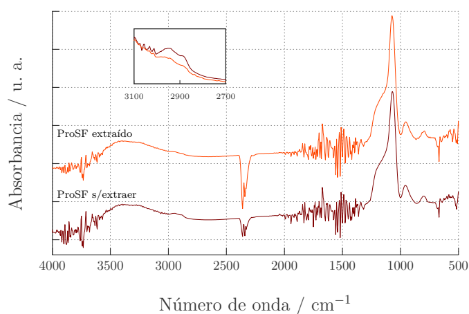
Figura A.14: Espectro de absorción de IR correspondiente a una ProSF antes y después de la extracción con 2-propanol.
