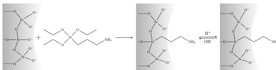
Figura 4.28: Esquema donde se representa la reacción de APTES con SZF para obtener películas funcionalizadas con grupos aminos y la dependencia de la carga con el pH. Figura adaptada de Films delgados mesoporosos híbridos conteniendo el grupo amino: una plataforma para el diseño y producción de membranas permeoselectivas , Calvo A., Tesis de Doctorado, Instituto de investigación e ingeniería ambiental - UNSAM, 2010. 103
