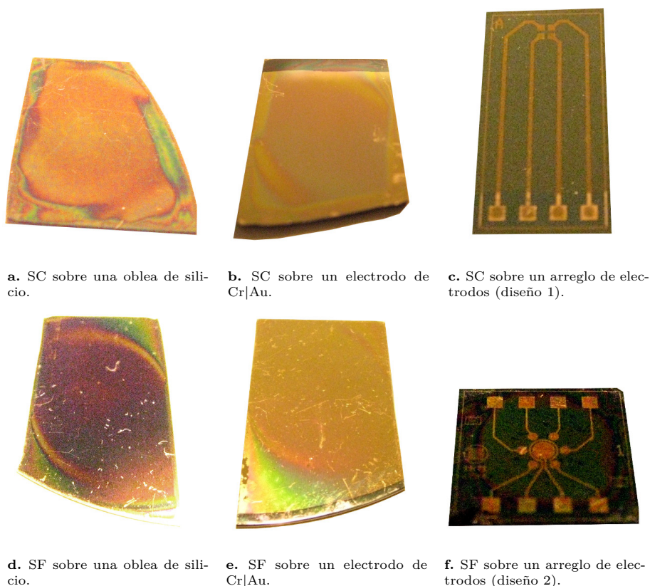
Figura 3.1: Fotografías de las PDM obtenidas por spin-coating sobre distintos sustratos para los surfactantes F127 y CTAB.
