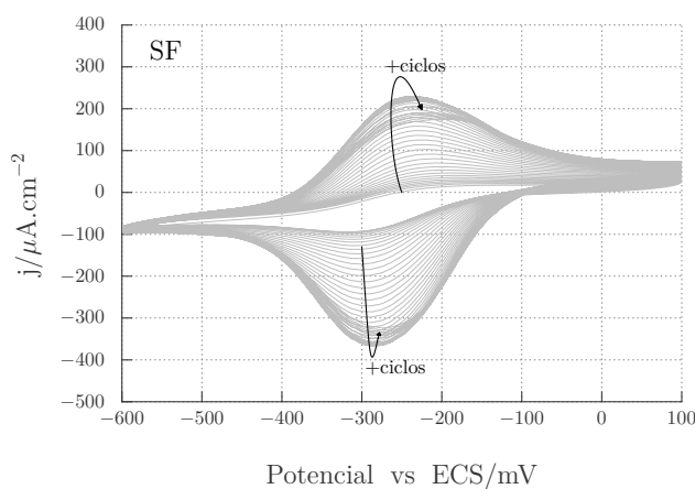
Figura 3.8: Voltametrías cíclicas consecutivas para [\text{Ru}(\text{NH}_3)_6]^{3+} 1 mM a partir del ciclo número 44 realizados a 50 \text{ mV s}^{-1} sobre electrodos modificados con MPTMS. La respuesta es de características similares a la obtenida para este tipo de sistemas, donde se observa el ingreso de la sonda, la adsorción y la disminución de la intensidad debido a un fenómeno de disolución. No se observa indicio alguno de falta de adherencia.
