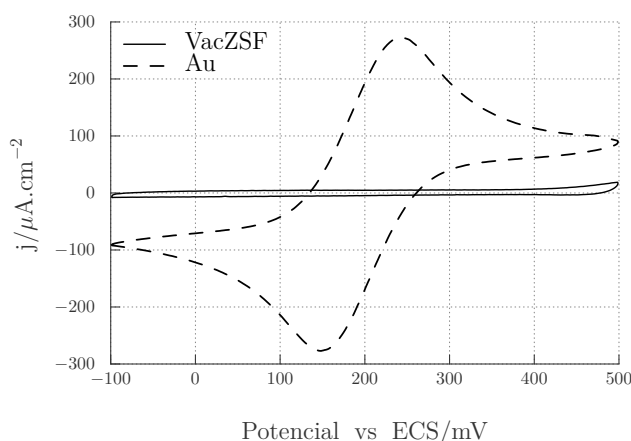
Figura 4.22: Respuesta comparativa de un electrodo de Au recubierto con SZF (sólida) y uno sin recubrir (punteado) frente a una sonda [\text{Fe}(\text{CN})_6]^{4- / 3-} 1 mM en 0,1 M de KCl utilizando ECS como referencia.
