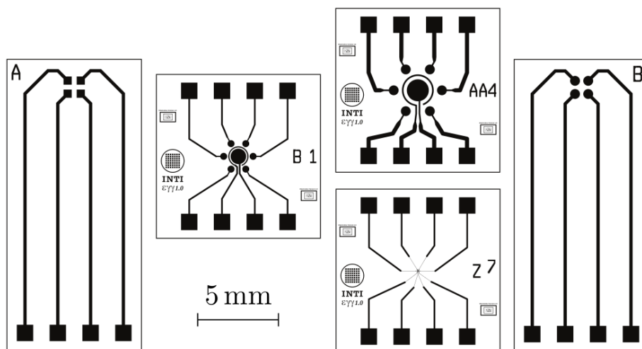
Figura 2.8: Algunos ejemplos de los diseños de los multisensores que se utilizaron a lo largo de este trabajo de tesis. Cada diseño corresponde a un dispositivo que forma parte de un lote de fabricación de al menos 40 unidades.
