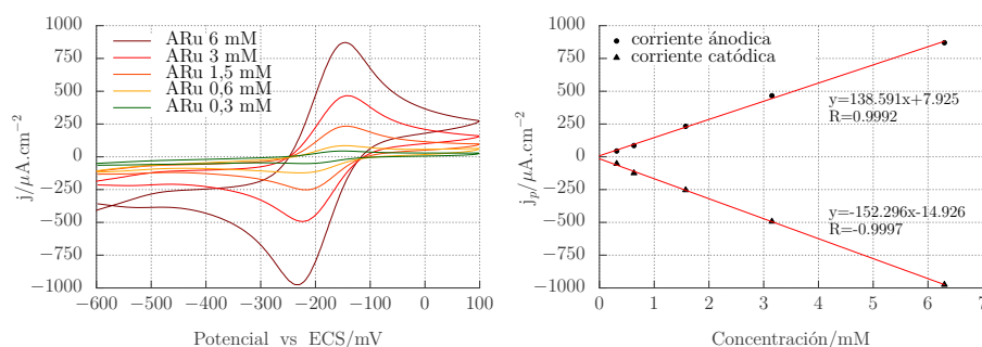
a. Voltametrías cíclicas para ARu a diferentes concentraciones.
