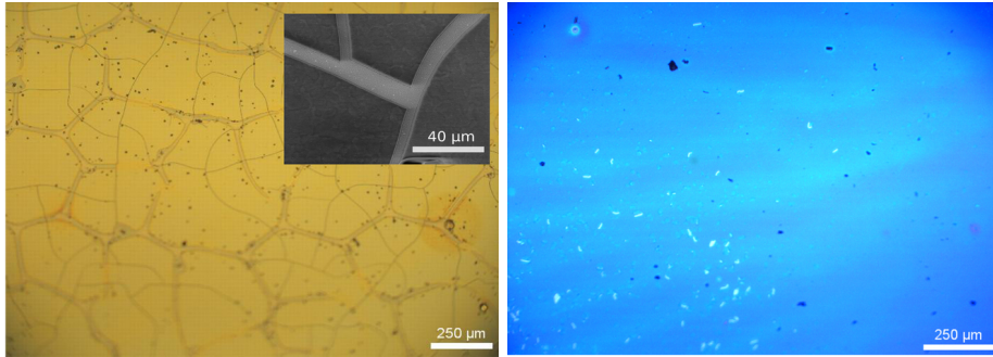
Figura A.30: Microscopías ópticas para AlcSC sintetizadas por el tratamiento de condensación y extracción en medio alcalino. Izquierda: sobre sustrato de Au. Derecha: sobre sustrato de Si.
