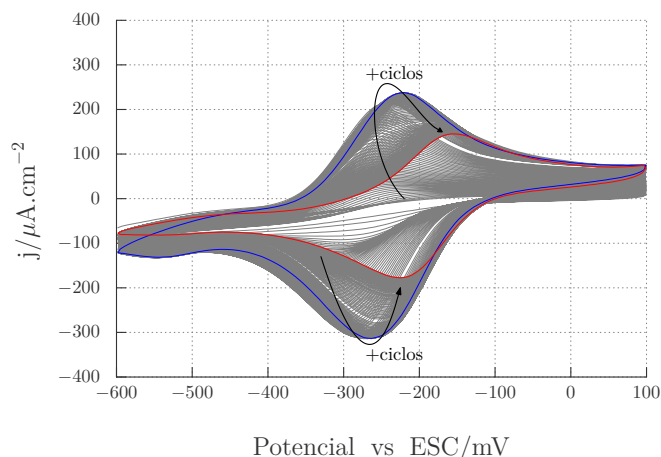
Figura 4.20: Ciclos sucesivos de VCs para ARu 1 mM en solución de KCl 100 mM. Se observa aquí como se carga para luego recuperar la señal de un electrodo de Au desnudo, debido a la disolución de la SF.
