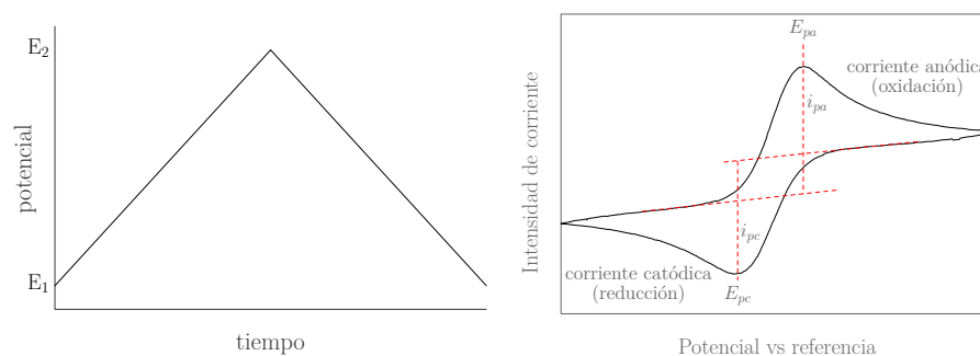
Figura 2.18: Curva de excitación y voltograma típico para una especie rédox reversible. Se destaca en el voltograma (derecha) los típicos parámetros que se extraen de la curva, picos máximos de corriente anódica y catódica sus correspondientes potenciales.
