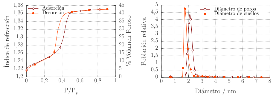
a. Elipsoporsimetría de una SC Tratamiento 7 días alto vacío. b. Distribución de tamaño de poro y cuello.
