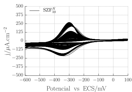
d. Respuesta sobre una SZF funcionalizada con APTES 10 mM utilizando como sonda positiva [\text{Ru}(\text{NH}_3)_6]^{3+} 1 mM.
