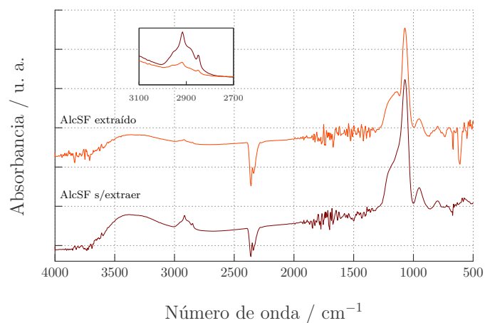
Figura A.33: Espectro de absorción en el IR para una AlcSF antes y después de extraer el surfactante. Obsérvese la ausencia de hombro en la región 1250-1100 cm -1 , el cual es típico en sistemas de SiO 2 mesoestructuras.
