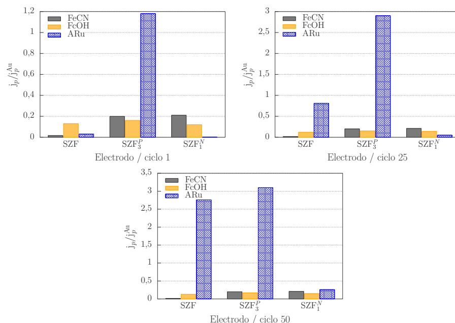
Figura 5.20: Densidad de corriente anódica máxima en los ciclos 1, 25 y 50 para cada uno de los electrodos del sensor. Las sondas probadas fueron FeOH 1 mM, FeCN 1 mM y ARu 1 mM en KCl 100 mM a una velocidad de barrido de 50 \text{ mV s}^{-1} .
