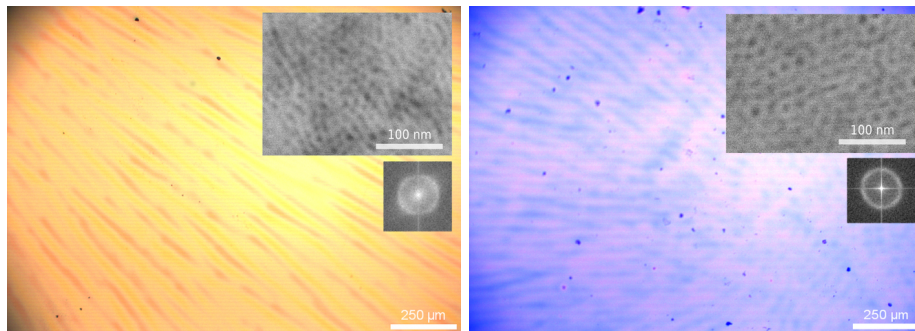
Figura A.4: Microscopías ópticas para SimSF. Izquierda: sobre sustrato de Au. Derecha: sobre sustrato de Si. En los respectivos recuadros se observa el detalle por MEB junto a la transformada de Fourier del arreglo nanoporoso.
