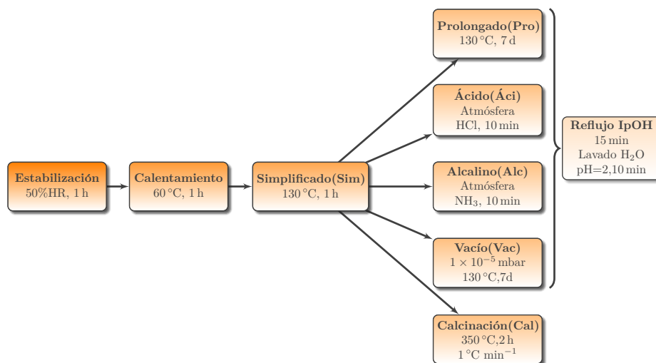
Figura 2.4: Etapas de estabilización y diferentes tratamientos posdeposición utilizados para condensar y extraer el surfactante en las PDM, tanto de óxidos puros como mixtos.
