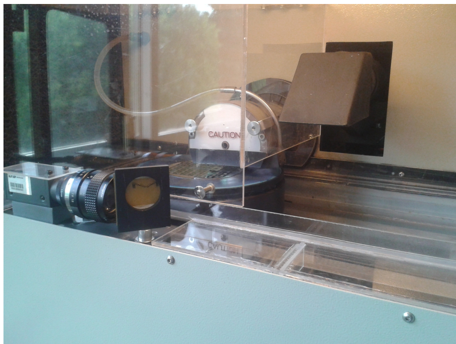
Figura 2.14: Cortadora de obleas de la marca Laser Optics , ubicada en los laboratorios del INTI-CMNB
