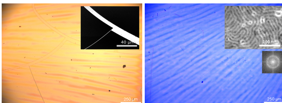
Figura A.23: Microscopías ópticas para ÁciSF. Izquierda: sobre sustrato de Au. Derecha: sobre sustrato de Si. En los respectivos recuadros se observa el detalle por MEB junto a la transformada de Fourier (sobre silicio) del arreglo nanoporoso.
