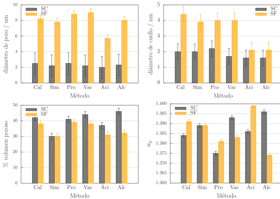
Figura 3.22: Comparación de las magnitudes más relevante (diámetro de poros, diámetro de cuellos, % volumen poroso e índice de refracción de la pared inorgánica), extraídas del análisis por EPA, con el ánimo de comparar el grado de condensación de las películas delgadas mesoporosas en base sílice, estructuradas con F127 (SF) y CTAB (SC).
