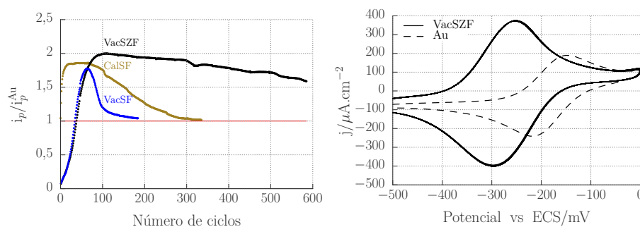
a. Comparación de la razón de la intensidad de pico de ARu 1 mM para CalSF, VacSF y VacSZF respecto de un electrodo de Au.
