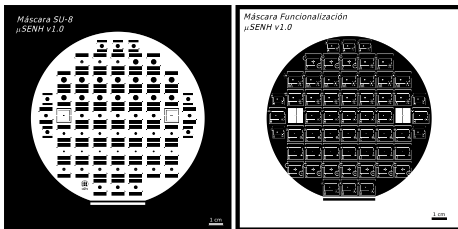
c. Máscara para depositar la fotorresina epoxi que dará lugar a la celda electroquímica.
