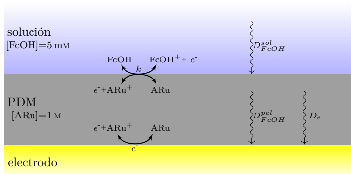
Figura 2.20: Esquema del modelo utilizado para las simulaciones por el MEF y las variables que se emplearon para evaluar fenómenos de transporte y mediación redox.
