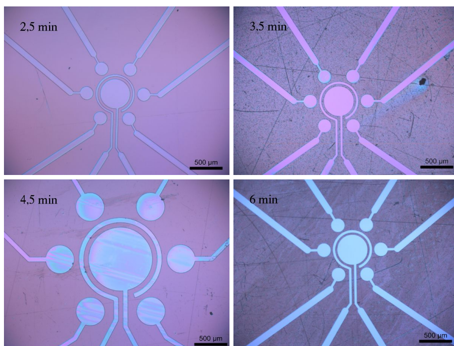
Figura 5.5: Tiempos crecientes de revelado: 2,5 min, 3,5 min, 4,5 min y 6 min). Se aprecia como se disuelve la resina en la solución reveladora indicado por el cambio de color a medida que disminuye el espesor. Se muestra en la última microscopía el revelado completo con un 20 % de tiempo adicional para crear el perfil negativo de las paredes, necesario para el proceso de lift-off .
