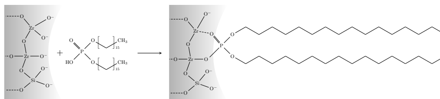
Figura 4.26: Esquema donde se representa la reacción de DHDP con SZF para obtener películas funcionalizadas con DHDP. Figura adaptada de Films delgados mesoporosos de óxidos metálicos, mixtos e híbridos. Hacia un diseño racional de nanomateriales funcionales . Angelomé P., Tesis de Doctorado, Facultad de Ciencias Exactas y Naturales - UBA, 2008. 32
