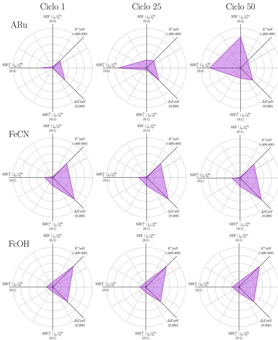
Figura 5.21: Marcas sensoriales para ARu, FeCN y FcOH para los ciclos electroquímicos 1, 25 y 50. Cabe destacar que para las sondas neutra y negativa (FcOH y FeCN) la marca permanece constante a lo largo de los ciclos. Para la sonda positiva (ARu) la marca va mudando en función de las propiedades permeoselectivas de cada electrodo del multisensor. Notar el cambio de escala para ARu en los electrodos SZF y SZF_3^P debido a la alta capacidad preconcentradora de estas películas para la sonda de carga positiva.
