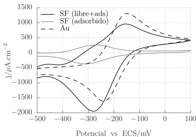
Figura 4.6: Voltagramas donde se compara la señal para ARu 10 mM a pH = 5,5 en KCl 100 mM en un electrodo de Au (- -), en una SF (—) y en una SF luego de retirar la solución de ARu(—).
