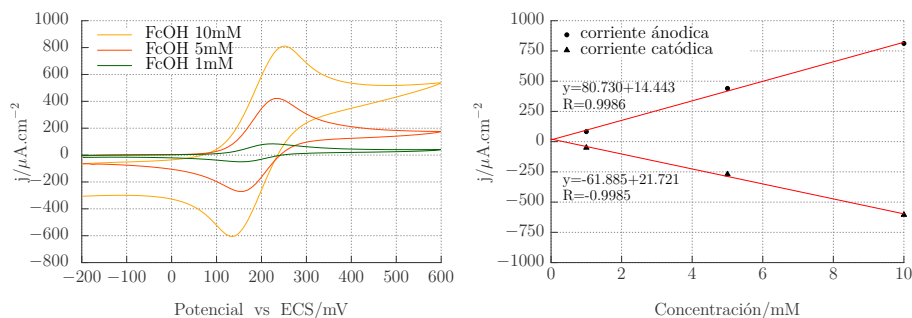
a. Voltametrías cíclicas para FcOH a diferentes concentraciones, 1 mM, 5 mM y 10 mM.
