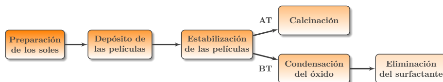
Figura 2.1: Diagrama de flujo para las dos rutas sintéticas utilizadas en la síntesis de películas delgadas mesoporosas: alta temperatura (AT, 350 °C) y baja temperatura (BT, 130 °C).
