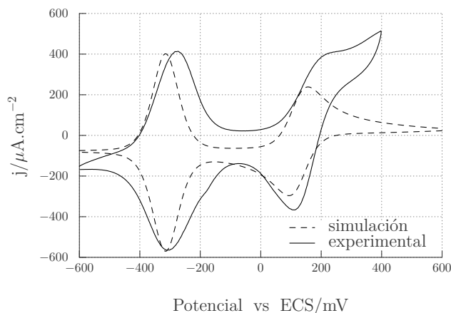
Figura 4.18: Comparación entre resultados experimentales y de simulación. Los parámetros de la simulación fueron k = 1000 \text{ M}^{-1} \text{ s}^{-1} , D_{Fc} = 10^{-6} \text{ cm}^2 \text{ s}^{-1} con FcOH 5 mM en un PDM con ARu adsorbido 1 M. El experimento de laboratorio fue realizado con las mismas concentraciones para ambas sondas.
