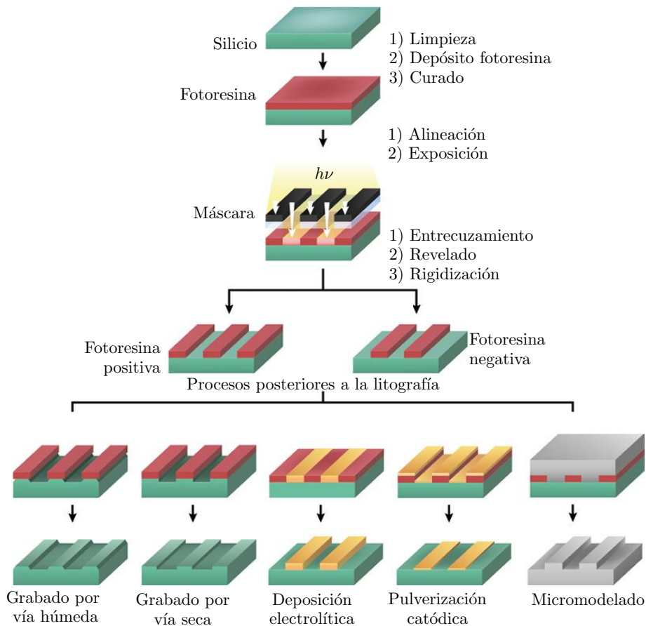
Figura 1.10: Etapas involucradas en un típico proceso fotolitográfico y algunas de sus posibles aplicaciones en la transferencia de los diseños.
