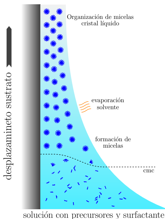
Figura 1.9: Proceso de autoensamblado inducido por evaporación (AEIE) mediante dip-coating . La evaporación del solvente favorece la formación de micelas más allá de la cmc formado el cristal líquido. Un proceso similar ocurre cuando se aplica la técnica de spin-coating . Adaptado de «Films delgados mesoporosos de óxidos metálicos, mixtos e híbridos. Hacia un diseño racional de nanomateriales funcionales». 32
