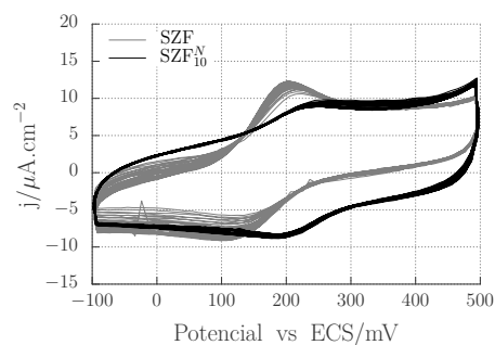
b. Respuesta utilizando como sonda neutra \text{FeOH} 1 mM.
