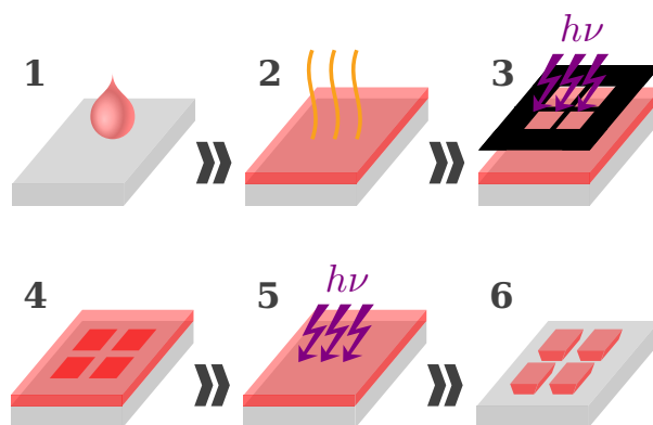
Figura 2.9: Proceso de fotolitografía para una resina de doble exposición. 1) Depósito de la resina, 2) calentamiento suave, mejora la adherencia y evapora solventes, 3) 1 a exposición, 4) calentamiento para invertir la polaridad de la resina, 5) 2 a exposición sin máscara, 6) revelado, nótese el perfil invertido, especialmente útil para aplicar en procesos de lift-off .
