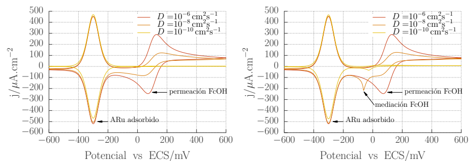
a. Simulación de mediación y permeación con k = 0 \text{ M}^{-1} \text{ s}^{-1} .
