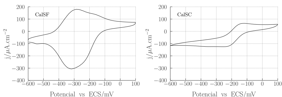
a. Voltametría Cíclica sobre CalSF.
