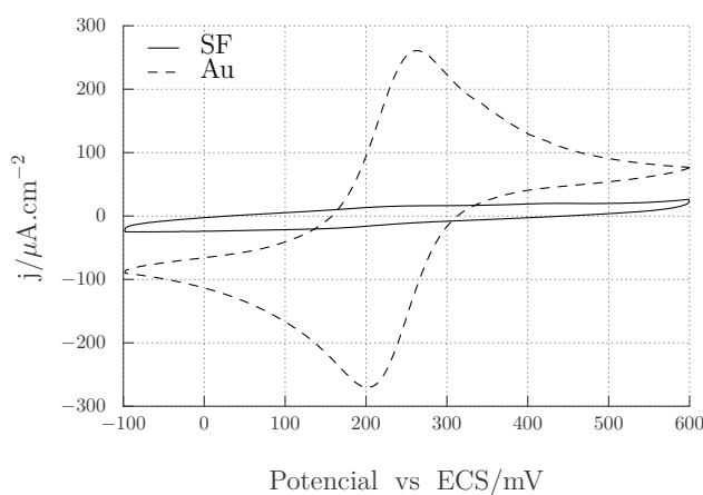
Figura 4.3: Respuesta comparativa de un electrodo de Au recubierto con SF y sin recubrir frente a una sonda FeCN 1 mM en 0,1 M de KCl a 50 \text{ mVs}^{-1} y utilizando un ECS como referencia.
