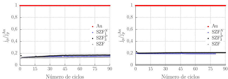
Figura 5.18: Corriente de pico anódico normalizada para FcOH 1 mM (izquierda) y FeCN 1 mM (derecha) en función de la cantidad de ciclos. Los datos fueron tomados a una velocidad de barrido de 50 \text{ mV s}^{-1} en solución de KCl 100 mM en un multisensor compuesto por cuatro electrodos diferentes: de Au (Au), recubierto con una película mesoporosa sin funcionalizar (SZF), con una funcionalizada con DHDP ( \text{SZF}_3^P ) y con una funcionalizada con APTES ( \text{SZF}_1^N ).
