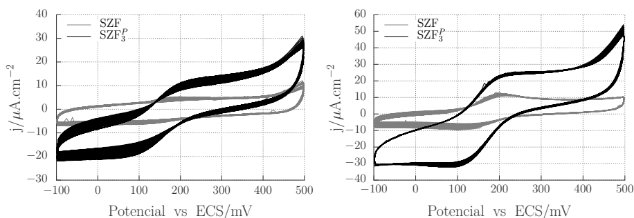
a. Respuesta utilizando como sonda negativa [\text{Fe}(\text{CN})_6]^{4-/3-} 1 mM.
