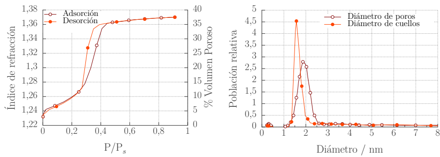
a. Isoterma de adsorción/desorción de agua realizada por PEA para una ÁciSC. b. Distribución de tamaño de poro y cuello.
