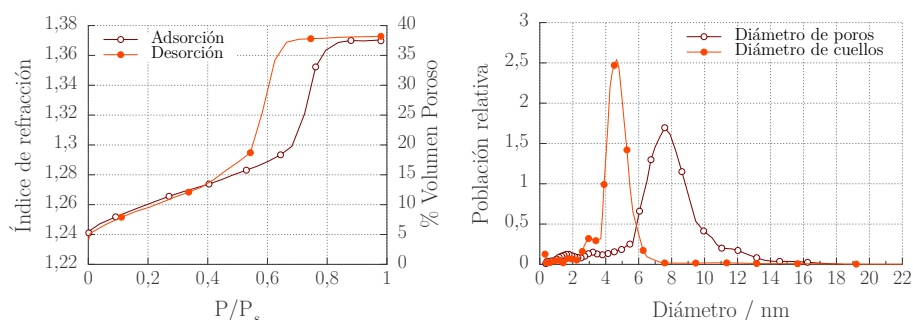
a. Elipsoporosimetría de una CalSF depositada sobre silicio sintetizada por calcinación.
