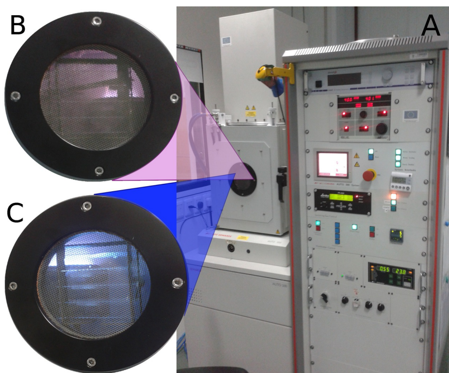
Figura 2.11: Foto del instrumental utilizado para realizar los depósitos bicapa Ti|Au o Cr|Au. (A) El equipo BOC Edwards completo donde se ve el gabinete de control y la cámara de vacío, (B) foto a través de la ventana al momento de realizar un depósito de Cr y (C) foto a través de la ventana al momento de realizar un depósito de Au.
