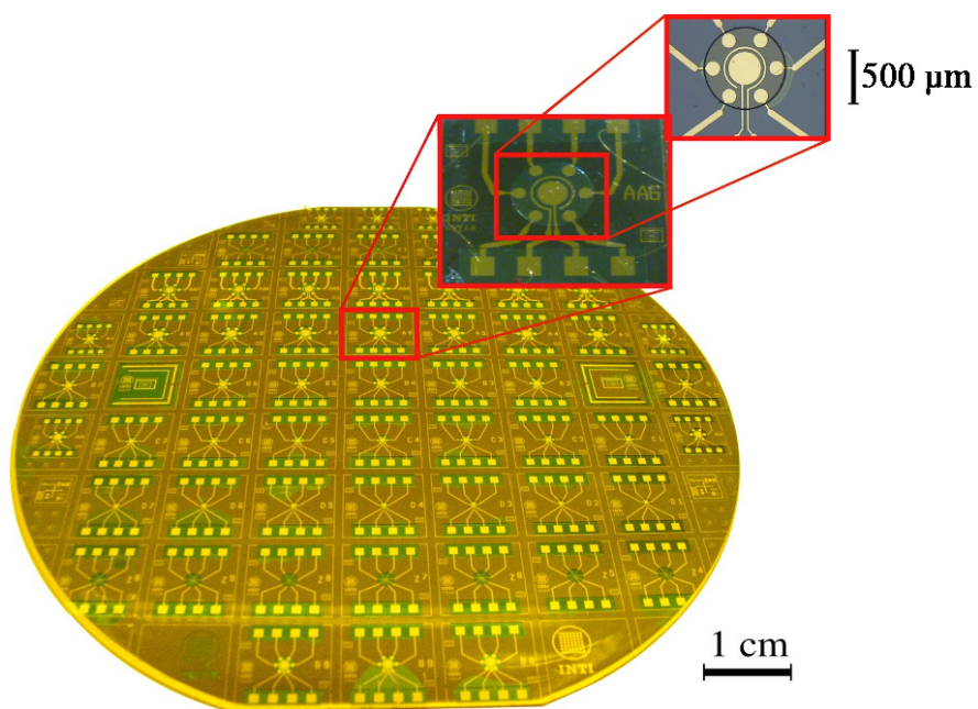
Figura 5.12: Segundo diseño de los sensores. Oblea de silicio de 10 cm de diámetro con 46 sensores con 6 electrodos de trabajo, contraelectrodo y pseudoreferencia. También se muestra la celda electroquímica depositada con resina epoxi SU-8.
