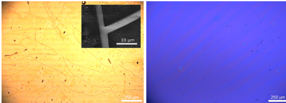
Figura A.24: Microscopías ópticas para ÁciSC. Izquierda: sobre sustrato de Au. Derecha: sobre sustrato de Si.
