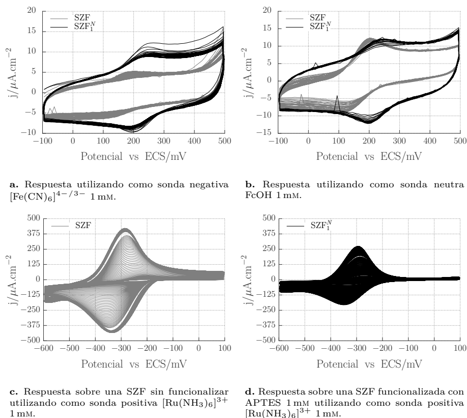
Figura 4.29: Respuesta comparativa entre SZF funcionalizadas con APTES 1 mM y sin funcionalizar en KCl 100 mM a 50 \text{ mV s}^{-1} . Para cada experimento se tomaron más de 90 voltogramas consecutivos.
