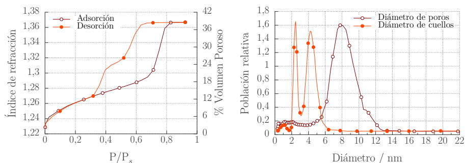
a. Isotherma de adsorción/desorción de agua realizada por PEA para ProSF. b. Distribución de tamaño de poro y cuello.
