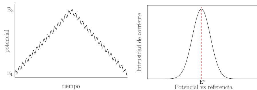
Figura 2.19: Curva de excitación utilizada en un voltametría de corriente alterna y el típico voltograma que se obtiene para una especie rédox reversible.
