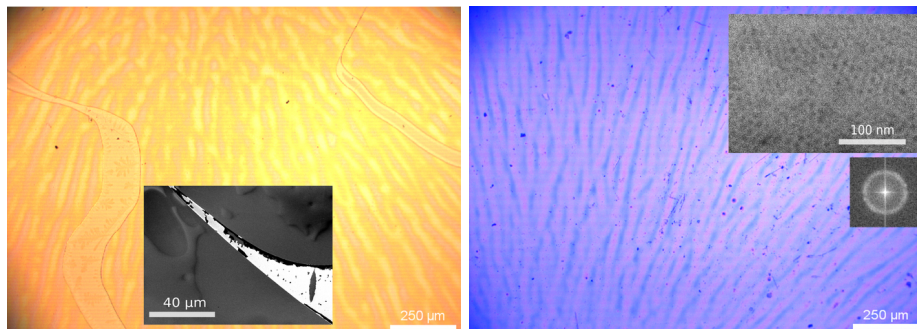
Figura A.29: Microscopías ópticas para AlcSF. Izquierda: sobre sustrato de Au. Derecha: sobre sustrato de Si. En los respectivos recuadros se observa el detalle por MEB junto a la transformada de Fourier (sobre silicio) del arreglo nanoporoso.
