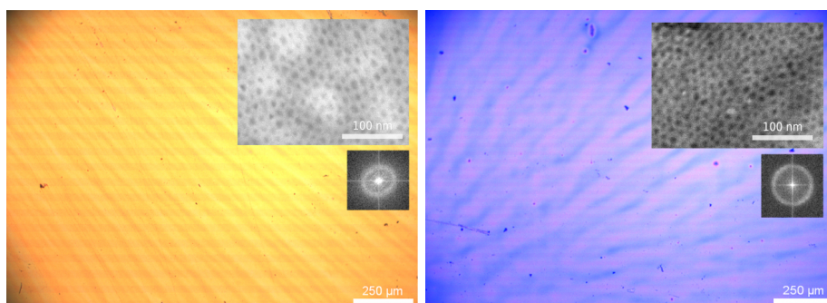
Figura A.16: Microscopías ópticas para VacSF. Izquierda: sobre sustrato de Au. Derecha: sobre sustrato de Si. En los respectivos recuadros se observa el detalle por MEB junto a la transformada de Fourier del arreglo nanoporoso.
