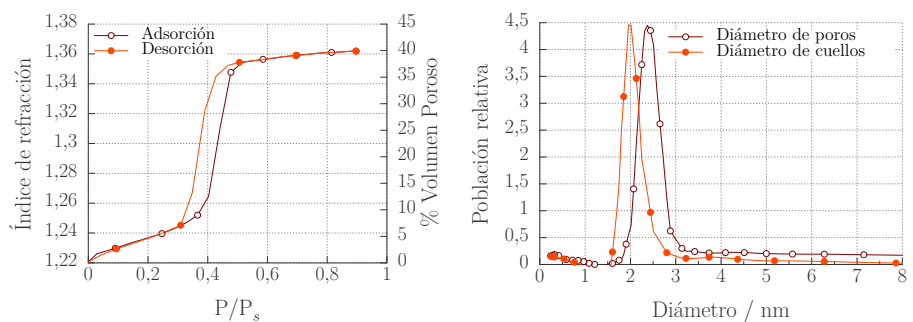
a. Isotherma de adsorción/desorción de agua realizada por PEA para ProSC . b. Distribución de tamaño de poro y cuello.
