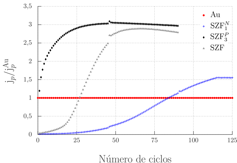
Figura 5.19: Corriente de pico anódico para ARu 1 mM en función de la cantidad de ciclos. Los datos fueron tomados a una velocidad de barrido de 50 \text{ mV s}^{-1} en solución de KCl 100 mM en un sensor compuesto por cuatro electrodos diferentes: de Au (Au), recubierto con una película mesoporosa sin funcionalizar (SZF), con una funcionalizada con DHDP ( \text{SZF}_3^P ) y con una funcionalizada con APTES ( \text{SZF}_1^N ).
