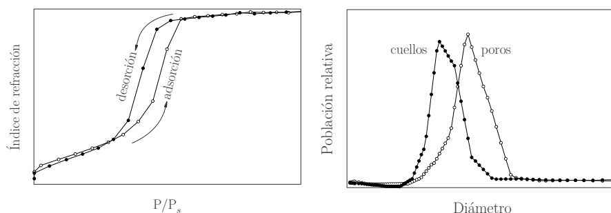
Figura 2.6: (a) Isotherma de adsorción/desorción de agua para un sistema mesoporoso de SiO 2 estructurado con CTAB. La misma se clasifica según la IUPAC como tipo IVa con ciclo de histéresis H2b; (b) Distribución de tamaño de poro y cuello.
