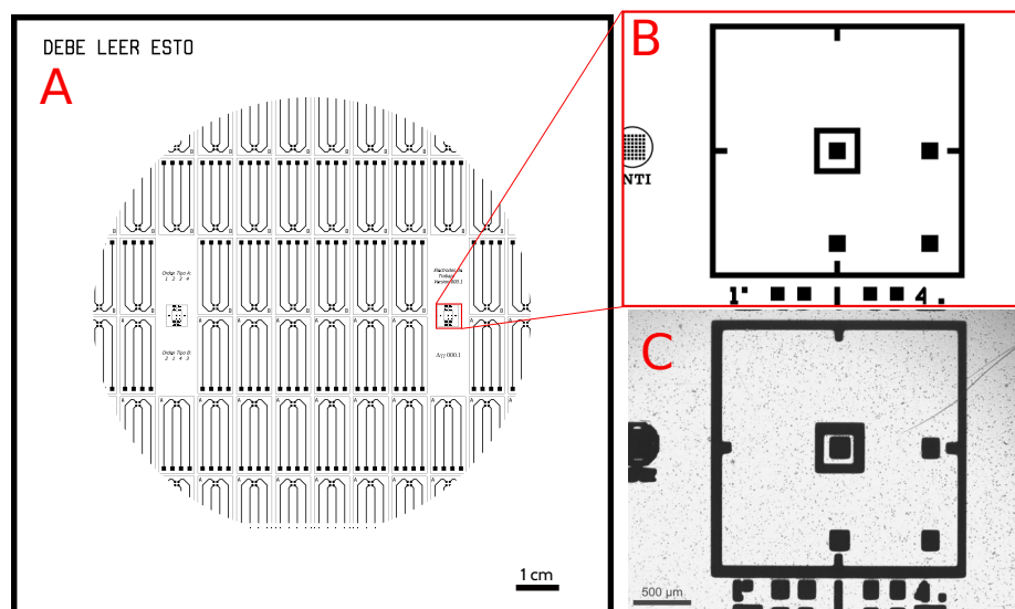
Figura 5.1: Diseño y máscara para la primera versión de los electrodos. (A) diseño completo con 32 sensores de 4 ET cada uno, (B) Detalles de las marcas de alineación empleadas, (C) microscopía óptica de la máscara donde se ven las imperfecciones de la impresión.
