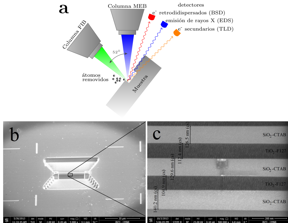
Figura 2.16: (a) Esquema donde se muestra la disposición de las columnas de electrones y de átomos de galio del Helios NanoLab 650 y los principales eventos que ocurren al impactar los haces sobre la muestra. (b) Corte en sección transversal de un dispositivo mesoporoso multicapa. (c) Imagen de alta resolución de la sección transversal enmarcada en (b).
