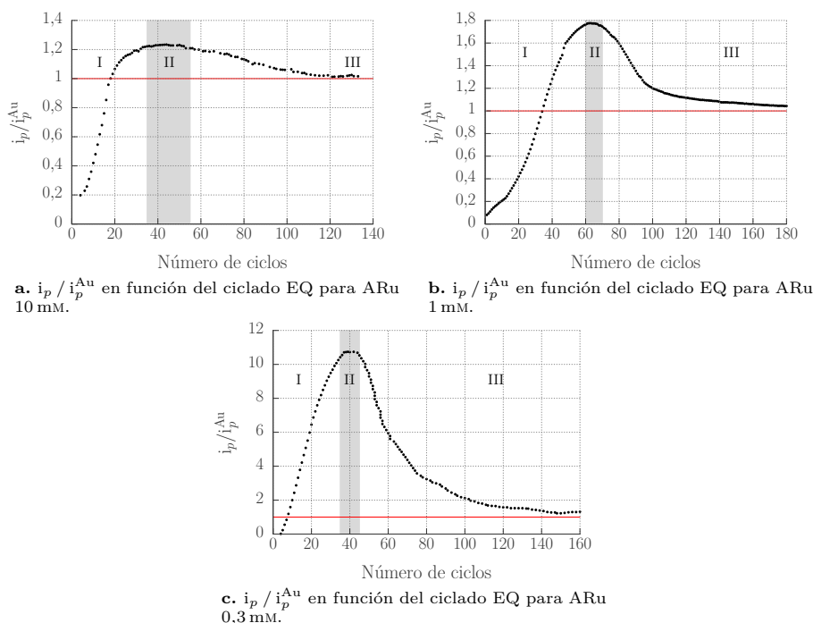
Figura 4.21: Razón entre la intensidad de pico catódica para ARu de un electrodo recubierto con PDM y uno sin recubrir, la línea roja indica cuando i_p / i_p^{\text{Au}} = 1 . Cabe destacar que al disminuir la concentración de ARu en solución aumenta el poder preconcentrador. Zona I: adsorción, zona II: máxima preconcentración, zona III: disolución.
