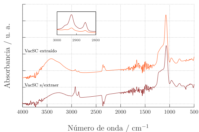
Figura A.22: Espectro de absorción de IR correspondiente a una VacSC, antes y después de la extracción con 2-propanol.
