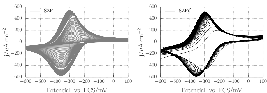
c. Respuesta sobre una SZF sin funcionalizar utilizando como sonda positiva [\text{Ru}(\text{NH}_3)_6]^{3+} 1 mM.
