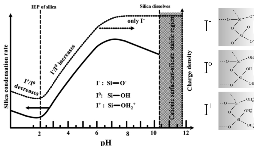
Figura 4.1: Velocidad de condensación y estado de carga superficial para nanopartículas de sílice en función de \text{pH} . Gráfico extraído de Synthesis of mesoporous silica nanoparticles Chem. Soc. Rev., 42(9):3862, 2013. 223
