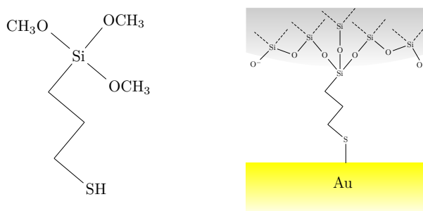
Figura 3.7: Izquierda: Molécula de 3-mercaptopropil trimetoxisilano utilizada como ligante entre los electrodos y las PDM. Derecha: esquema pictórico de la modificación superficial con MPTMS sobre los electrodos como anclaje de las PDM.
