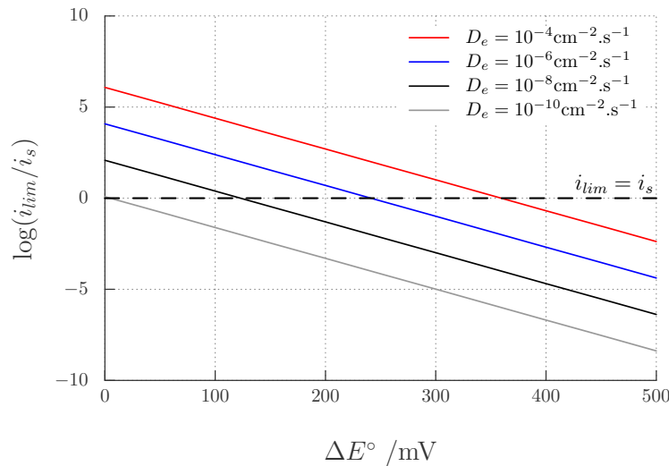
Figura 4.19: Dependencia de la relación i_{lim}/i_s variando el coeficiente de difusión dentro de la película D_e en función de la separación entre potenciales formales para el mediador y la sonda para una película de 200 nm de espesor.
