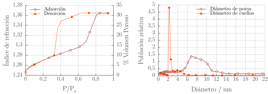
a. Isoterma de adsorción/desorción de agua realizada por PEA para una SF. b. Distribución de tamaño de poro y cuello.
