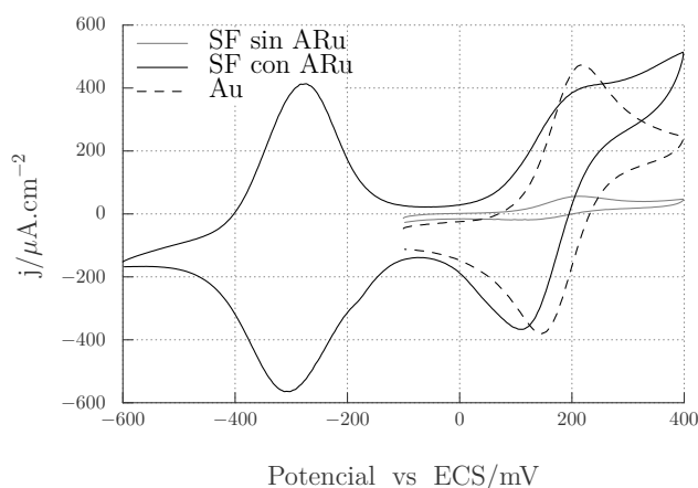
Figura 4.15: Mediciones electroquímicas de \text{FcOH} 5 mM en solución de \text{KCl} 100 mM sobre un electrodo de \text{Au} desnudo (---), sobre una SF (—) y sobre una SF con \text{ARu} adsorbido (—).
