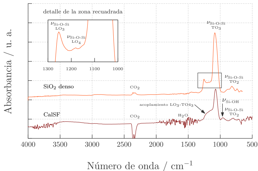
Figura 3.14: Espectro de absorción de IR de una película SiO_2 denso depositada por sputtering comparada con una CalSF. Se observa, para las PDM, la aparición de un marcado hombro en 1180\text{ cm}^{-1} debido al acoplamiento TO_3 - LO_3 y un pico correspondiente a la vibración \nu Si-OH .
