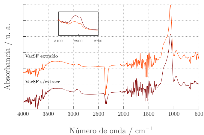
Figura A.21: Espectro de absorción de IR correspondiente a una VacSF, antes y después de la extracción con 2-propanol.
