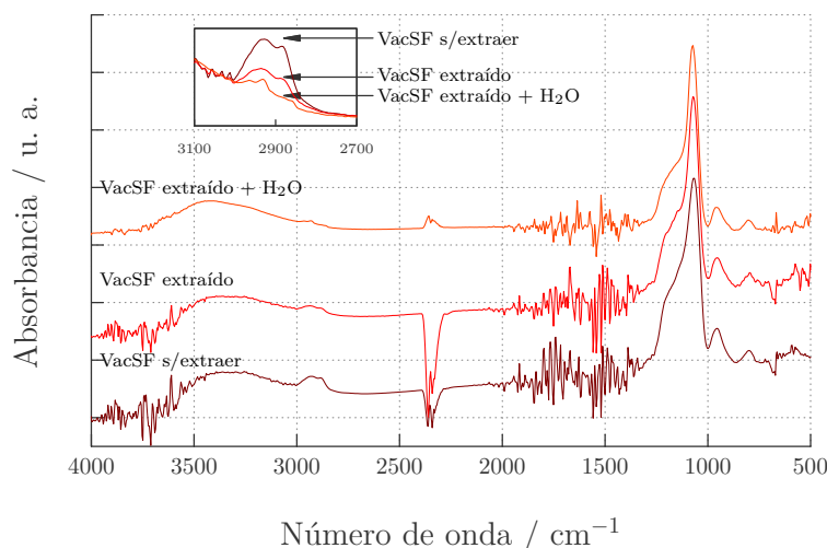
Figura 3.23: IR para cada etapa de eliminación del surfactante correspondiente a una SF sintetizada por el método de alto vacío.
