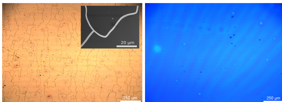
Figura A.17: Microscopías ópticas para VacSC. Izquierda: sobre sustrato de Au. Derecha: sobre sustrato de Si.
