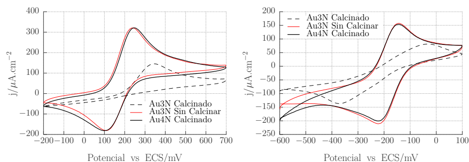
a. Voltametrías cíclicas para FeCN 1 mM tomadas a 50 mV s -1 en una solución 0,1 M de KCl.
