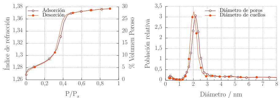
a. Isoterma de adsorción/desorción de agua realizada por PEA para una SimSC. b. Distribución de tamaño de poro y cuello.
