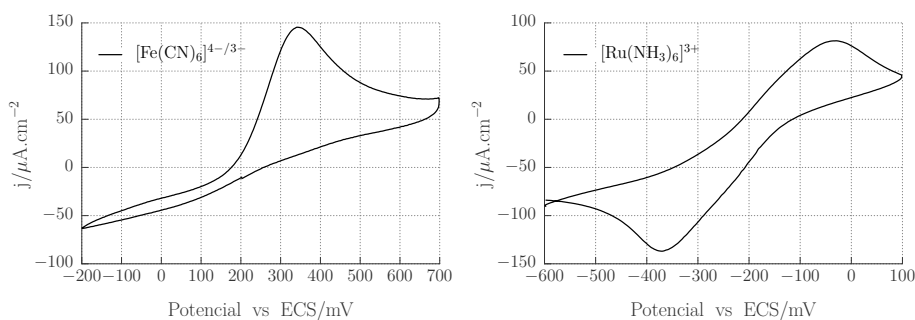
Figura 5.13: Voltametrías para [\text{Fe}(\text{CN})_6]^{4-}/3- (izquierda) y [\text{Ru}(\text{NH}_3)_6]^{3+} (derecha) tomados a 50 \text{ mV s}^{-1} sobre electrodos de Au calcinados, en los cuales la respuesta es deficiente para ambas sondas, producto de una transferencia electrónica impedida.
