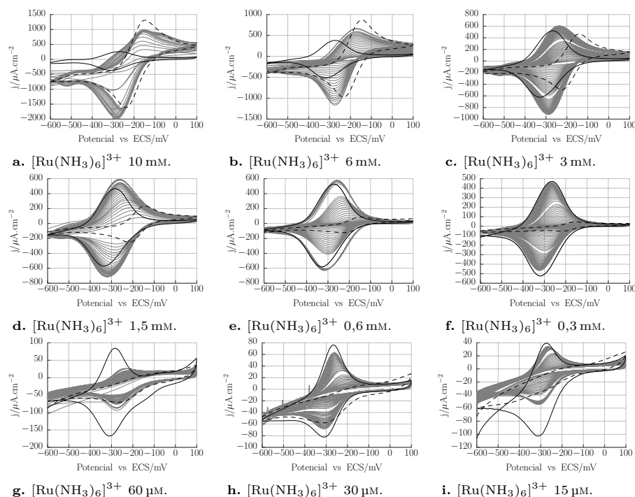
Figura 4.9: Adsorción de ARu en PDM a diferentes concentraciones de la sonda. Los voltagramas grises (—) indican el ingreso de la sonda en la red mesoporosa, los de línea sólida (—) corresponden a la sonda adsorbida en solución con electrolito soporte únicamente y los voltagramas de línea punteada (- -) son la respuesta en electrodos de Au desnudo. Todos los voltagramas fueron medidos a 50 \text{ mV s}^{-1} en solución de KCl 100 mM.
