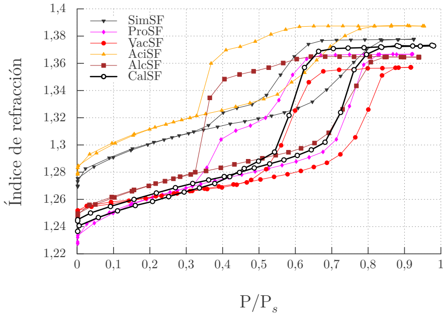
Figura 3.21: Comparación de las isotermas para todos los tratamientos posdeposición para SF. Se destacan la doble distribución de cuellos (SimSF, ÁciSF y AlcSF) sugiriendo dos tamaños de cuellos o dos sistemas porosos independientes.
