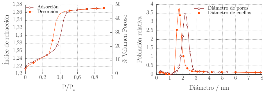
a. Isoterma de adsorción/desorción de agua realizada por PEA para una AlcSC. b. Distribución de tamaño de poro y cuello.
