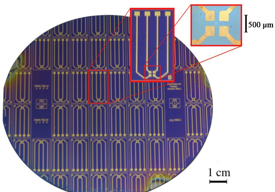
Figura 5.11: Primer diseño de los sensores. Oblea de silicio de 10 cm de diámetro, capa de SiO 2 y 32 sensores con cuatro electrodos de trabajo cada uno.
