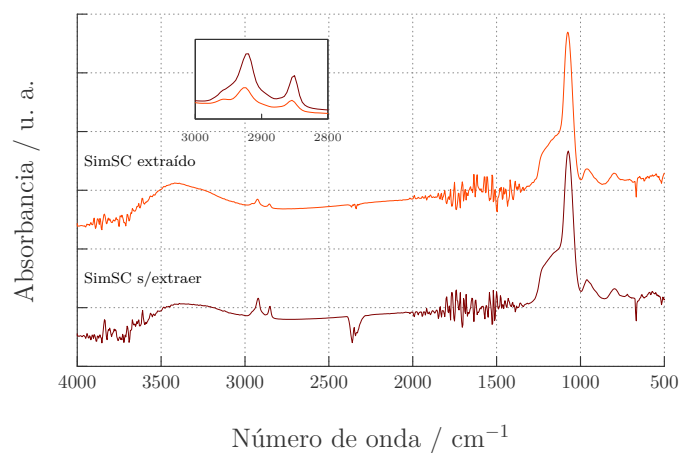
Figura A.9: Espectro de absorción en el IR para una SimSC sintetizada con el tratamiento simplificado antes y después de extraer el surfactante. Todavía se puede apreciar un cantidad pequeña de surfactante luego de la extracción.
