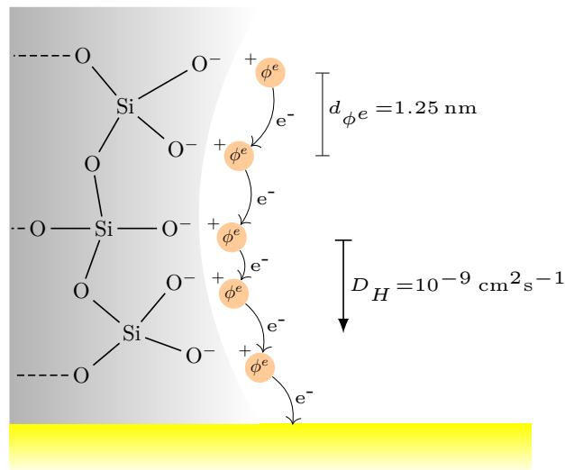
Figura 4.11: Diagrama en el cual se ejemplifica el mecanismo de transferencia y transporte de carga mediante saltos electrónicos o electron hopping .
