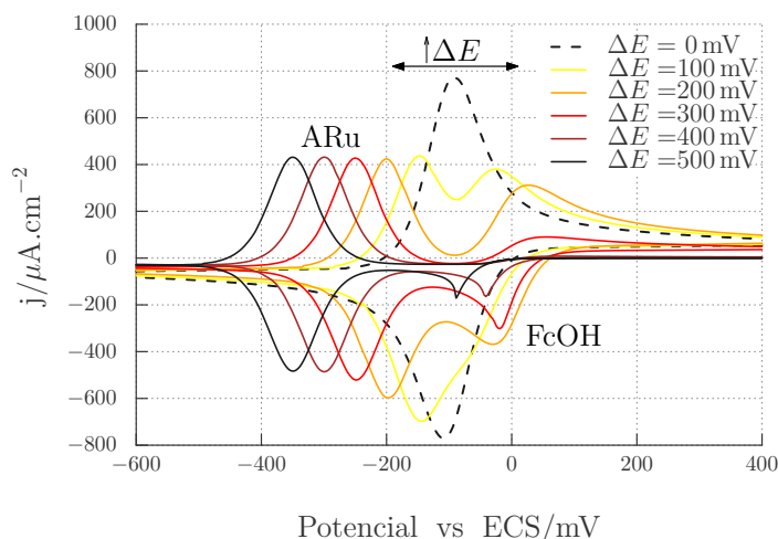
Figura 4.16: Simulación por elementos finitos de voltagramas cíclicos para la mediación entre una sonda en solución y una SF con \text{ARu} 1 mM. En el eje de la abscisas se coloca la diferencia de potencial estándar para cada una de las sondas con ECS.
