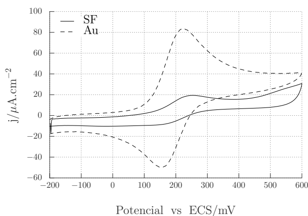
Figura 4.4: Respuesta comparativa de FcOH 1 mM sobre un electrodo de Au recubierto con SF y uno sin recubrir en 0,1 M de KCl, a 50 \text{ mV s}^{-1} utilizando como referencia un ECS.
