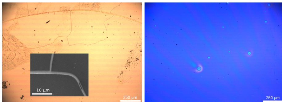
Figura A.5: Microscopías ópticas para SimSC. Obsérvese las grietas presentes cuando se sintetiza sobre Au (izquierda), mientras que sobre Si las SimSC no presentan rupturas ni discontinuidades.
