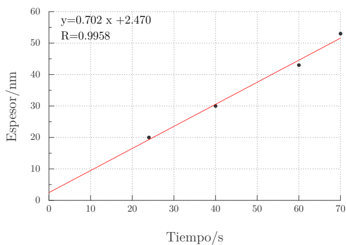
Figura 5.9: Curva de calibración para establecer la velocidad de depósito de la capa de Au. La misma se realizó por pulverización catódica en las condiciones experimentales detalladas en la tabla 2.6.
