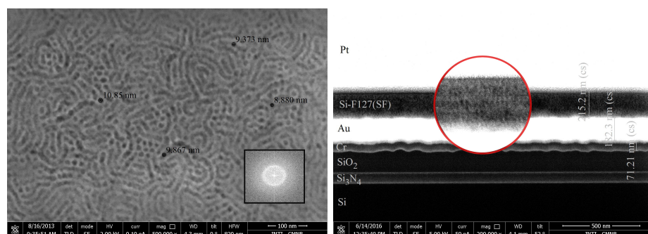
a. MEB donde se observa la superficie de una SF con poros de 10 nm de diámetro en promedio. Recuadro: FFT de la imagen completa.
