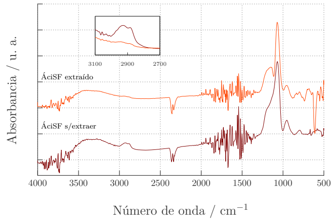
Figura A.27: Espectro de absorción en el IR para una ÁciSF antes y después de extraer el surfactante.
