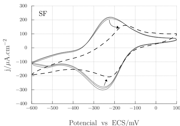
Figura 3.4: Serie de voltametrías cíclicas consecutivas, del ciclo 39 al 42, donde se evidencia la pobre adherencia de SF sobre electrodos de Au. Las flechas negras indican un cambio repentino en el comportamiento, de un electrodo recubierto con una PDM a un electrodo desnudo (curva punteada). Las VC fueron tomadas a 50 \text{ mV s}^{-1} usando de referencia ECS y con sonda ARu 1 mM.
