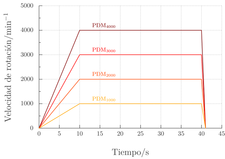
Figura 2.2: Esquema con las rampas de velocidad de rotación o velocidad angular mas frecuentemente utilizadas para el depósito de PDM. A mayor velocidad y mayor tiempo, menor es el espesor de los depósitos resultantes.
