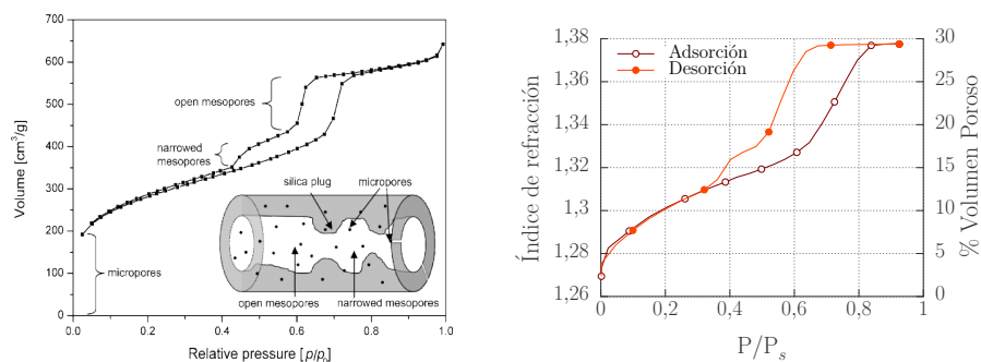
a. Efecto de poros bloqueados en sílice calcinada estructurada con Pluronic 123.
