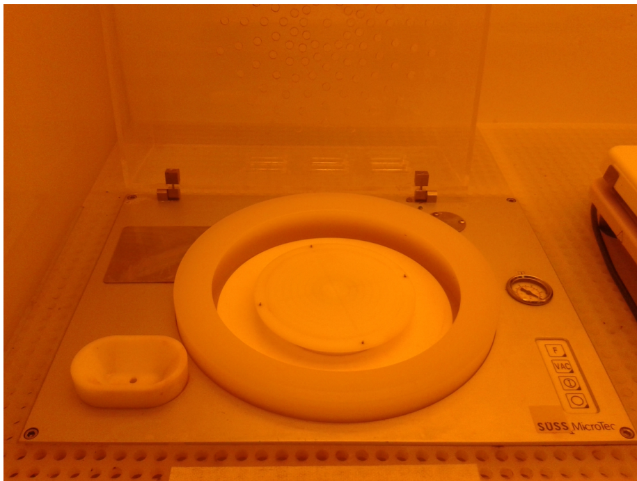
Figura 2.3: Spin-coater ubicado en el Laboratorio de Fotolitografía del INTI-CMNB utilizado para el depósito de las películas delgadas mesoporosas, Marca Suss MicroTec , modelo Delta 20BM .
