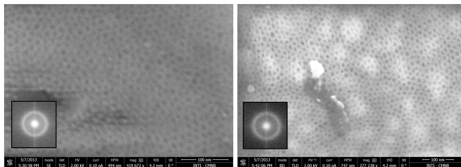
Figura 3.10: Microscopía electrónica de barrido de sistemas CalSF y sus respectivas FFT. Se observa la distribución y homogeneidad de los poros en superficie. Izquierda: sobre sustrato de silicio. Derecha: sobre sustrato de Au.
