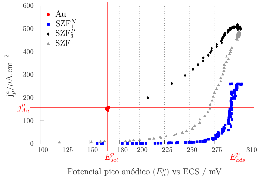
Figura 4.30: Intensidad de corriente de pico anódico vs potencial de pico de [\text{Ru}(\text{NH}_3)_6]^{3+} para diferentes funcionalizaciones sobre películas delgadas mesoporosas de \text{Si}_{0,9}\text{Zr}_{0,1}\text{O}_2 . Los puntos rojos corresponden a la señal de un electrodo de Au desnudo.
