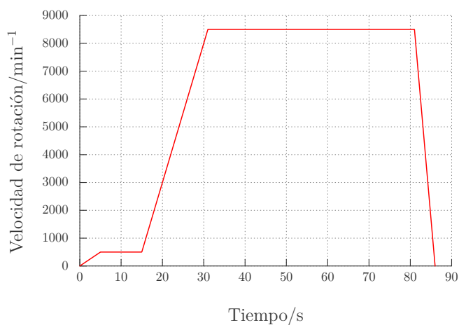
Figura 2.13: Esquema de aceleración y velocidad de rotación para el depósito de la fotorresina epoxi SU8.
