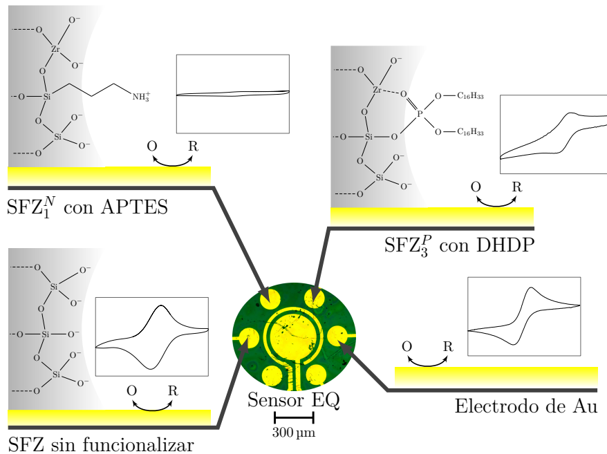
Figura 5.17: Microscopía óptica de un sensor con múltiples electrodos recubiertos con películas delgadas mesoporosas de \text{Si}_{0.9}\text{Zr}_{0.1}\text{O}_2 . Uno se dejó sin recubrir mientras que dos fueron funcionalizados con DHDP y APTES respectivamente. A modo ilustrativo se muestra un esquema de la estructura de las películas en cada caso y una típica respuesta EQ para cada uno de ellos.
