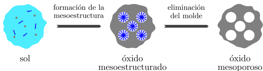
Figura 1.7: Esquema general para la formación de un óxido mesoporoso combinando precursores inorgánicos y tensioactivos para la moldear los poros.
