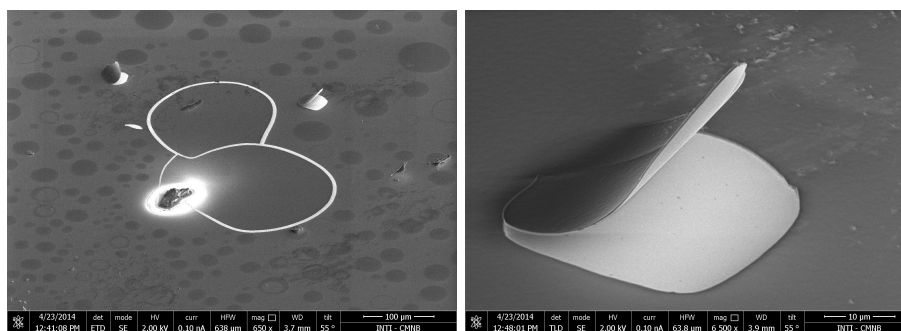
Figura 3.5: MEB donde se muestra la falta de adherencia de SC sobre una película delgada de Au. Obsérvese los círculos grises que corresponden a PDM elevadas en forma de cúpula y separadas del sustrato. La imagen de la derecha muestra una porción de SC despegada y elevada.
