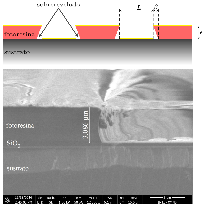
Figura 5.4: Arriba: esquema de la fotorresina depositada y revelada, donde se muestra la relación de espesor respecto del ancho de línea y el sobre-revelado necesario para un correcto decapado. Abajo: corte por FIB para evaluar el sobre-revelado y espesor obtenido luego de la transferencia por litografía.
