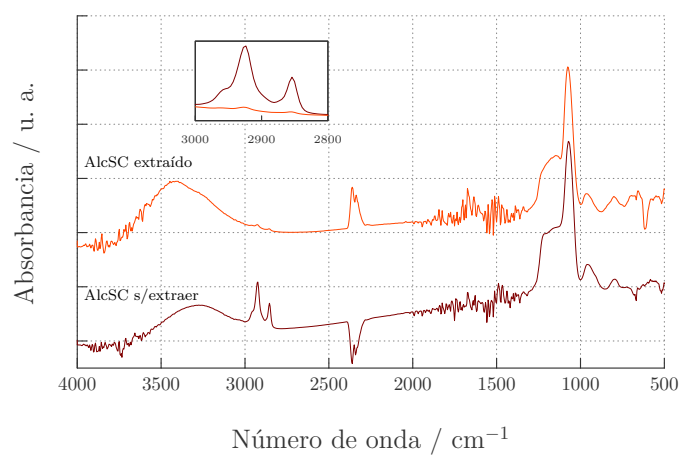
Figura A.34: Espectro de absorción en el IR para una AlcSC antes y después de extraer el surfactante. Obsérvese la ausencia de hombro en la región 1250-1100 cm -1 , el cual es típico en sistemas de SiO 2 mesoestructuras.
