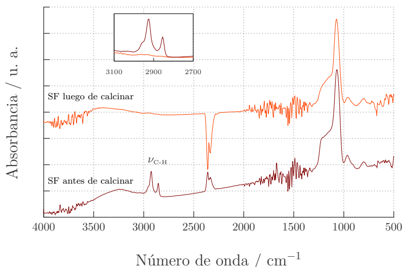
Figura 3.15: Espectro de absorción para una SF antes y después de calcinar, donde se puede apreciar la aparición de una banda fuerte la cual corresponde al surfactante F127.
