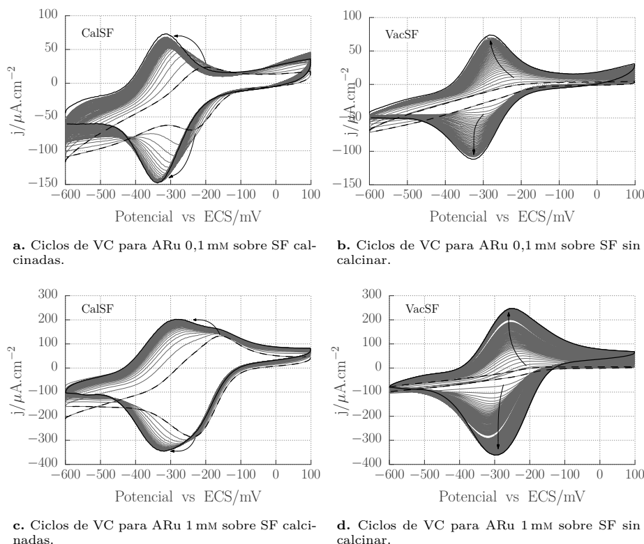
Figura 3.24: Voltametrías cíclicas donde se compara la accesibilidad de una sonda electroquímica sobre SF con dos tratamientos posdepósito diferentes. Las curvas punteadas corresponden al primer ciclo, las grises a los sucesivos ciclos y las negras a la máxima capacidad de adsorción para cada concentración de sonda. (a) y (c) Método de calcinación a (350 °C) y, (b) y (d) Método de alto vacío (130 °C, 7 días, P=10^{-5} mbar). Todas las VC fueron realizadas en una solución 0,1 M de KCl a 50 \text{ mV s}^{-1} .
