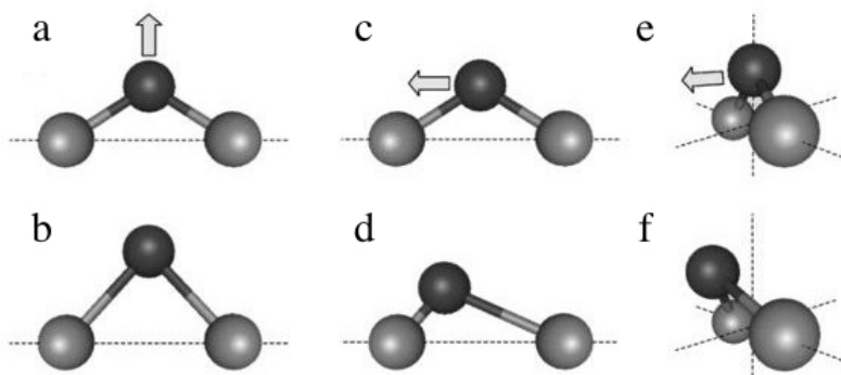
Figura 3.13: Representación de los movimientos de vibración del oxígeno (gris oscuro) respecto de los átomos de silicio (gris claro). (a) y (b) Estiramientos simétricos perpendiculares al plano Si-Si. (c) y (d) Estiramientos antisimétricos paralelos a la recta Si-Si. (e) y (f) Balanceos perpendiculares al plano Si-O-Si. La figura fue adaptada de la publicación de Innocenzi, J. Non. Cryst. Solids, 316(2-3), p. 309-319.
