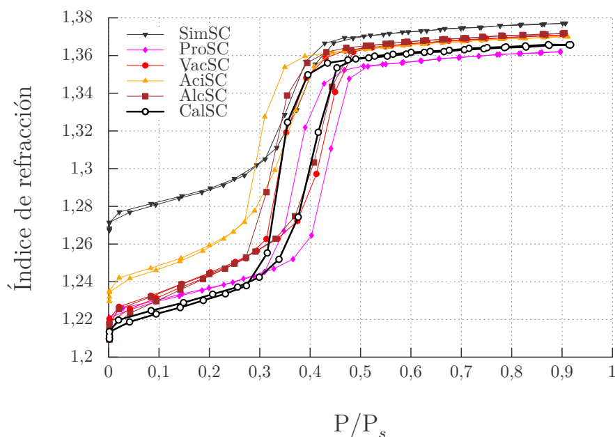
Figura 3.20: Comparación de las isotermas para todos los tratamientos posdeposición para SC. Destacan los altos valores para el índice de refracción de los tratamientos simplificado y en medio ácido.
