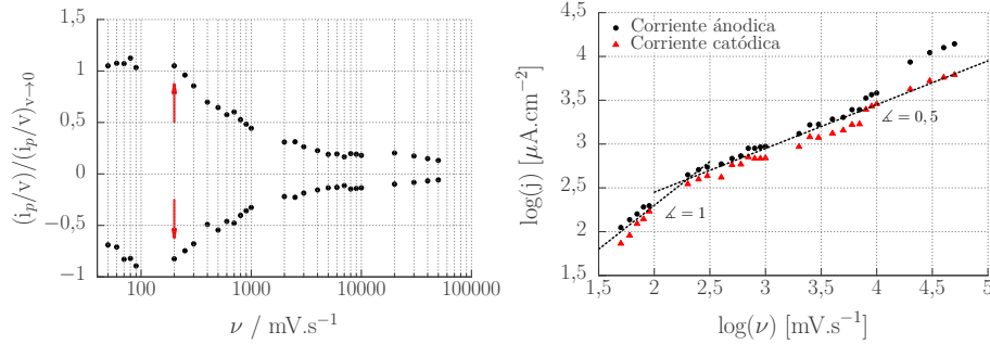
a. Intensidad de pico en función de la velocidad de barrido. Las flechas rojas indican la velocidad característica para el cambio de régimen. b. \log(i_p) vs \log(\nu) para determinar el cambio de régimen.
