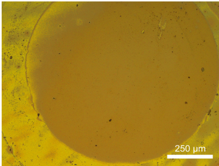
Figura A.35: Microscopía óptica de una SF luego de realizar 90 ciclos electroquímicos. Se puede observar el Au desnudo del electrodo donde se colocó el sello de la celda electroquímica, indicando la disolución de la película mesoporosa.
