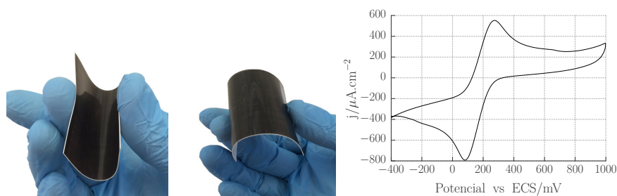
Figura 6.3: Electrodo basados en nanotubos de carbono impresos por inyección de tinta en donde se muestra la flexibilidad de la tinta y su respuesta electroquímica con una sonda de FeCN 2,5 mM en solución de KCl 100 mM a 50 \text{ mV s}^{-1} .
