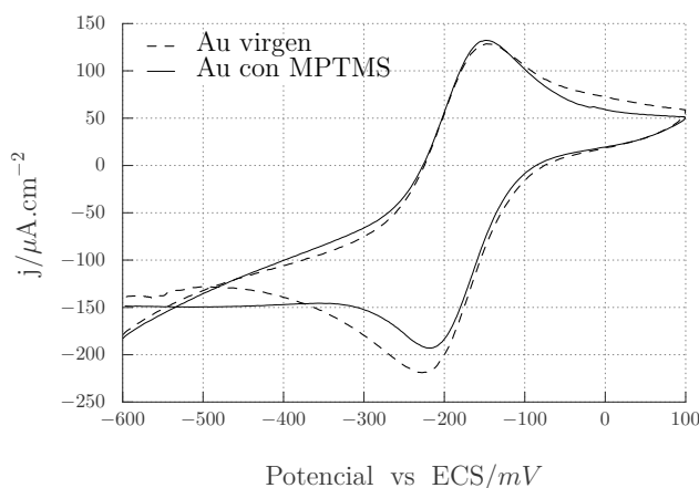
Figura 3.9: VC para [\text{Ru}(\text{NH}_3)_6]^{3+} 1 mM a 50 \text{ mV s}^{-1} sobre un electrodo virgen de Au (punteado) comparado con uno funcionalizado con MPTMS (sólido). La funcionalización no bloquea ni modifica el desempeño electroquímico de los electrodos.
