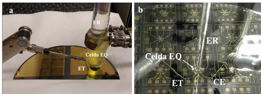
Figura 2.21: Fotografía del instrumental que se utilizó a lo largo de la tesis para tomar las medidas electroquímicas. Izquierda: celda de acrílico sobre electrodos de Au recubierto con una PDM utilizando CE y ER externos. Derecha: oblea con 6 ET por sensor, celda fabricada con resina epoxi SU8, CE integrado y utilizando un ER externo.
