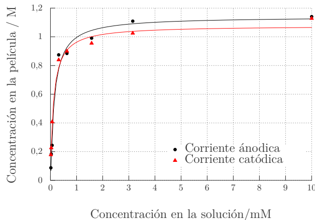
Figura 4.10: Isoterma de Langmuir a T=25^\circ\text{C} donde se gráfica la concentración de [\text{Ru}(\text{NH}_3)_6]^{3+} adsorbido en función de la concentración en solución colocada inicialmente.
