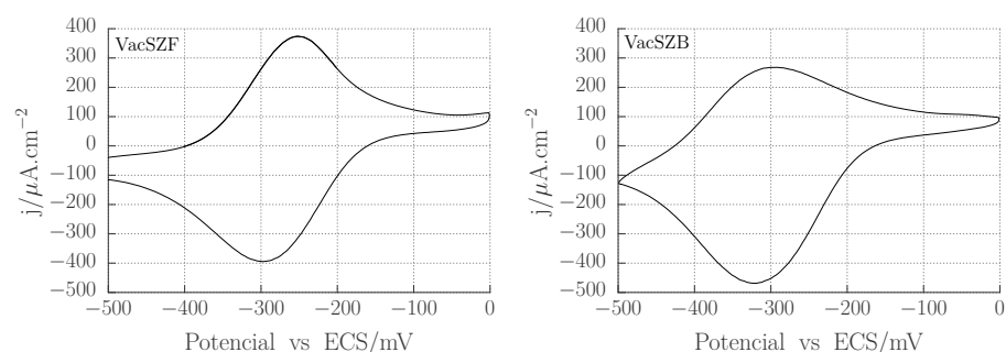
a. Voltametría Cíclica sobre VacSZF correspondiente al ciclo número 95.
