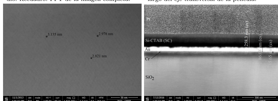
c. MEB donde se observa la superficie regular de muestra SC con poros de 3 nm de diámetro en promedio.
