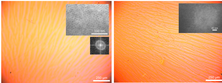
Figura A.18: Microscopías ópticas para VacSZF depositadas sobre electrodos de Au. Izquierda: Utilizando F127 como surfactante. Derecha: Utilizando Brij58 como surfactante.
