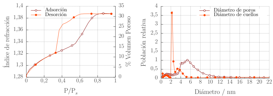
a. Isoterma de adsorción/desorción de agua realizada por PEA para una ÁciSF. b. Distribución de tamaño de poro y cuello.
