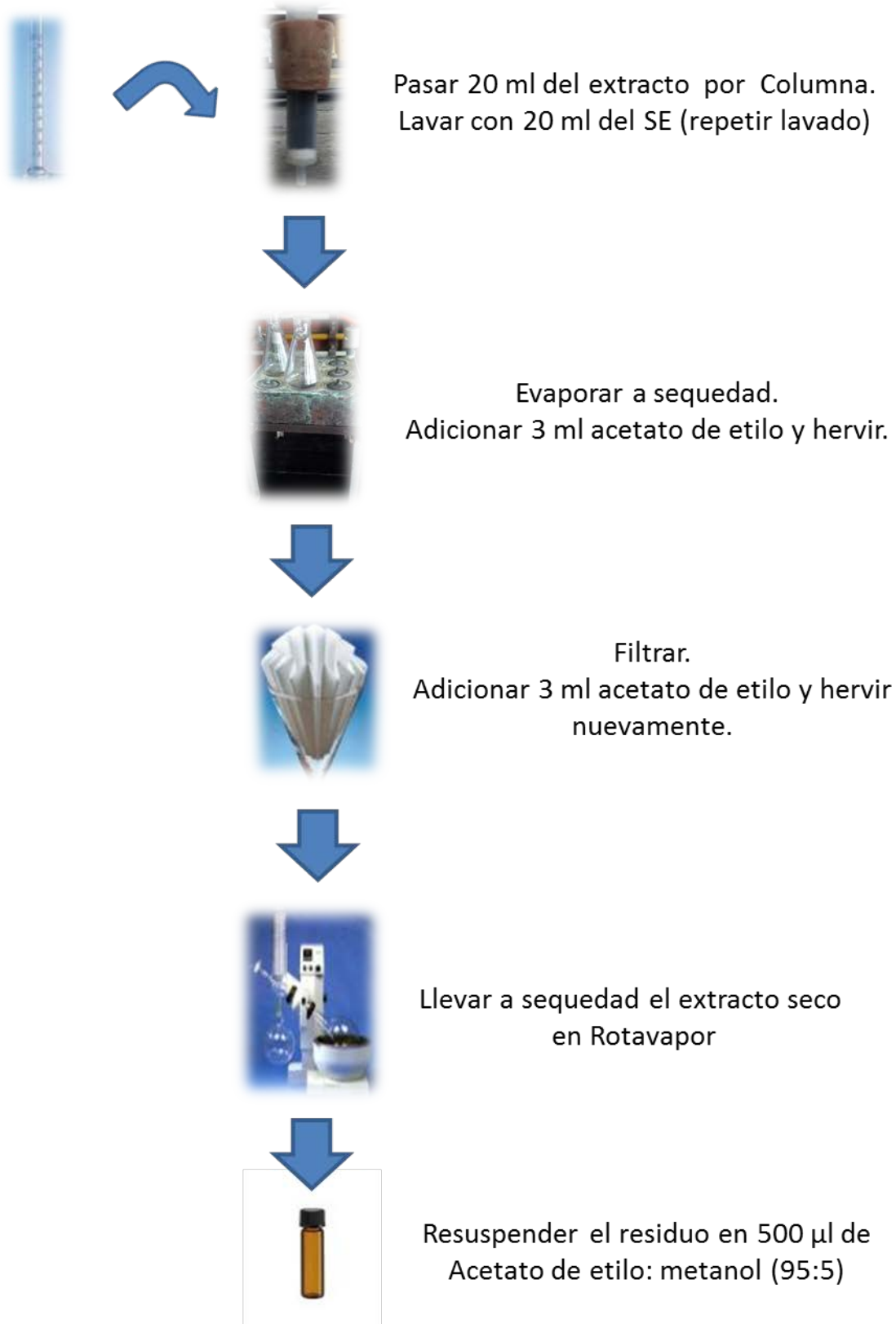
Figura 11 Esquema del proceso de purificación
