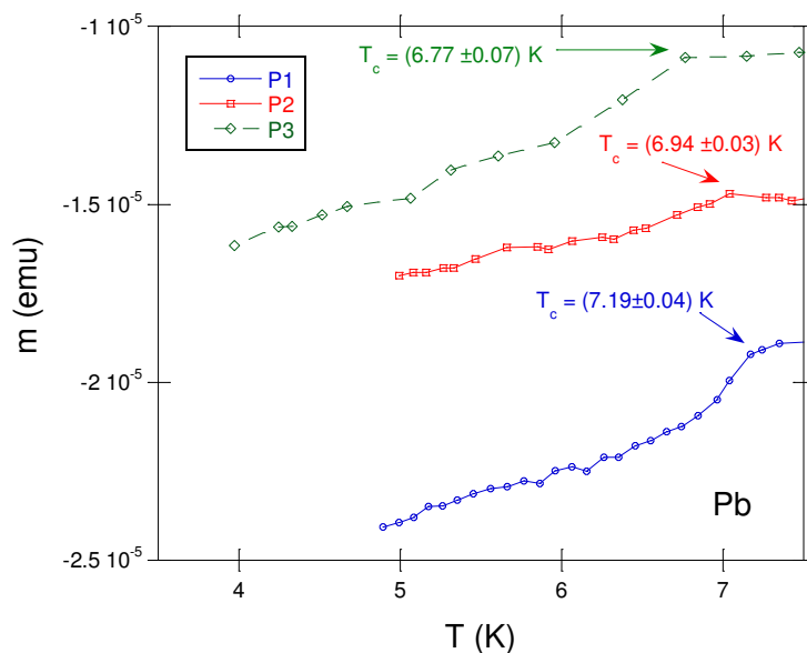
Figura 6.3.1.1: m vs T para el compuesto Pb con tres presiones distintas.
