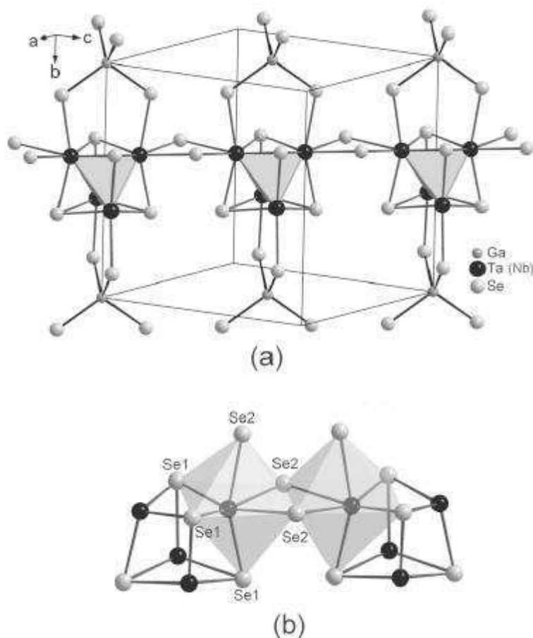
Figura 2.1.1: a) Estructura FCC del tipo \text{GaMo}_4\text{Se}_8 , para los compuestos \text{GaTa}_4\text{Se}_8 y \text{GaNb}_4\text{Se}_8 ; b) Átomos de Ta desplazados del centro de la estructura octaédrica de \text{Se}_6 . Figuras extraídas de la bibliografía [2.1.1] .
