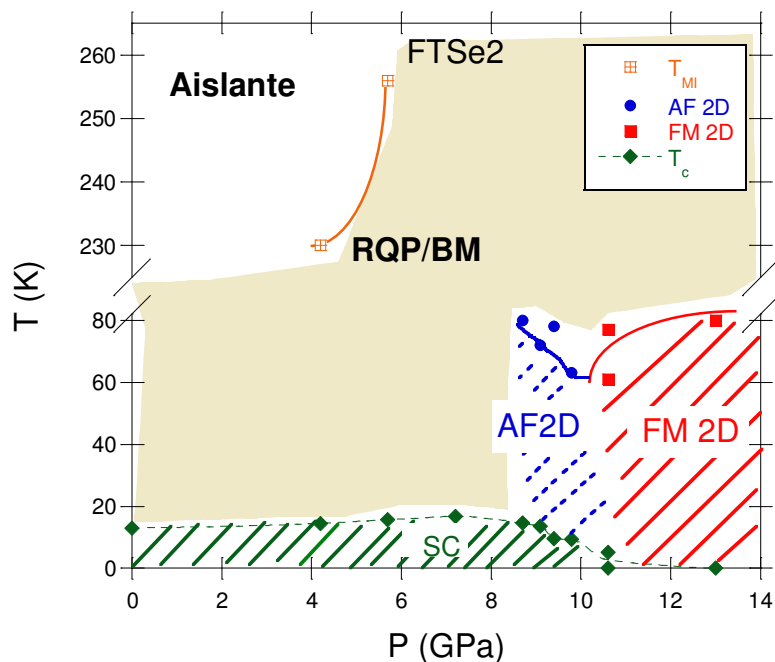
Figura 8.4.4: Diagrama de fases de T vs P del cristal FTSe2 (las líneas que unen los puntos son para guiar al ojo). Se indican las zonas donde se desarrolla el estado SC ( T_c ), aquellas con un transporte del tipo BM/RQP y donde el transporte eléctrico está dominado por fluctuaciones de espín (AF 2D y FM 2D).
