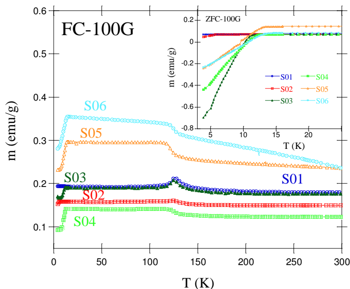
Figura 7.2.3: m en función de T con el protocolo FC para las muestras S01-S06. En la figura insertada se muestra las curvas medidas con el protocolo ZFC.
