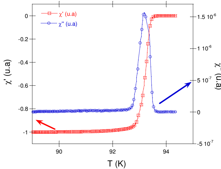
Figura 5.3.1: \chi'' y \chi' vs T para la muestra de \text{YBa}_2\text{Cu}_3\text{O}_{7-\delta} medido a una frecuencia de 90.6 kHz.
