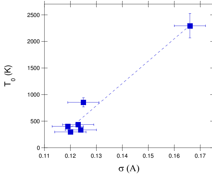
Figura 7.3.2: Parámetro T_0 en función del desorden \sigma .
