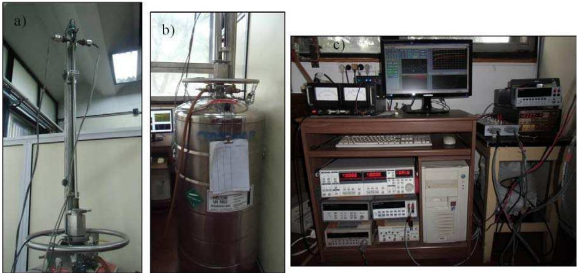
Figura 6.1.5: a) Crióstato de acero inoxidable montada en el sistema automático (de aluminio); b) termo con He utilizado para alcanzar temperaturas cercanas a los 4 K; c) Dispositivos electrónicos utilizados para realizar las mediciones.
