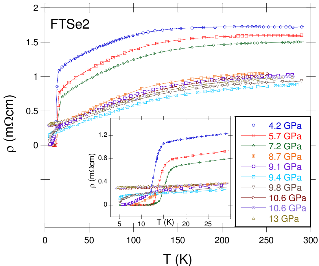
Figura 8.3.1: \rho vs T a distintas presiones para el cristal FTSe2. En la figura insertada se muestra en detalle la transición superconductora.
