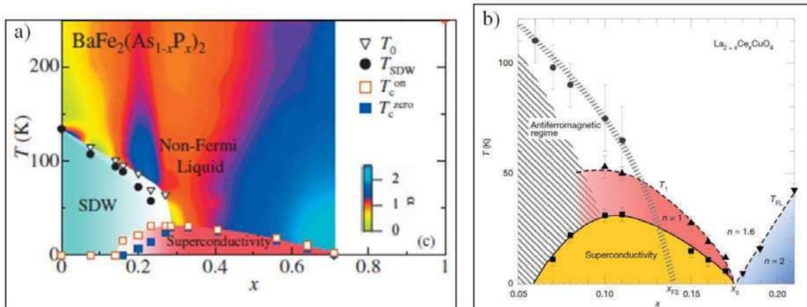
Figura 1.5.2: a) Diagrama de fases de T vs contenido de fósforo en el compuesto \text{BaFe}_2(\text{As}_{1-x}\text{P}_x)_2 , donde se muestra un posible QCP; b) Diagrama de fases de T en función del dopaje del cuprato \text{La}_{2-x}\text{Ce}_x\text{CuO}_4 , donde se marca un posible QCP en x_c = 0.175
