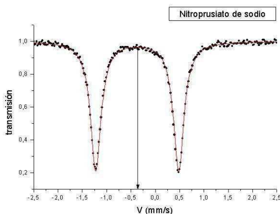
Figura C.2: Espectro Mössbauer para el nitroprusiato de sodio a temperatura ambiente [C.4].
