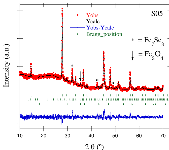
Figura 7.1.3: Difractograma de la muestra S05 (en rojo) y su correspondiente refinamiento Rietveld (línea negra). La diferencia entre los valores observados y los calculados se marcan con una línea azul y las líneas verticales verdes corresponden a las posiciones de Bragg. Las impurezas también se indican.
