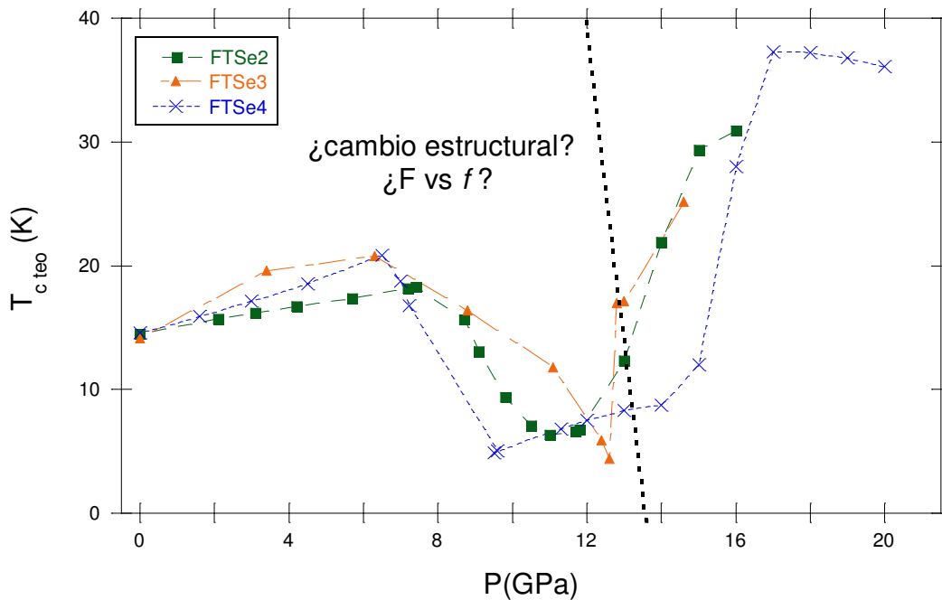
Figura 9.6: T_c teórica vs P calculada a partir del modelo para las muestras FTSe2, FTSe3 y FTSe4. La línea punteada marca un posible cambio estructural (ver figura 8.39).
