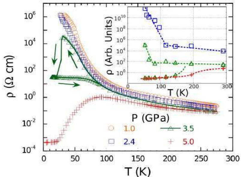
Figura 10.1: Resistividad en función de la temperatura para presiones de 1 a 5 GPa medidas en el cristal GTS (muestra A). En la figura insertada se muestran los resultados obtenidos de \rho(T) con los cálculos LDA+DMFT (ver explicación más abajo). Las líneas sirven para guiar al ojo.
