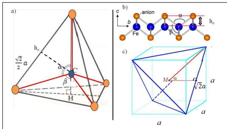
Figura 1.1.7: a) Esquema de la estructura de un tetraedro, donde se marca los parámetros h_a y a . La esfera azul en el medio de la figura representa al Fe, mientras que las esferas naranjas son los aniones; b) Representación gráfica del h_a , donde se marcan los ángulos \alpha y \beta ; c) Estructura del tetraedro dentro de una estructura cúbica, donde se define el lado del tetraedro en función del lado de la celda unidad cúbica a .
