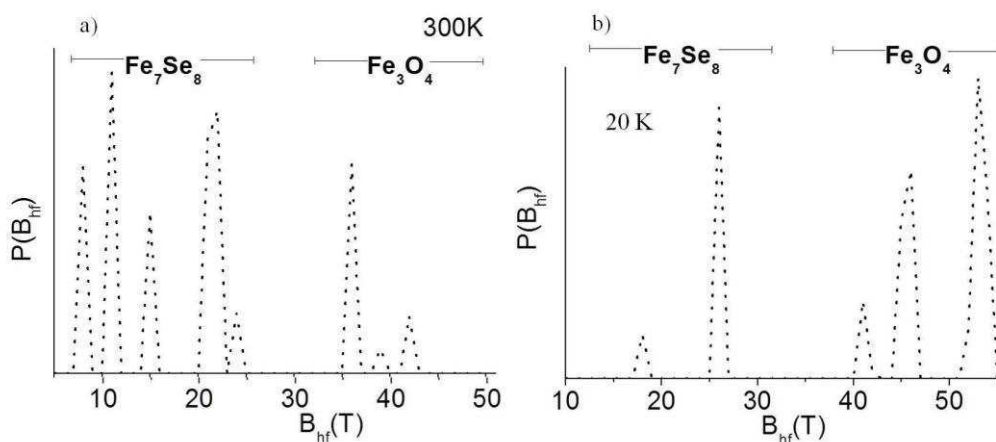
Figura 8.1.7: Distribución de campos hiperfinos para las impurezas magnéticas de \text{Fe}_7\text{Se}_8 y \text{Fe}_3\text{O}_4 ; a) Temperatura ambiente y b) 20 K.
