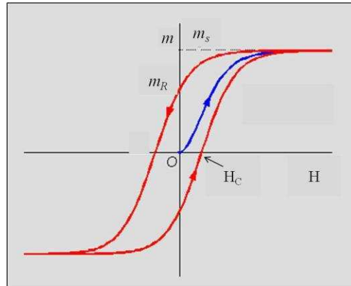
Figura 5.1.1: Curva típica m vs H de un material ferromagnético. En la figura se indican la magnetización remanente ( m_R ), la magnetización de saturación ( m_s ) y el campo coercitivo ( H_c ).
