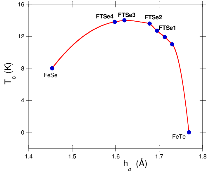
Figura 8.1: Curva T_c vs h_a para la familia FTSe [8.1-8.3] .
