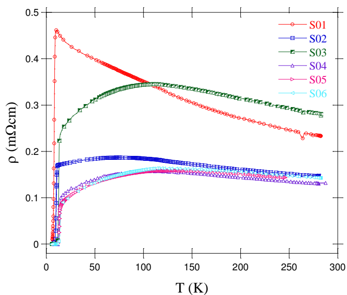
Figura 7.2.1: \rho vs T para las muestras S01-S06.
