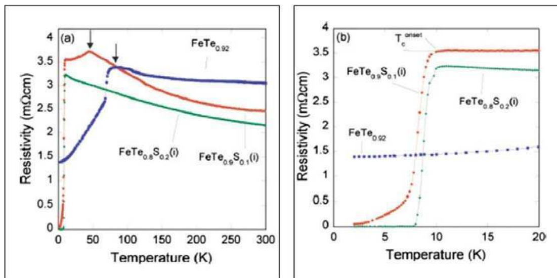
Figura 1.2.4: Curva de \rho en función de la temperatura para la familia Fe_{1+y}Te_{1-x}S_x [1.2.8] a) para todo el rango de temperatura; b) detalle de la T_c .
