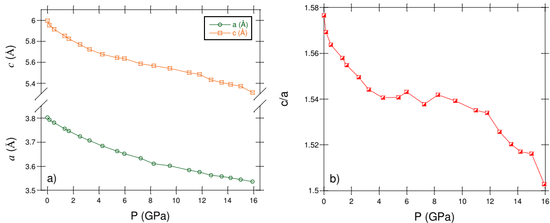
Figura 8.3.7: a) Parámetros estructurales a y c vs P ; b) c/a vs P para el cristal FTSe3
