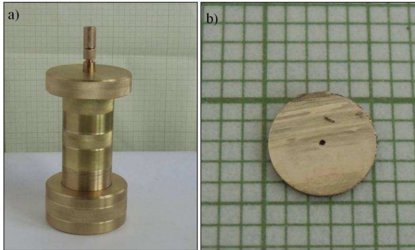
Figura 6.3.2:a) Foto del cuerpo de la celda para el SQUID dentro del soporte; b) Foto del gasket.
