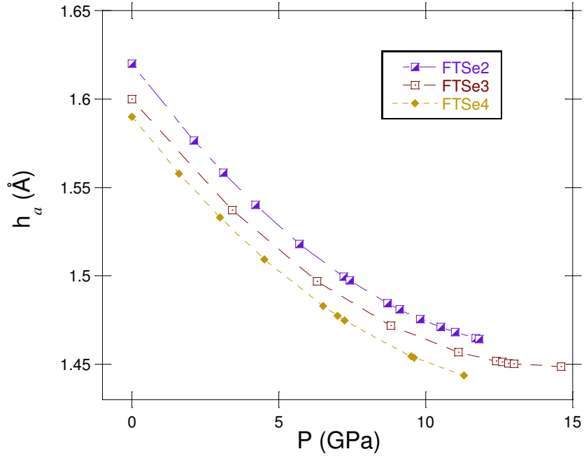
Figura 9.3: h_a vs P para las muestras FTSe2, FTSe3 y FTSe4 calculados a través del modelo de T_c [ver ec. (9.1)] y b(a) (ver fig.9.2).
