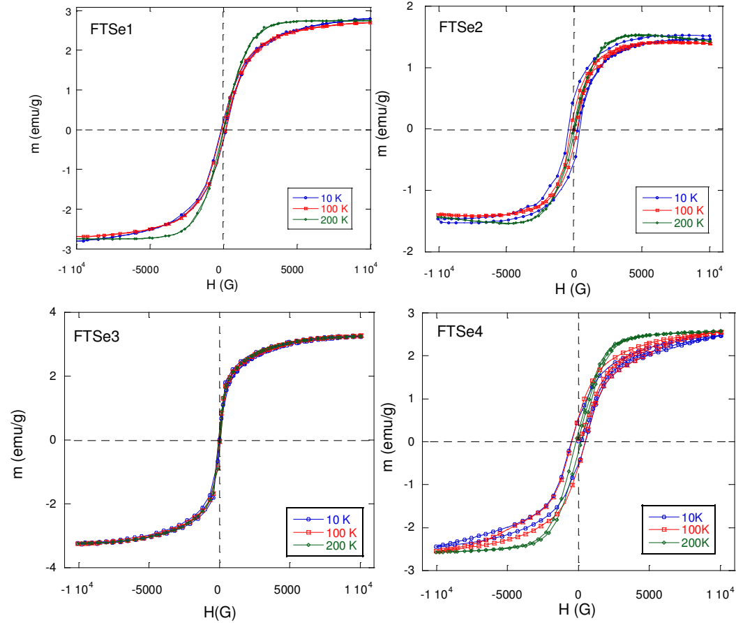
Figura 8.2.2: m vs H para la familia FTSe, medidas a 10 K, 100 K y 200 K.
