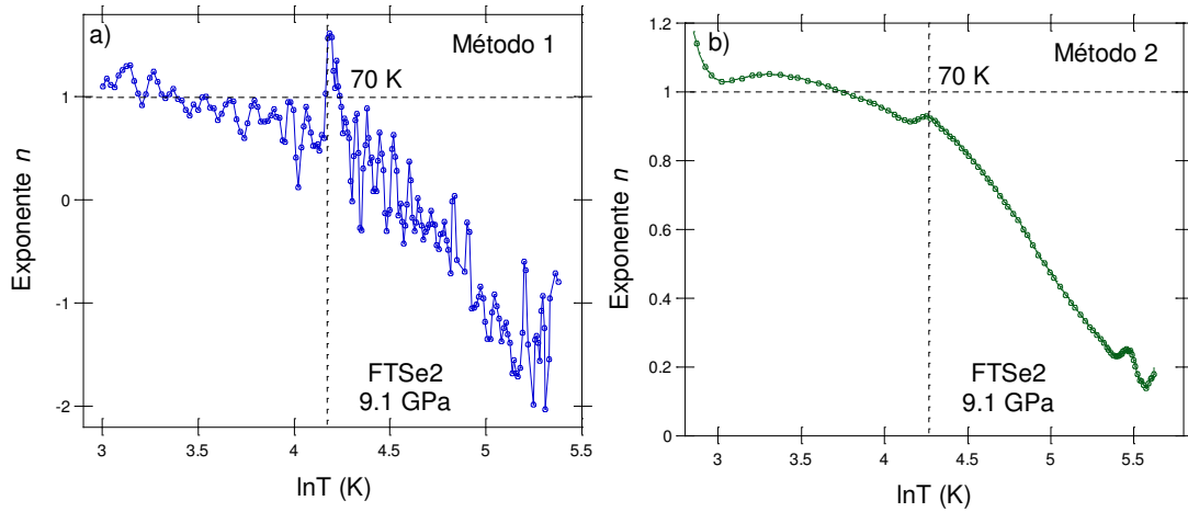
Figura 8.4.2: Exponente n vs \ln T obtenido con: a) método 1 y b) método 2 para el cristal FTSe2 a 9.1 GPa.
