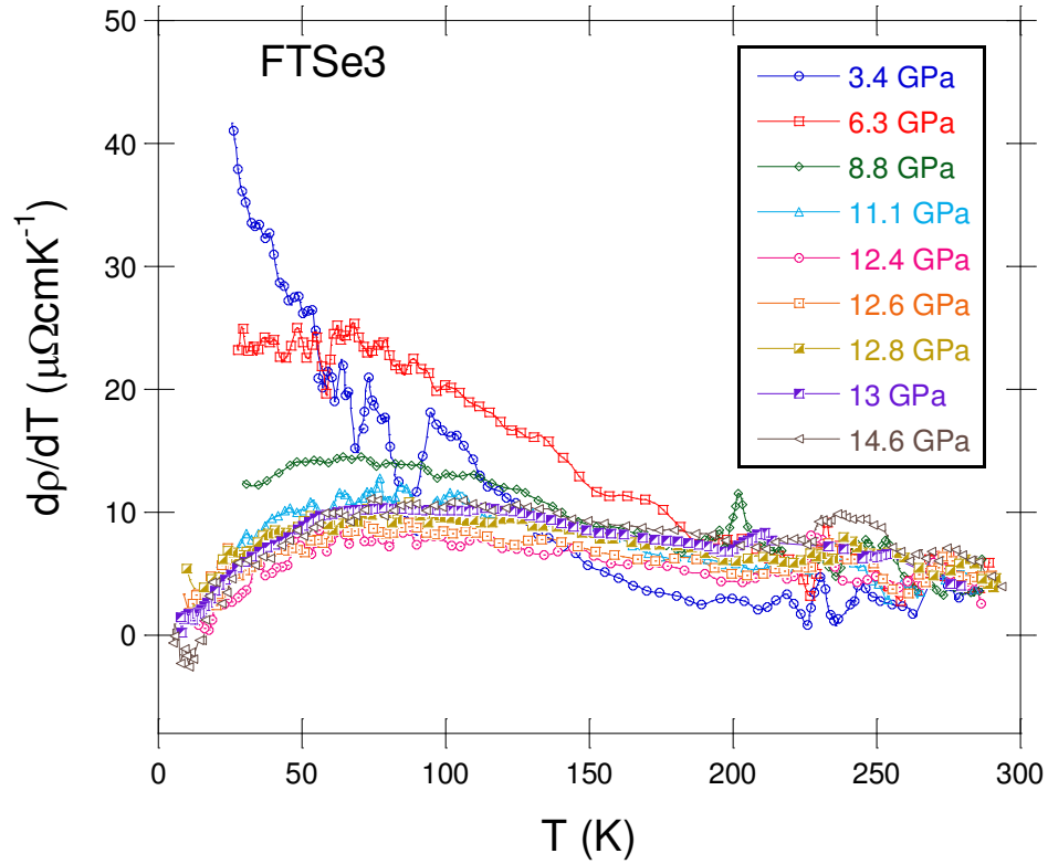
Figura 8.4.5: Curva dp/dT vs T para el cristal FTSe3.
