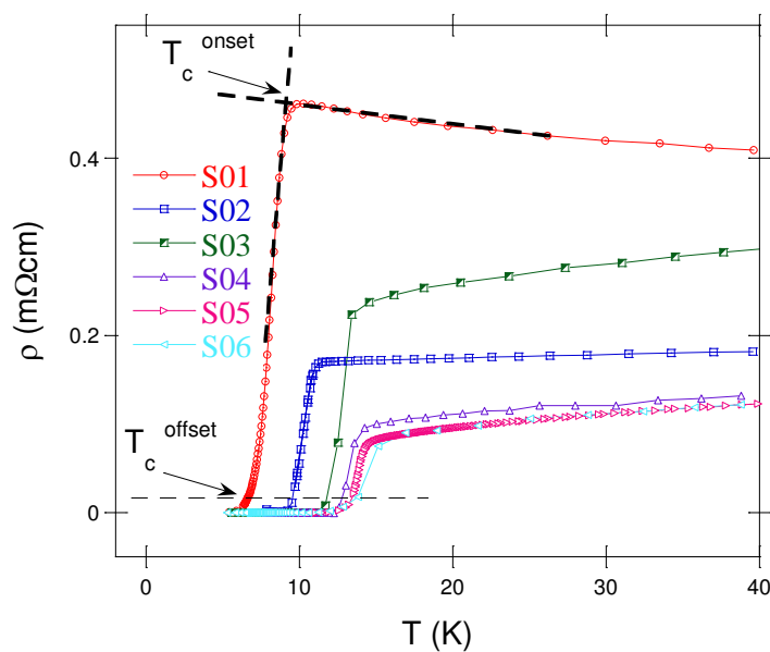
Figura 7.2.2: Detalle a bajas temperaturas de \rho vs T para las muestras S01-S06.
