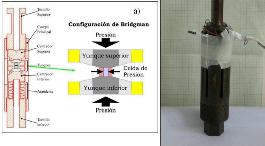
Figura 6.1.2: a) Esquema de la celda cuasi-hidrostática con yunques del tipo Bridgman; b) Foto del cuerpo principal de la celda.
