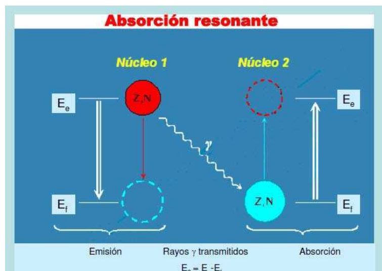
Figura C.1: Esquema de la absorción resonante para la técnica Mössbauer [C.2] .
