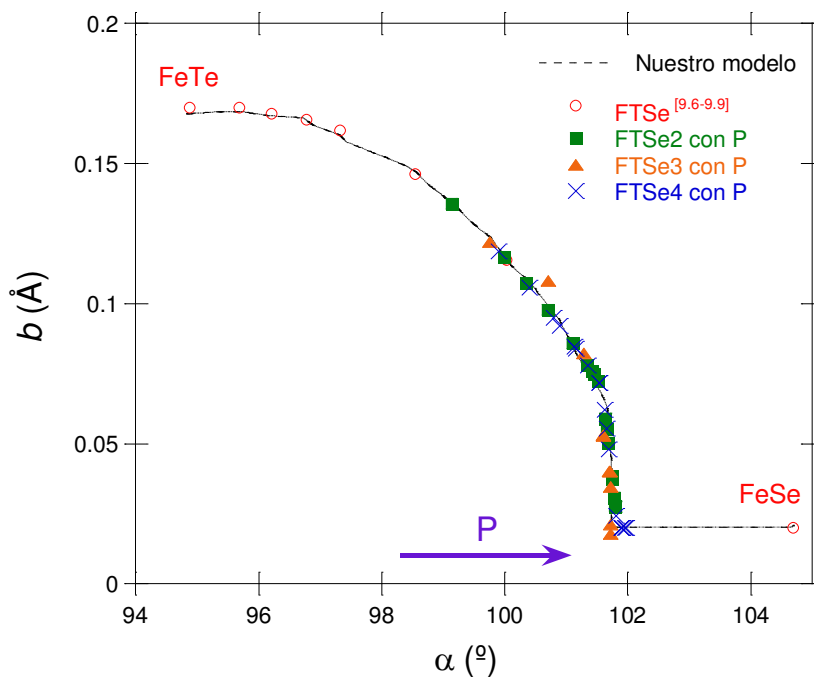
Figura 9.2: Parámetro de control b en función del ángulo \alpha para la familia FTSe con y sin presión.
