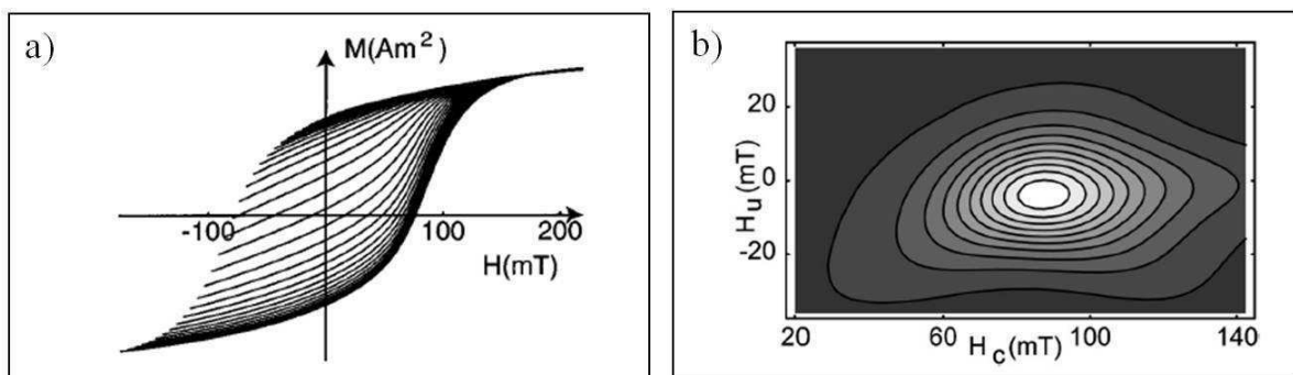
Figura 5.2.1: a) Conjunto de curvas FORC, esquema obtenido del artículo del autor Pike [5.2.1] , b) Curvas de nivel del diagrama de FORC correspondiente.
