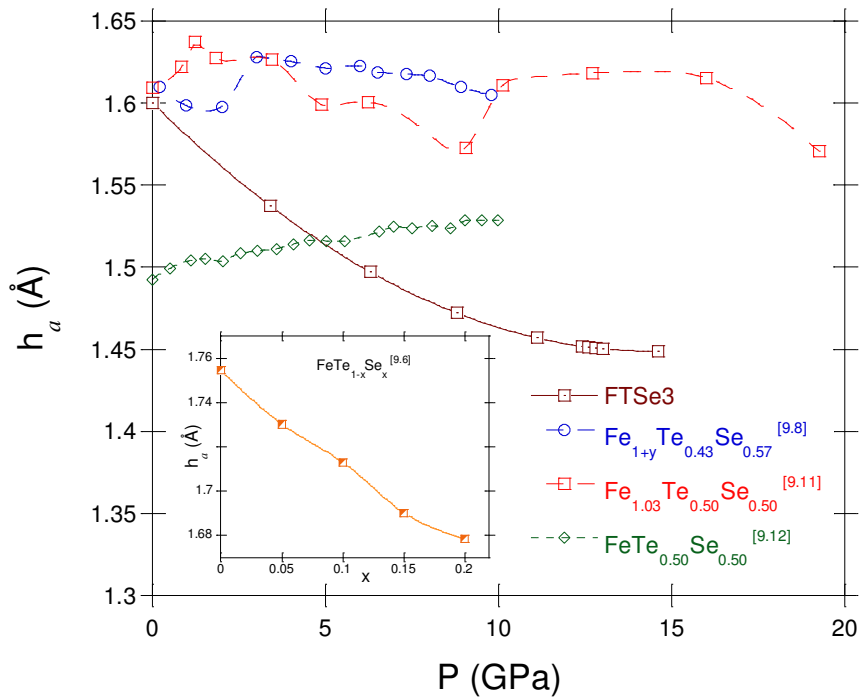
Figura 9.4: h_a vs P para las muestras FTSe3, \text{Fe}_{1+y}\text{Te}_{0.43}\text{Se}_{0.57} [9.8], \text{Fe}_{1.03}\text{Te}_{0.50}\text{Se}_{0.50} [9.11] y \text{FeTe}_{0.50}\text{Se}_{0.50} [9.12]. En la figura insertada se muestra h_a vs x para \text{FeTe}_{1-x}\text{Se}_x [9.6].
