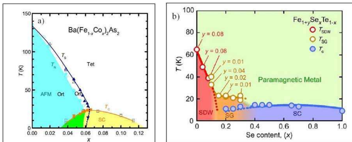
Figura 1.3.1: a) Diagrama de fases magnético y estructural de T vs dopaje “ x ” para el compuesto \text{Ba}(\text{Fe}_{1-x}\text{Co}_x)_2\text{As}_2 [1.3.1]; b) Diagrama de fases magnético para \text{Fe}_{1+y}\text{Te}_{1-x}\text{Se}_x [1.3.2].
