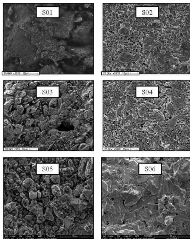
Figura 7.1.2: Imágenes SEM para las muestras S01 a S06.
