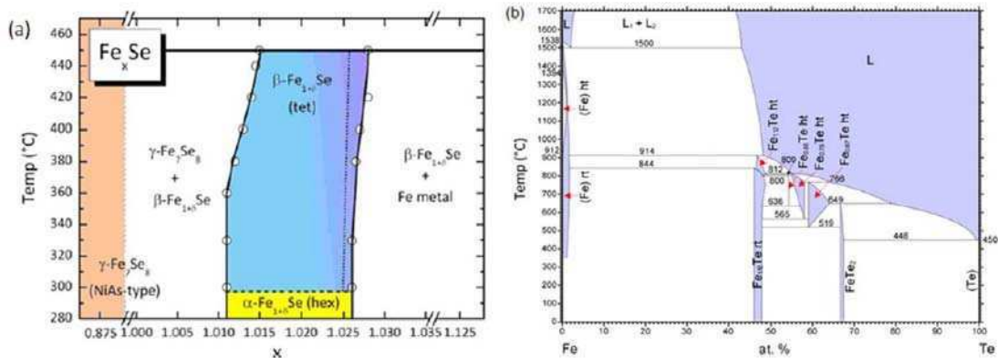
Figura 1.3.3: a) Diagrama de fases para el compuesto \text{Fe}_x\text{Se} [1.3.6]; b) Diagrama de fases para el compuesto \text{FeTe} [1.3.7].
