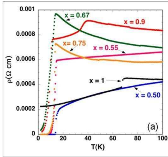
Figura 1.2.2: Curva de \rho en función de la temperatura para la familia \text{Fe}_{1+y}\text{Te}_x\text{Se}_{1-x} para diferentes valores de x [1.2.5].
