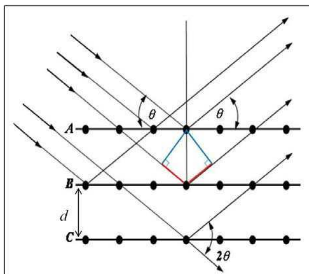
Figura A.1: Esquema de la reflexión de Bragg, con una distancia interplanar d .
