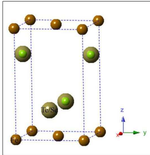
Figura 8.1.5: Esquema de la estructura cristalográfica para el cristal FTSe2.
