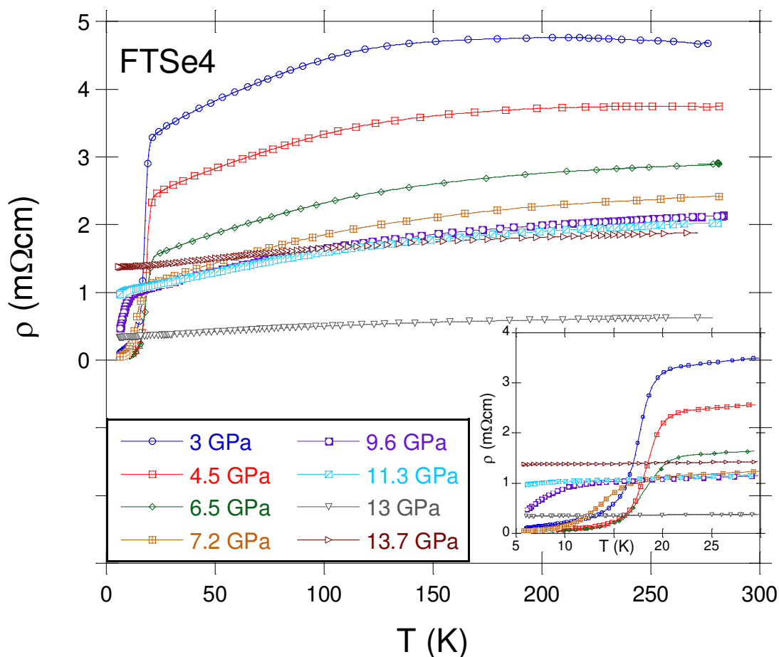
Figura 8.3.3: \rho vs T a distintas presiones para el cerámico FTSe4. En la figura insertada se muestra el detalle de la transición superconductor.
