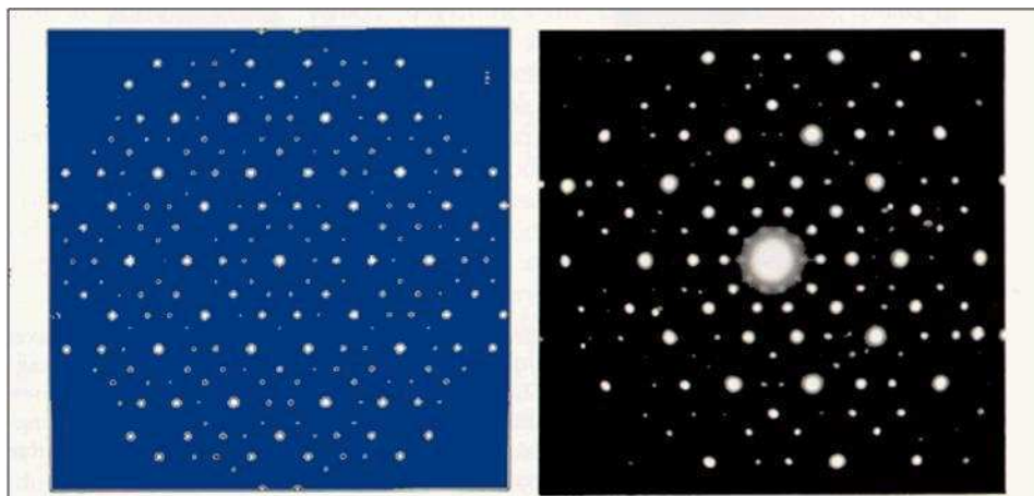
Figura A.2: Comparación del patrón de difracción de un cristal observado (der.) con el calculado (izq.) [A.2] .
