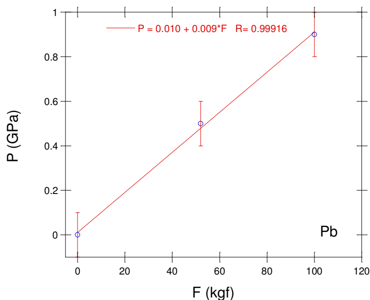
Figura 6.3.1.2: Curva de calibración P vs F para el Pb.
