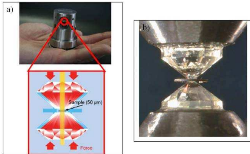
Figura 6.2.2: a) Esquema de la aplicación de la fuerza con los yunques de diamantes sobre la muestra; b) Imagen de los yunques de diamantes y el gasket [6.2.1] .
