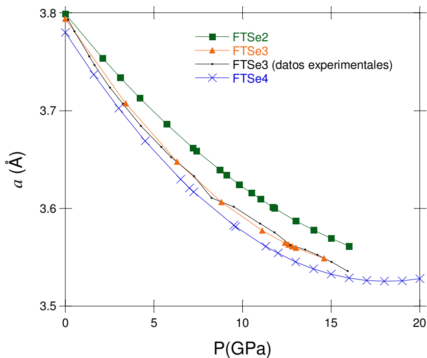
Figura 9.5: a vs P para las muestras FTSe2, FTSe3 y FTSe4 calculados a través del modelo de T_c [ver ec. (9.1)] y b(a) (ver fig.9.2).
