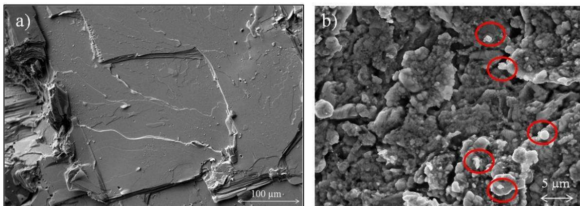
Figura 8.1.3: a) Imagen SEM del cristal FTSe2; b) Imagen SEM del cerámico FTSe4.
