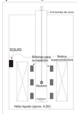
Figura D.1: Esquema del magnetómetro SQUID
