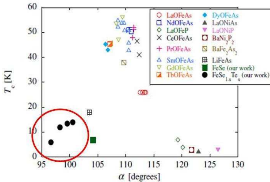
Figura 1.1.5: T_c vs \alpha tanto para los nitrogenoides como los calcogenuros basados en Fe.
