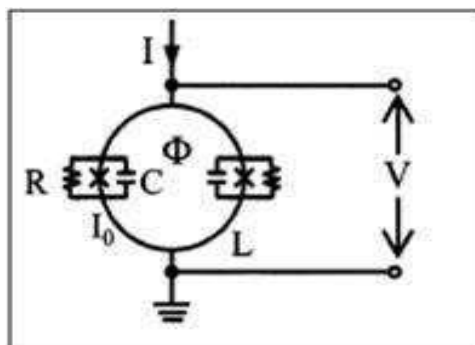
Figura D.2: Circuito del SQUID [D.2]
