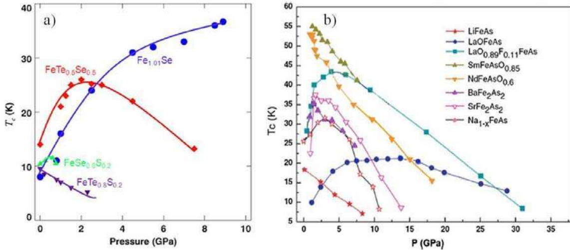
Figura 1.4.1: T_c en función de la presión externa. a) Familias de calcogenuros de Fe [1.4.1] b) Familias de nitrogenoides de Fe [1.4.2] .
