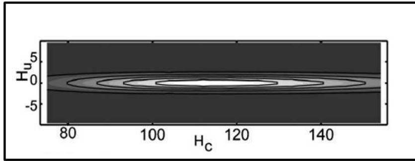
Figura 5.2.3: Diagrama FORC para un conjunto de partículas de un solo dominio no interactuantes.
