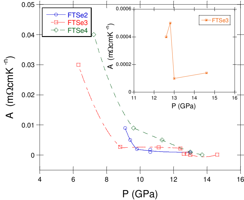
Figura 8.4.10: A vs P para FTSe2, FTSe3 y FTSe4, donde el coeficiente A se obtuvo del ajuste de \rho(T) mediante la ec. (1.5.1). En la figura insertada se muestra el detalle de evolución de A con presión para FTSe3, donde se puede observar un máximo local para presiones en la zona cercana a la reemergencia.
