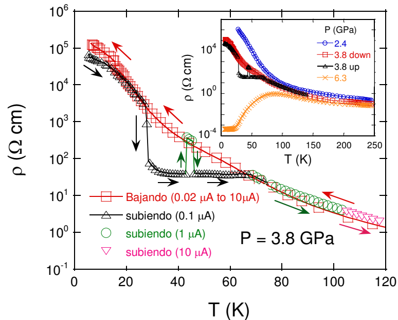
Figura 10.2: Resistividad del cristal GTS (muestra B) en función de la temperatura para presiones medidas en la región de coexistencia a 3.8 GPa y en un rango de temperatura de 4 K a 120 K. En la figura insertada se muestra toda la curva de \rho(T) para diferentes presiones (2.4 GPa para la muestra A y 3.8 y 6 GPa para la muestra B).
