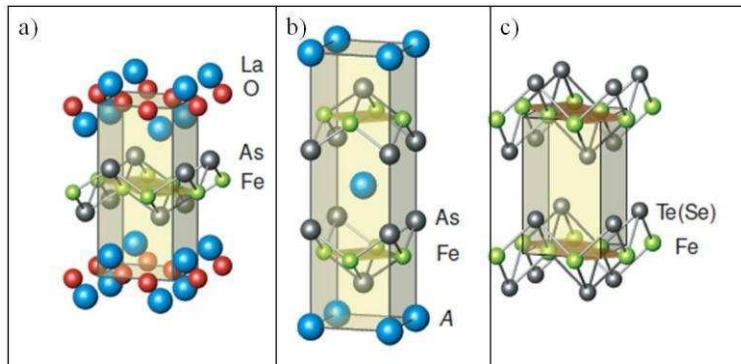
Figura 1.1.1: Ejemplos de estructuras de diferentes SCFe [1.1.1] : a) "1111", b) "122" y c) "11".
