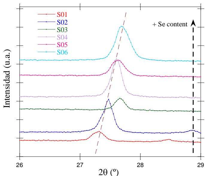
Figura 7.1.4: Reflexión (1,0,1) correspondiente al pico de mayor intensidad para las muestras S01-S06.
