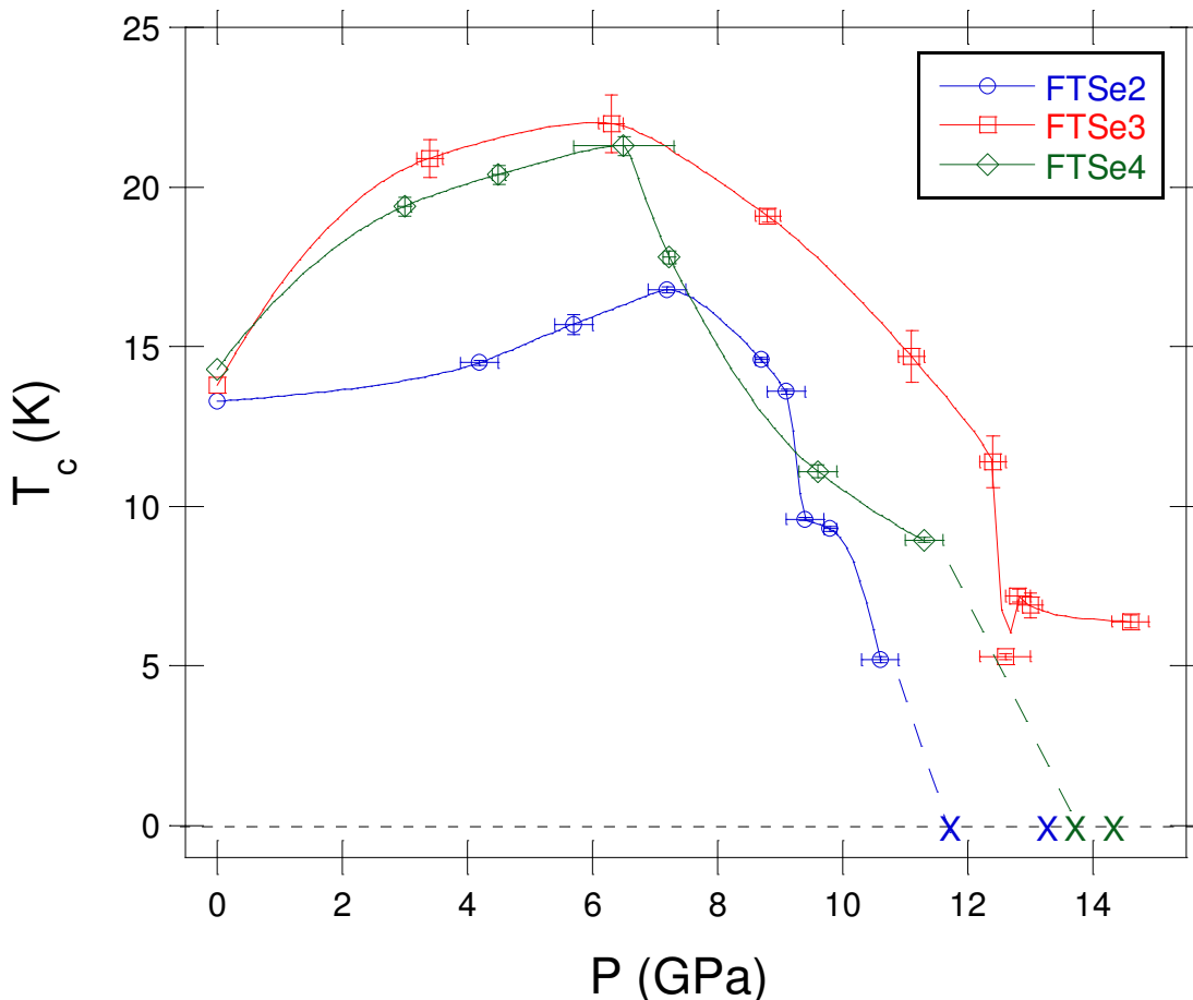
Figura 8.3.4: T_c vs P para los cristales FTSe2 y FTSe3 y el cerámico FTSe4.
