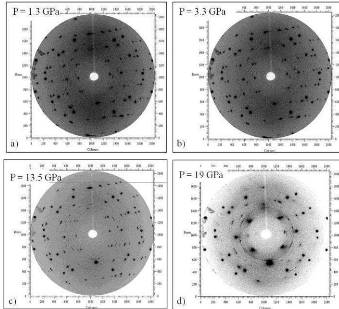
Figura 8.3.6: Espectros de difracción de cristal único para la muestra FTSe3 a distintas presiones: a) P = 1.3 GPa; b) P = 3.3 GPa; c) P = 13.5 GPa; d) P = 19 GPa.
