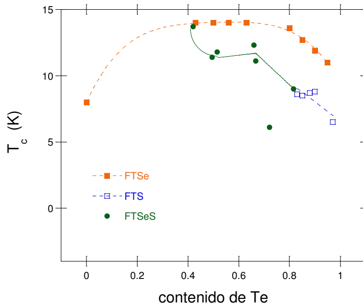
Figura 7.3.3: T_c en función del contenido de Te para las familias FTSe [7.3.4-7.3.7] , FTS [7.3.8] y FTSeS (nuestro trabajo).
