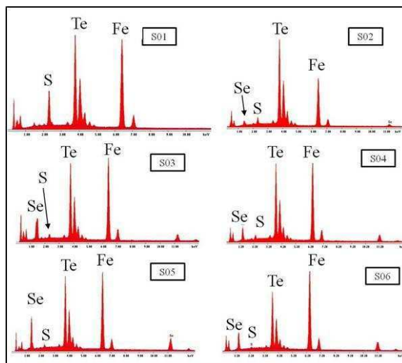
Figura 7.1.1: Espectros de EDX para las muestras S01 a S06.
