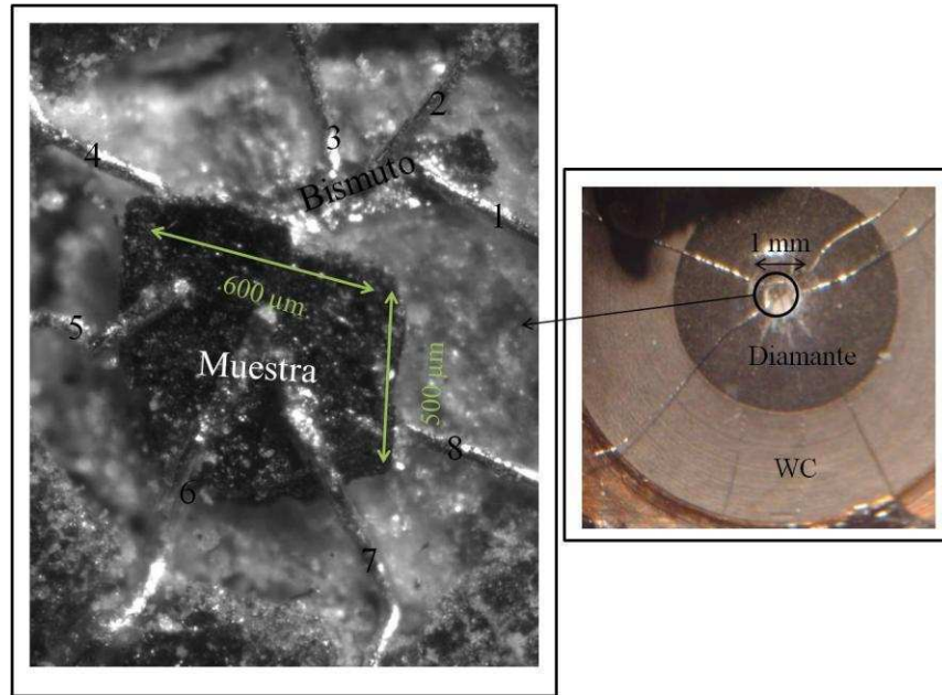
Figura 6.1.3: Foto del armado de la celda de alta presión, donde se distingue la superficie del diamante contenido en un disco de carburo de tungsteno (WC). Se exhibe el detalle la muestra con el manómetro utilizado (bismuto).
