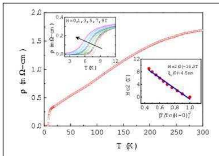
Figura 1.2.1: Curva de \rho en función de la temperatura para el compuesto \text{FeSe}_{0.88} [1.2.1] . En la figura insertada de la izquierda, se exhibe las mediciones de \rho(T) al aplicar diferentes campos magnéticos, H , por debajo de 12 K. En la figura insertada de la derecha se muestra la curva del campo crítico, H_{c2} , en función de la temperatura.
