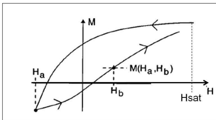
Figura 5.2.2: Esquema de medición de una curva FORC, donde H_a es el campo de inversión, H_b es un campo aplicado durante el proceso y M(H_a, H_b) es la magnetización medida en ese campo H_b con el correspondiente campo de inversión H_a .
