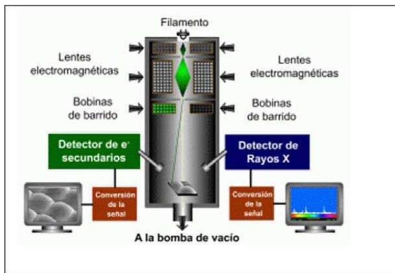
Figura B.2: Esquema del dispositivo de SEM y EDX [B.2] .
