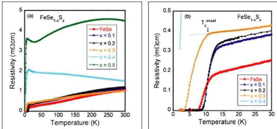
Figura 1.2.3: Curva de \rho en función de la temperatura para los compuestos de la familia \text{Fe}_{1+y}\text{Se}_{1-x}\text{S}_x [1.2.7] a) para todo el rango de temperatura; b) detalle cerca de la T_c .
