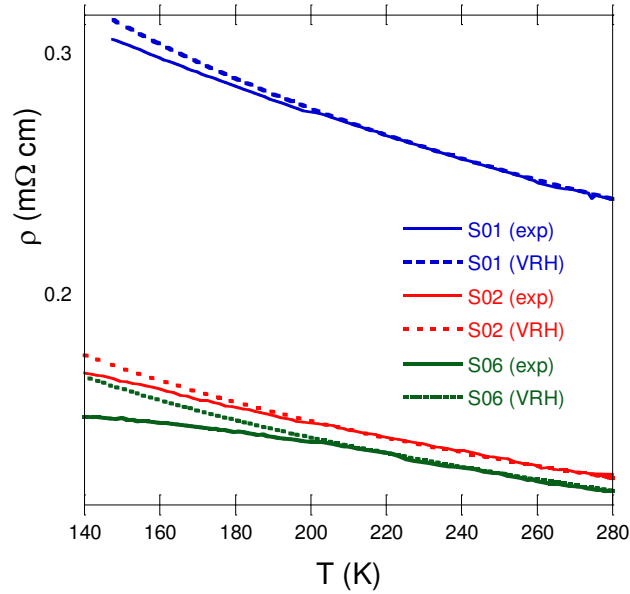
Figura 7.3.1: \rho vs T para las muestras S01, S02 y S06. La ley de VRH es la que mejor ajusta en el rango de temperaturas superiores a 200 K. Para valores menores de temperatura, los datos experimentales se desvían de esta ley.
