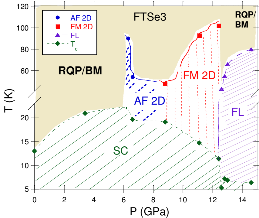
Figura 8.4.7: Diagrama de fases de T vs P para el cristal FTSe3 (las líneas que se utilizan para unir los puntos sirven para guiar al ojo).
