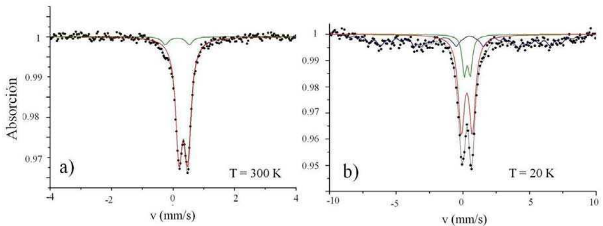
Figura 8.1.6: Espectros Mössbauer de la muestra FTSe4; a) Absorción vs velocidad a 4 mm/s y a temperatura ambiente; b) Absorción vs velocidad a 10 m/s y 20 K.
