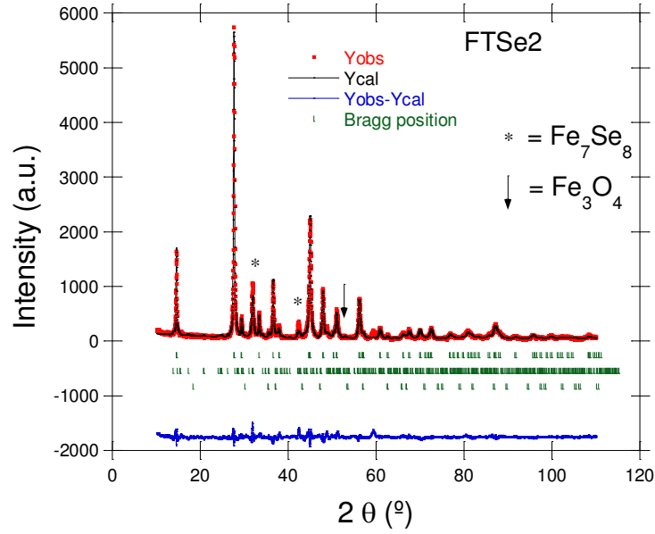
Figura 8.1.4: Difractograma del cristal FTSe2 (en rojo) y su correspondiente refinamiento Rietveld (línea negra). La diferencia entre los valores observados y los calculados se marcan con una línea azul y las líneas verticales verdes corresponden a las posiciones de Bragg.
