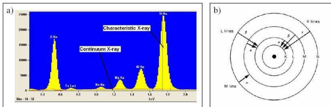
Figura B.1: a) Espectro típico medido con EDX, donde se muestra el espectro continuo y el pico característico de los rayos X; b) esquema de las capas atómicas con sus respectivos nombres [B.1] .
