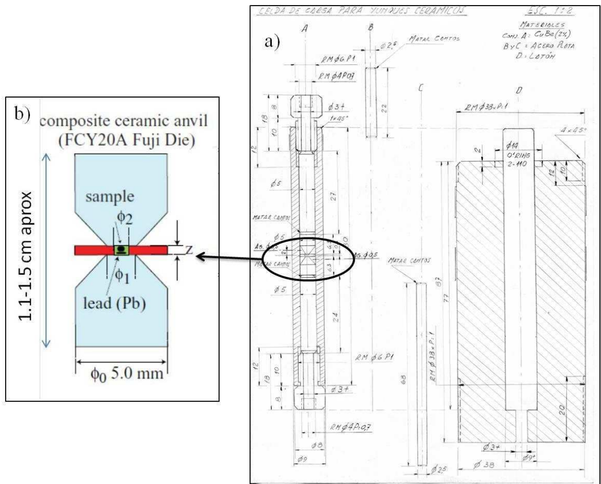
Figura 6.3.1: a) Esquema de la celda de alta presión para el SQUID; b) Detalle de los yunques y el gasket.
