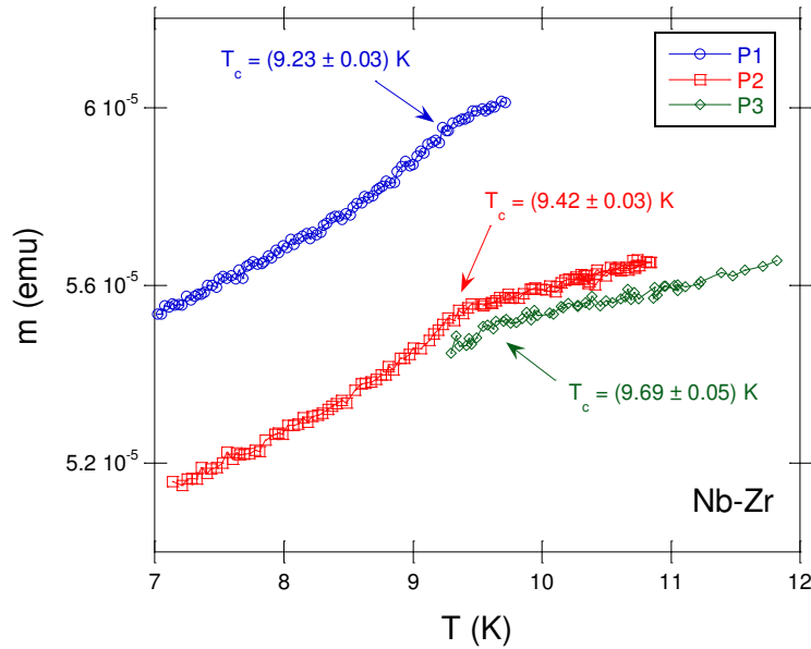
Figura 6.3.1.3: m vs T para el compuesto \text{Nb}_{0.40}\text{Zr}_{0.60} con tres presiones distintas.
