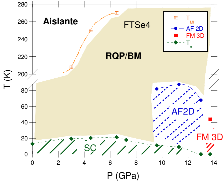
Figura 8.4.8 Diagrama de fases de T vs P para el cerámico FTSe4.
