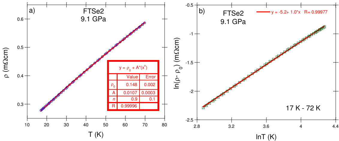
Figura 8.4.3: a) Resistividad en función de la temperatura con el ajuste según ec. (1.5.1); b) \ln(\rho - \rho_0) vs \ln T con el ajuste según la ec. (8.4.2) en 9.1 GPa.
