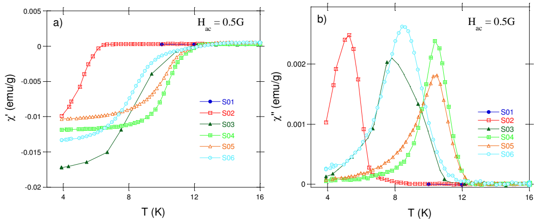
Figura 7.2.6: a) \chi' vs T ; b) \chi'' vs T para la familia FTSeS
