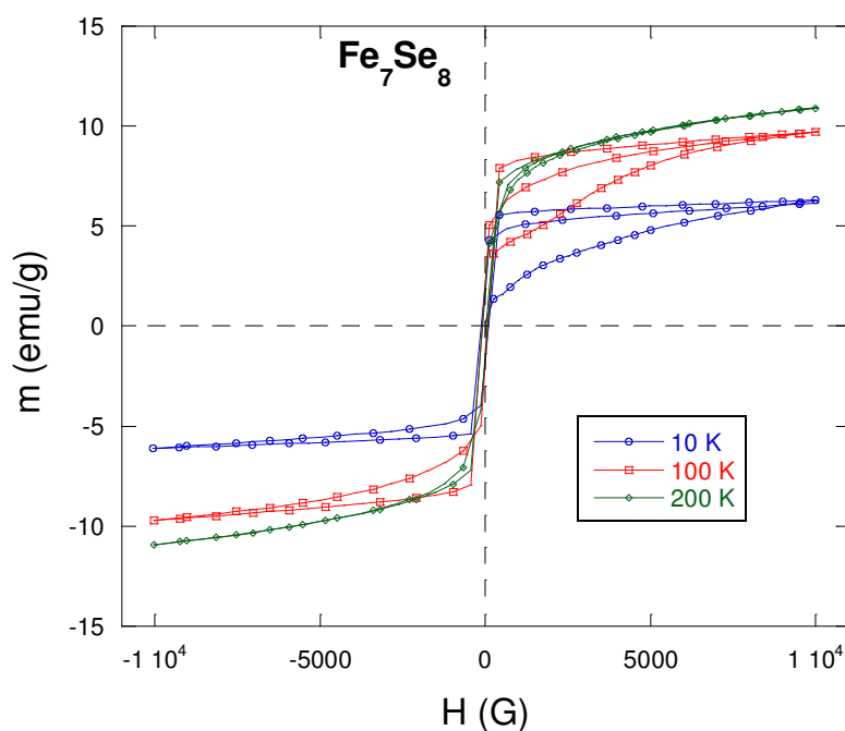
Figura 8.2.5: Curva m(H) para el compuesto Fe_7Se_8 .
