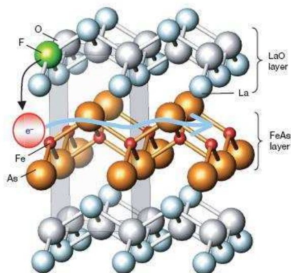
Figura 1.1.3: Esquema que muestra la transferencia de carga de los planos reservorios de carga a los planos de conducción para el compuesto LaOFeAs dopado con flúor en el sitio del oxígeno [1.1.6] .
