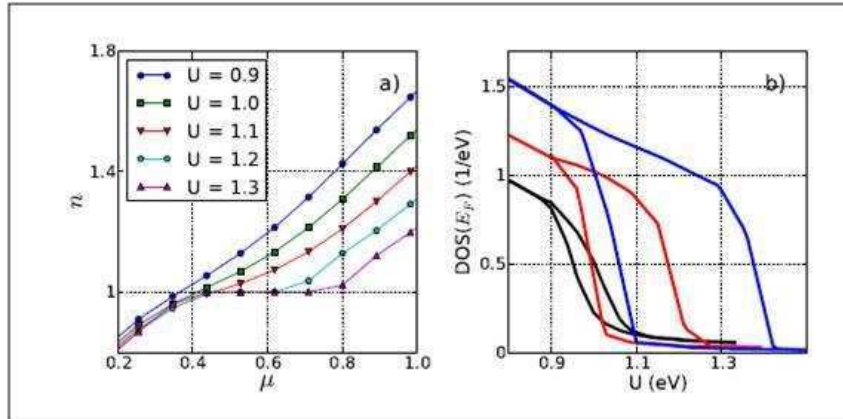
Figura 10.3: a) Número de ocupación ( n ) en la banda t_{2g} del compuesto GTS en función de potencial químico \mu y la interacción coulombiana local U , obtenidos con los cálculos de LDA+DMFT; b) La densidad de estados en la energía de Fermi como función de U para n=1 a T=58, 116 y 232 K (desde arriba hacia abajo), indicando la coexistencia de soluciones.
