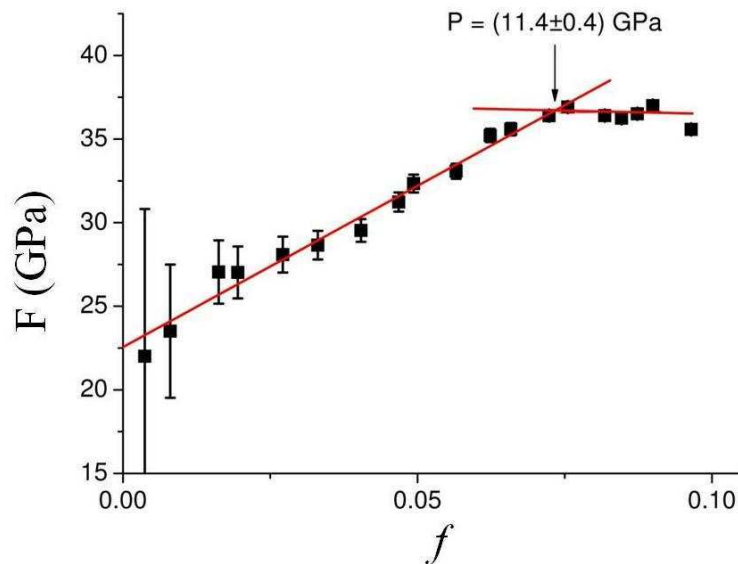
Figura 8.3.8: Fuerza normalizada, F , en función de la fuerza euleriana, f , para el cristal FTSe3.
