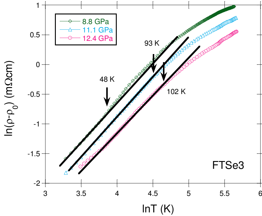
Figura 8.4.6: Curvas \ln(\rho-\rho_0) vs \ln T para las presiones 8.8 GPa, 11.1 GPa y 12.4 GPa en FTSe3. Las rectas indican una dependencia del tipo \rho = \rho_0 + AT^n con n = 1.3 . Las flechas marcan la temperatura hasta donde es válida esta dependencia.
