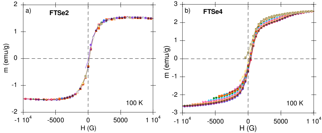
Figura 8.2.3: Curvas FORC para la muestra FTSe2 (a) y FTSe4 (b).
