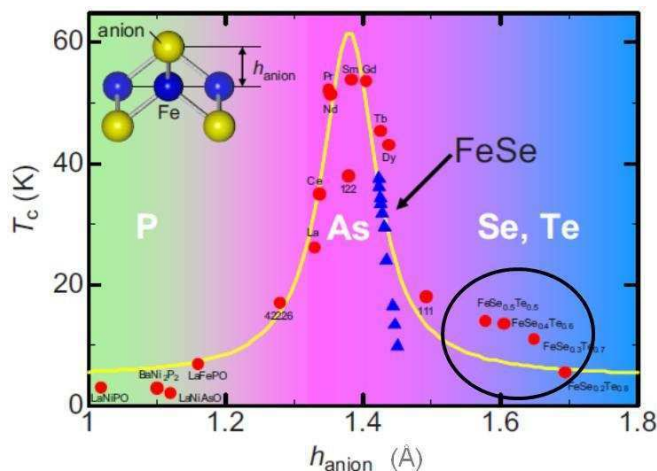
Figura 1.1.6: Curva Lorentziana, marcada con amarillo, publicada por H. Okabe et al [1.1.8] . Dentro de la figura se marca con un círculo negro los compuestos pertenecientes a la familia FTSe que no se pueden ajustar con la Lorentziana. Además, se muestra gráficamente la definición de distancia al anión, h_a .
