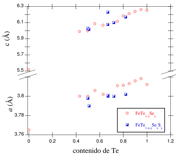
Figura 7.1.5: Parámetros a y c en función del contenido de Te para las muestras de FTSeS. Para comparar se agregan las muestras de la familia \text{FeTe}_{1-x}\text{Se}_x (FTSe) de la bibliografía [7.1.5 - 7.1.8].
