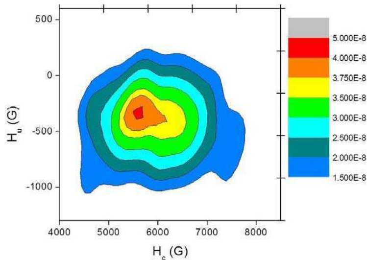
Figura 8.2.4: Diagrama FORC para la muestra FTSe4. Los valores de la escala son en unidades arbitrarias ya que se trata de la función de distribución (ver apéndice E).
