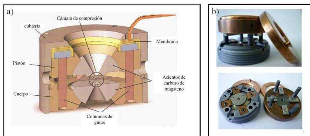
Figura 6.2.1: a) Esquema del DAC donde se detallan las partes que lo componen; b) Imágenes del cuerpo de la celda de 50 mm de diámetro y 32 mm de alto [6.2.1] .
