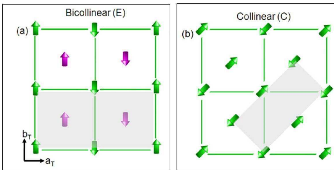
Figura 1.2.5: a) Esquema de la estructura de espín bicolineal (tipo E) para los compuestos 11; b) Estructura magnética colineal (del tipo C) para la mayoría de los SCFe. En ambas figuras se representa la celda unidad con el color gris [1.2.12] .
