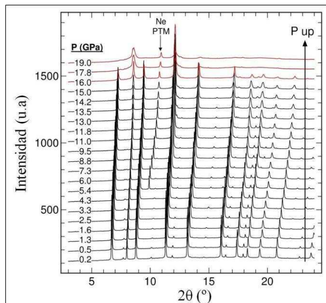
Figura 8.3.5: Intensidad en función del ángulo 2\theta para el cristal FTSe3 a distintas presiones.
