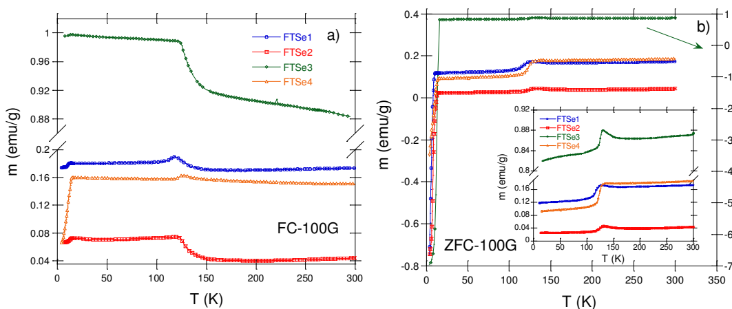
Figura 8.2.1: a) m vs T FC a 100 G para los cuatro compuestos; b) m vs T ZFC a 100 G. En la figura insertada se muestra en detalle la región normal para la curva medida con el protocolo ZFC.
