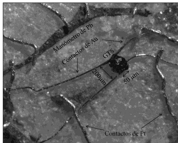
Figura 6.1.4: Muestra GTS, con los correspondientes contactos y el manómetro de plomo.
