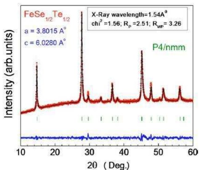
Figura 4.1: Difractograma y refinamiento para el compuesto FeSe_{0.5}Te_{0.5} [4.2] .
