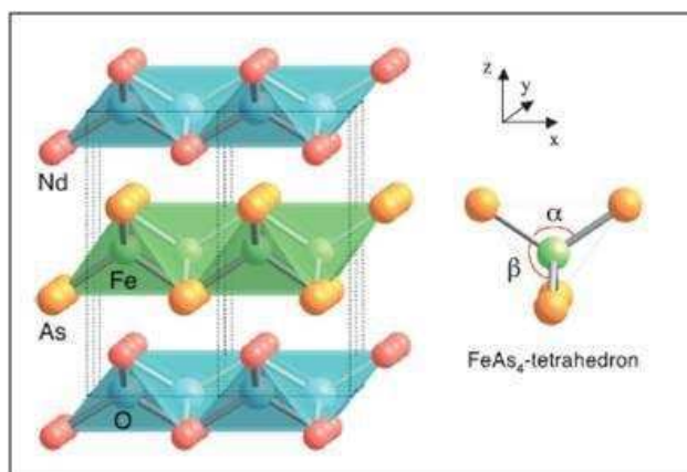
Figura 1.1.2: Estructura tetragonal del compuesto NdFeAsO junto con los ángulos relevantes [1.1.5]
