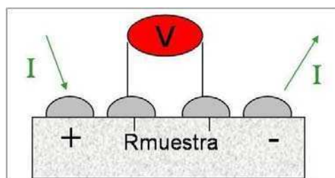
Figura 6.1.1: Esquema del método de medición a cuatro terminales.
