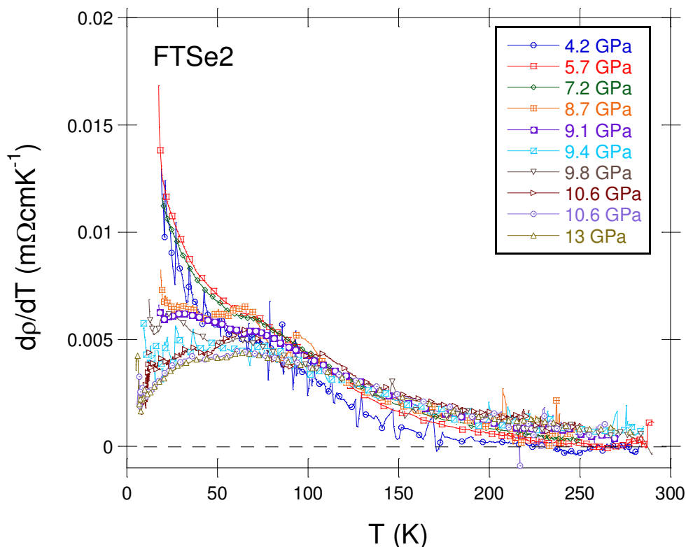
Figura 8.4.1: Curva d\rho/dT vs T para el cristal FTSe2 a distintas presiones.
