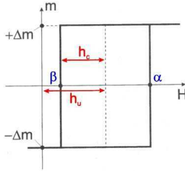
Figura E.1: Esquema de un histérón correspondiente al modelo de Preisach
