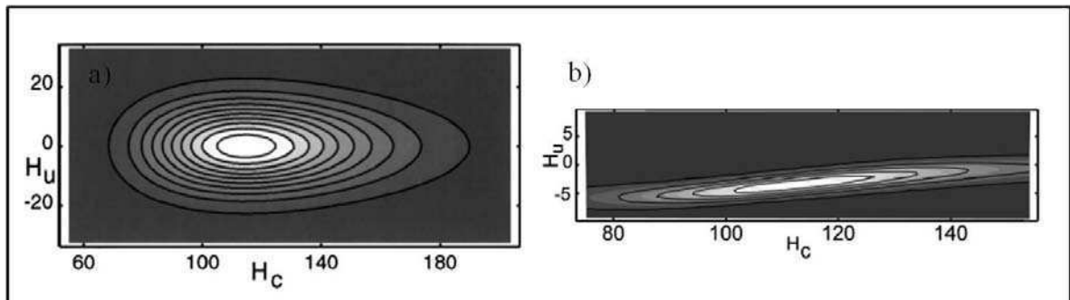
Figura 5.2.4: a) Diagrama FORC para un conjunto de partículas de un solo dominio interactuantes mediante un campo de interacción local. b) Diagrama de FORC para un conjunto de partículas monodominio interactuantes mediante un campo de interacción medio.
