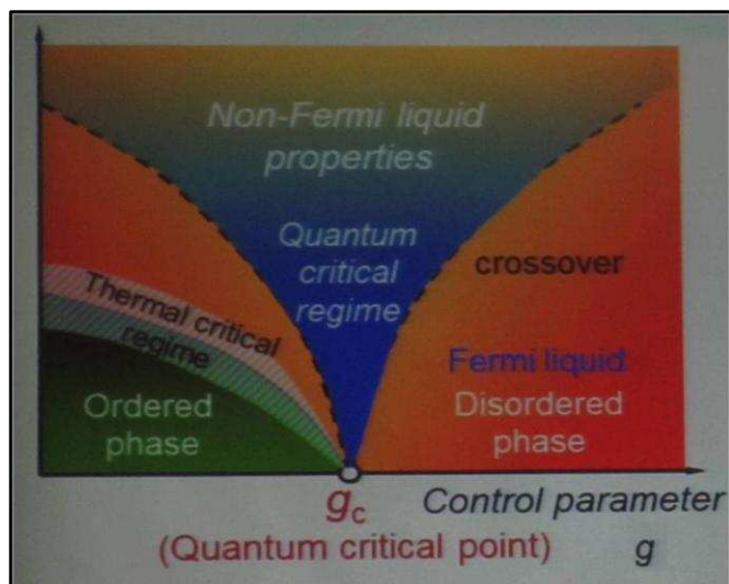
Figura 1.5.1: Esquema de un diagrama de fases típico en la cercanía de un QCP [1.5.2] .
