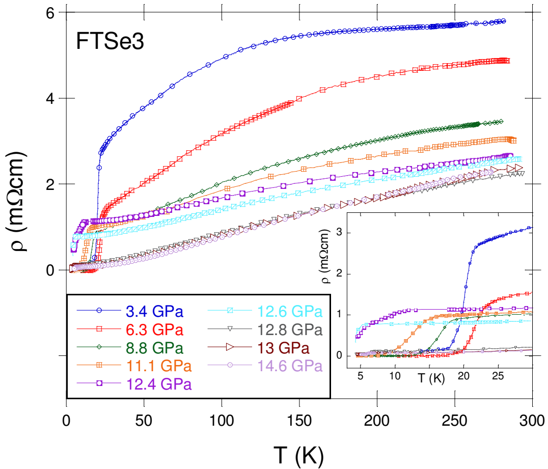
Figura 8.3.2: \rho vs T a distintas presiones para el cristal FTSe3. En la figura insertada se observa un detalle para las temperaturas cercanas a la T_c .
