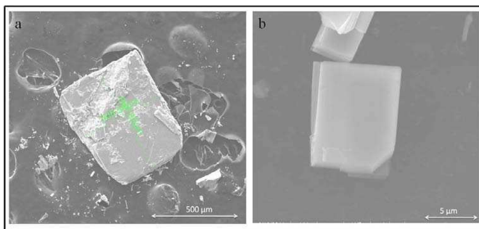
Figura 8.1.1: a) Imagen SEM del cristal FTSe3. b) Detalle de un cristal más pequeño del mismo lote, donde se puede observar la característica de “twin” del mismo.
