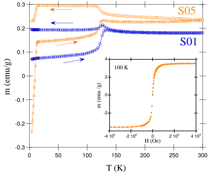
Figura 7.2.4: m vs T con ZFC y FC para las muestras S01 y S05, medidas a 100 G. En la curva insertada se muestra m vs H para S05 medida a 100 K.
