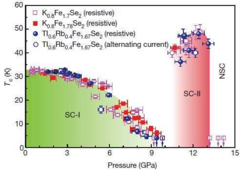
Figura 1.4.2: T_c en función de la presión externa para la familia A_{1-x}Fe_{2-y}Se_2 [1.4.4], donde se observa la reemergencia
