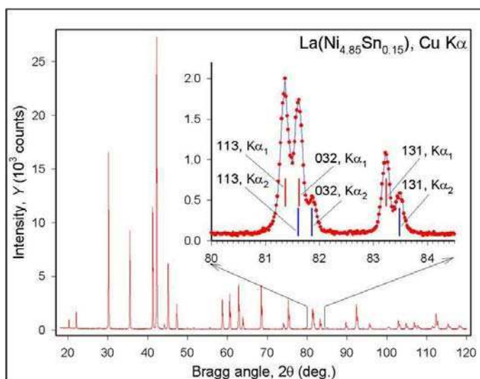
Figura A.3: Difractograma de la muestra \text{La}(\text{Ni}_{4.85}\text{Sn}_{0.15}) [A.3] .
