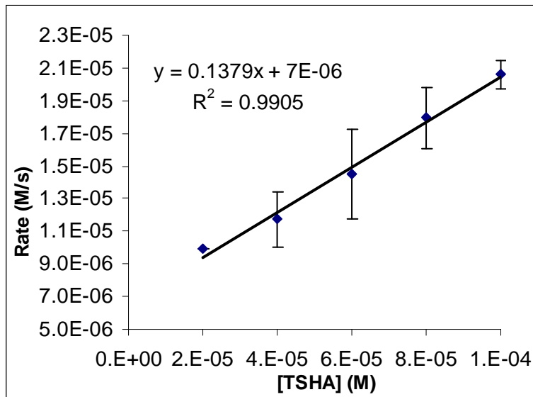
Figura 7. Velocidad inicial para la conversión de \text{Fe}^{\text{III}}\text{TMPyP } 5 \times 10^{-6} \text{ M} a \text{Fe}^{\text{II}}\text{TMPyP-NO} (M/s) vs. [TSHA] a pH 10 (buffer fosfato, 25^{\circ}\text{C} ).
