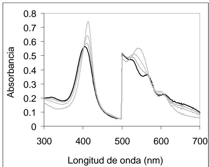
Figura 1B. Cambios espectrales correspondientes a la conversión de \text{Fe}^{\text{III}}\text{TPPS} 5 \times 10^{-6} M, (trazo negro, \lambda_{\text{max}}=403\text{nm} ) a \text{Fe}^{\text{II}}\text{TPPS-NO} (trazo gris \lambda_{\text{max}}=415\text{nm} ) en buffer fosfato a 25^{\circ} C. La región 500-700 nm está ampliada 5 veces para observar las bandas Q.
