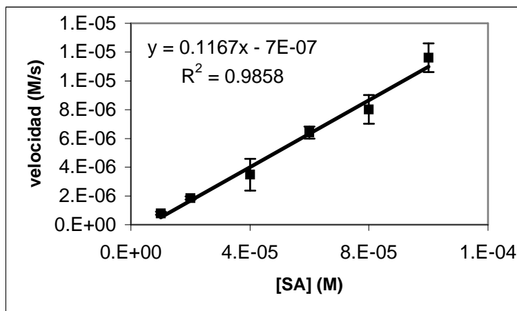
Figura 6. Gráfico de velocidad inicial de conversión de \text{Fe}^{\text{III}}\text{TMPyP } 5 \times 10^{-6} \text{ M} a \text{Fe}^{\text{II}}\text{TMPyP-NO} (M/s) vs concentración de SA (M). ( pH 7 buffer fosfato, 25^{\circ}\text{C} ).
