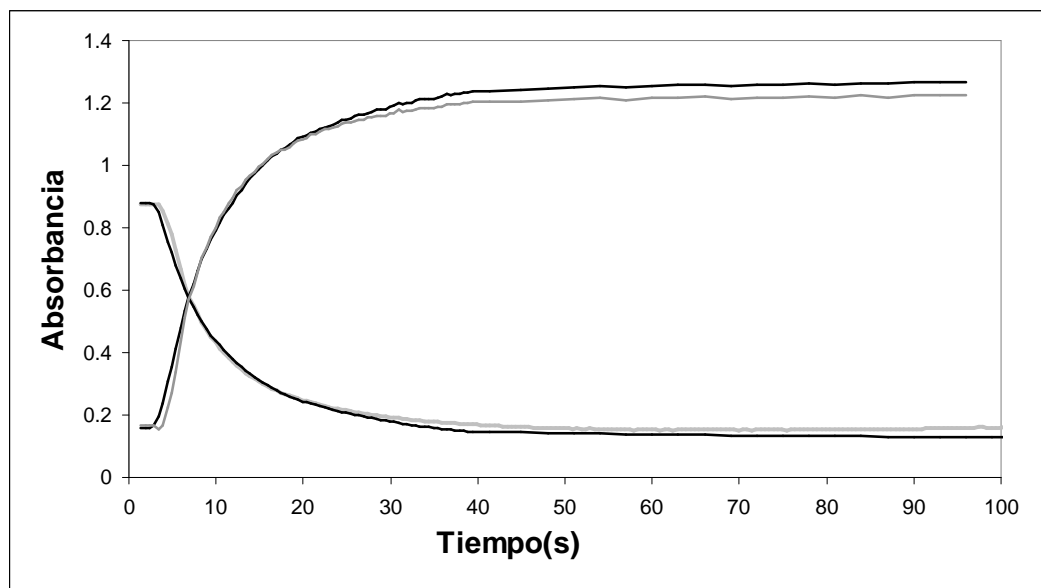
Figura 3. Absorbancia en función del tiempo para Mn^{III}TEPyP (454 nm) y Mn^{II}TEPyP-NO (422 nm), en la reacción de Mn^{III}TEPyP con SA en atmósfera de argón (negro) y en presencia de oxígeno (gris).
