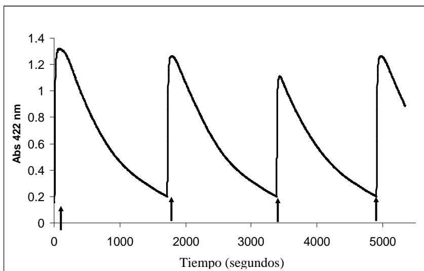
Figura 5. Absorbancia de Mn^{II}TEPyP-NO (422 nm) para la reacción de Mn^{III}TEPyP con SA/TSHA en aire. Las flechas indican cada agregado de SA.
