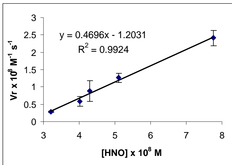
Figura 13. Velocidad inicial observada vs [HNO] estimada. (pH 10 buffer fosfato 0.1 M, 25 °C), para la reacción de \text{Mn}^{\text{III}}\text{TPPS} ( 5 \times 10^{-6} M) con TSHA.
