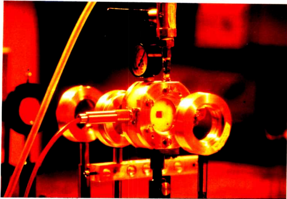
Figura 1: a) Esquema básico del dispositivo experimental. b) Detalle del cristal en su cápsula.
