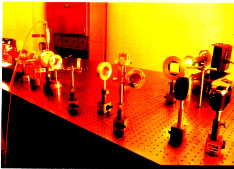
Figura IV.3: b) Fotografía del montaje experimental.
