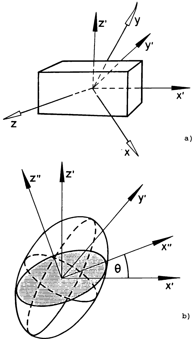
Figura II.3: a) Sistema de coordenadas OXYZ paralelo a los ejes propios del medio y OX'Y'Z' fijo a la lámina. b) Ejes propios del medio y dirección de las líneas neutras de la lámina.
