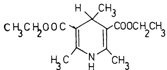
3,5-dietoxicarbonil-1,4-dihidrocolidina (DDC).
