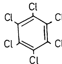
Hexaclorobenceno (HCB)
