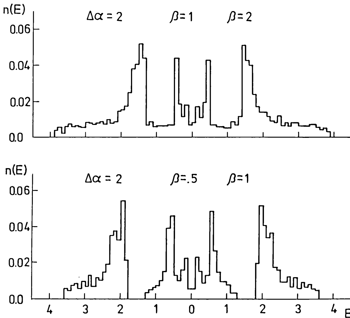
FIGURA VII.12: n(E) para dos ejemplos tridimensionales, incommensurados según una sola dirección. La celda unidad correspondiente es la que aparece en la figura VII.11. En ambos casos Q/2\pi = 10/33 .
