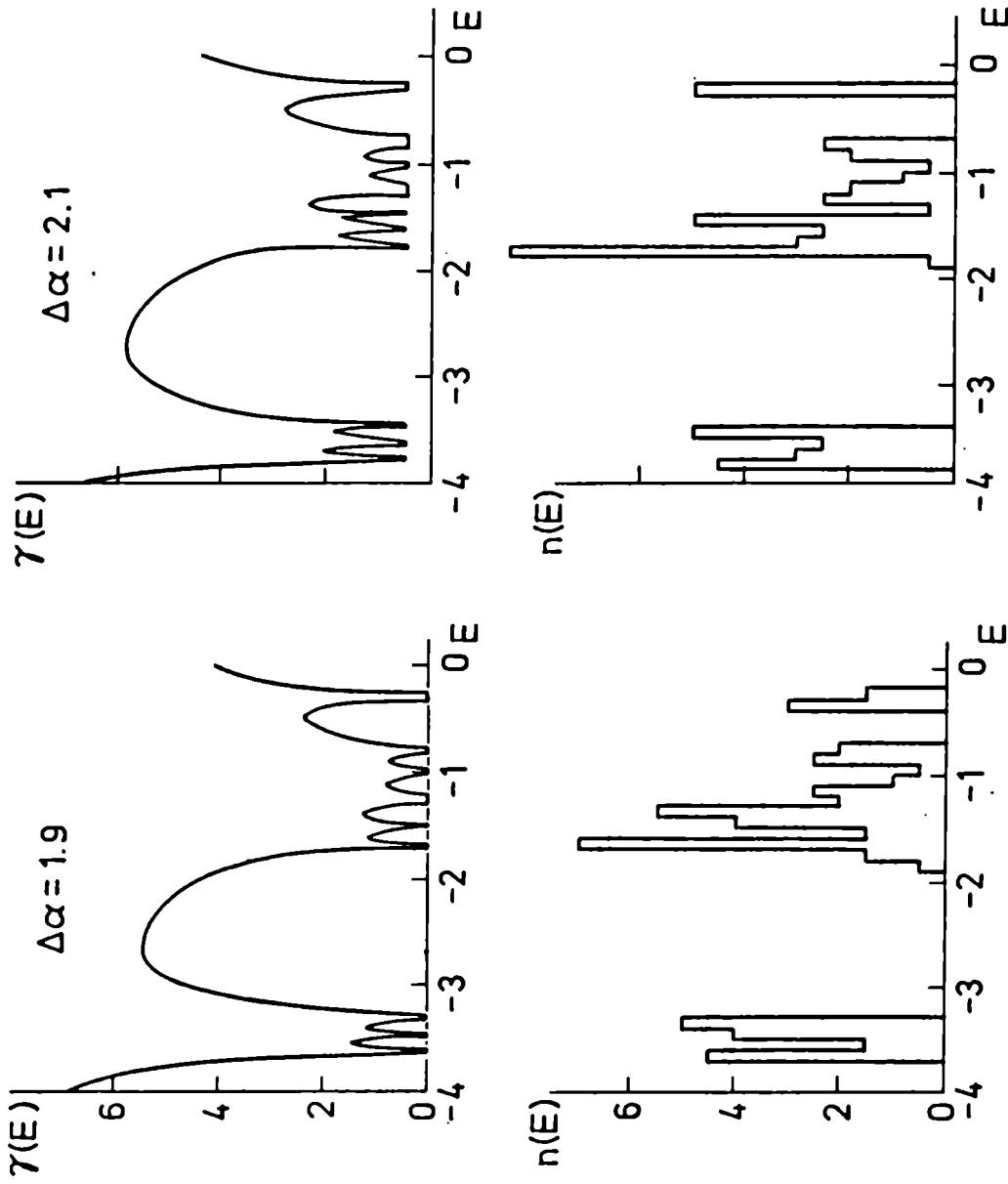
FIGURA VIII.3: n(E) y \gamma(E) para dos ristraes en fase para dos valores de \Delta\alpha , para la mitad de la banda. Q/2\pi=(\sqrt{13}-3)/2 , \beta_1=\beta_2=1 .
