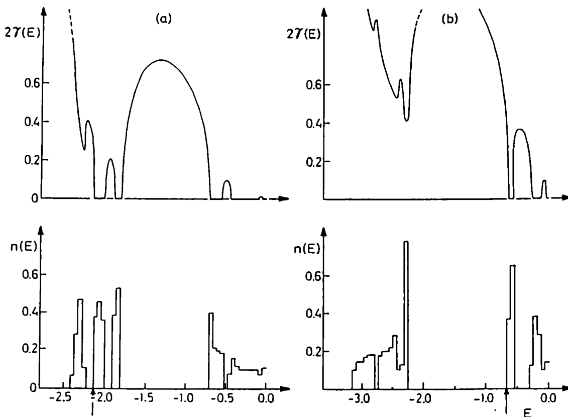
FIGURA V.2: n(E) y \gamma(E) para la modulación tipo zigzag para la mitad de la banda de energías y r=3 en ec. (2.16). (a) \Delta\alpha= 1.5 , (b) \Delta\alpha= 2.5 El borde de movilidad está indicado con una flecha.
