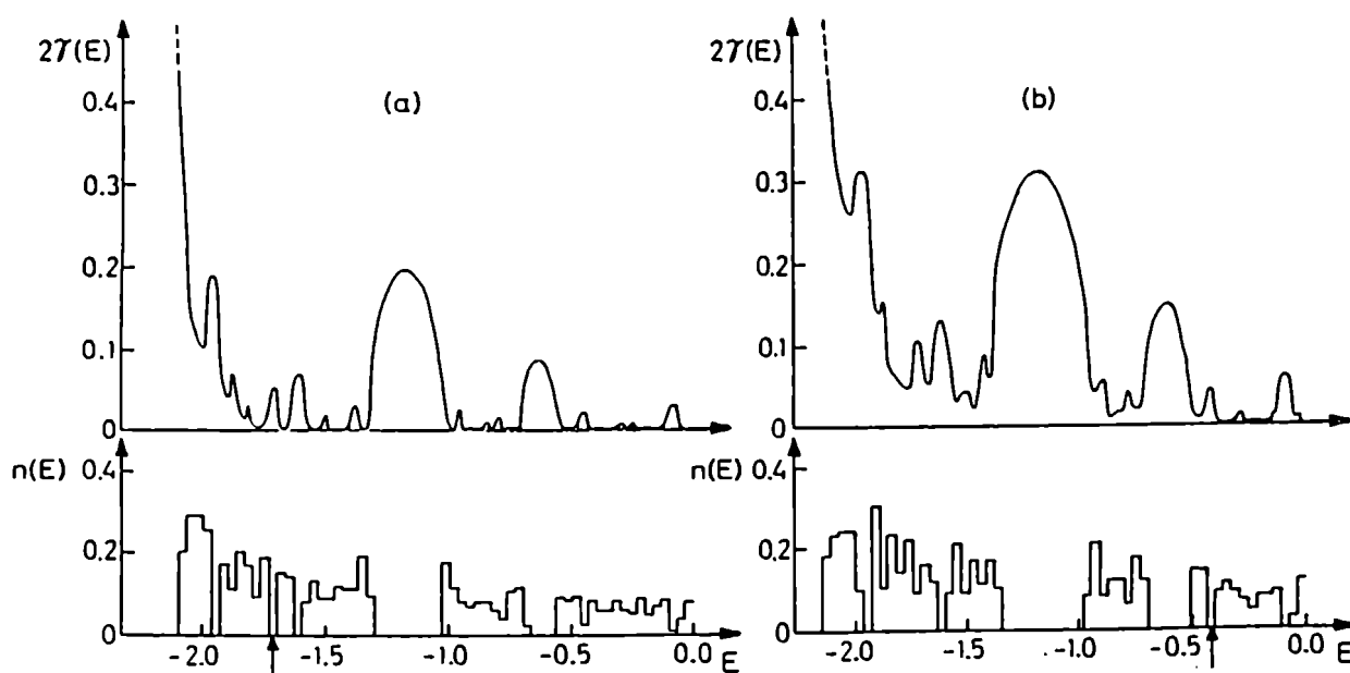
FIGURA V.3: n(E) y \gamma(E) para la modulación tipo diente de sierra para la mitad de la banda de energías y r=3 en ec. (2.16). (a) \Delta\alpha=.5 , (b) \Delta\alpha=.8 . El borde de movilidad se indica con una flecha.
