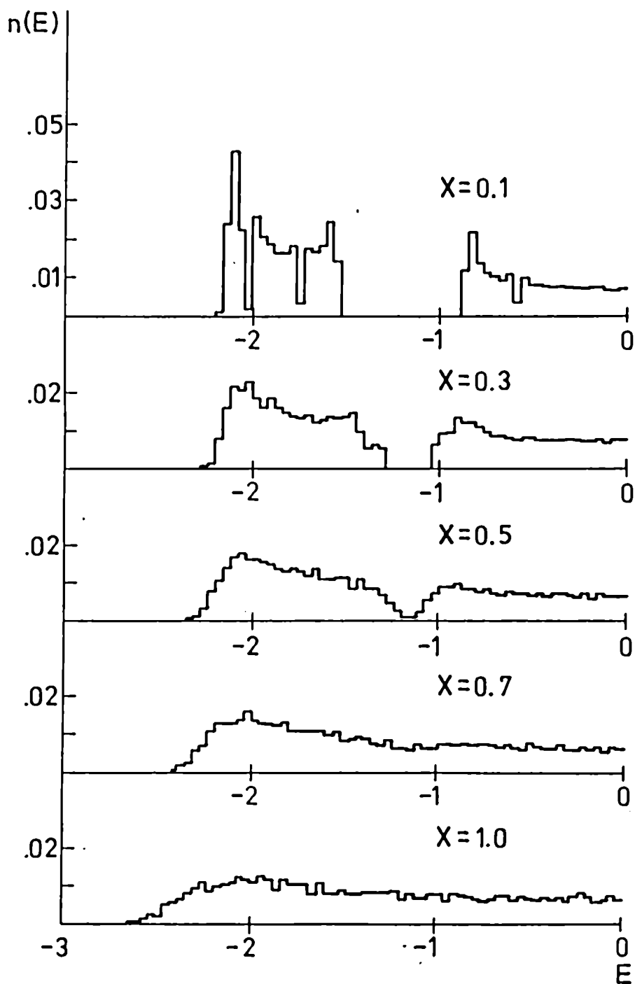
FIGURA III.1: Densidad de estados, n(E) , para r=3 en ec. (2.16), \Delta\alpha=1. , y t\neq 1 como función del grado de desorden, x , para el desorden tipo uniforme introducido en el modelo zigzag.
