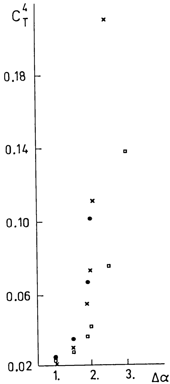
FIGURA VIII.2: C_T^4 en función de \Delta\alpha . Los puntos negros corresponden al modelo unidimensional con modulación coseno, las cruces al sistema formado por dos ristras en fase y los cuadrados a dos ristras en antifase.
