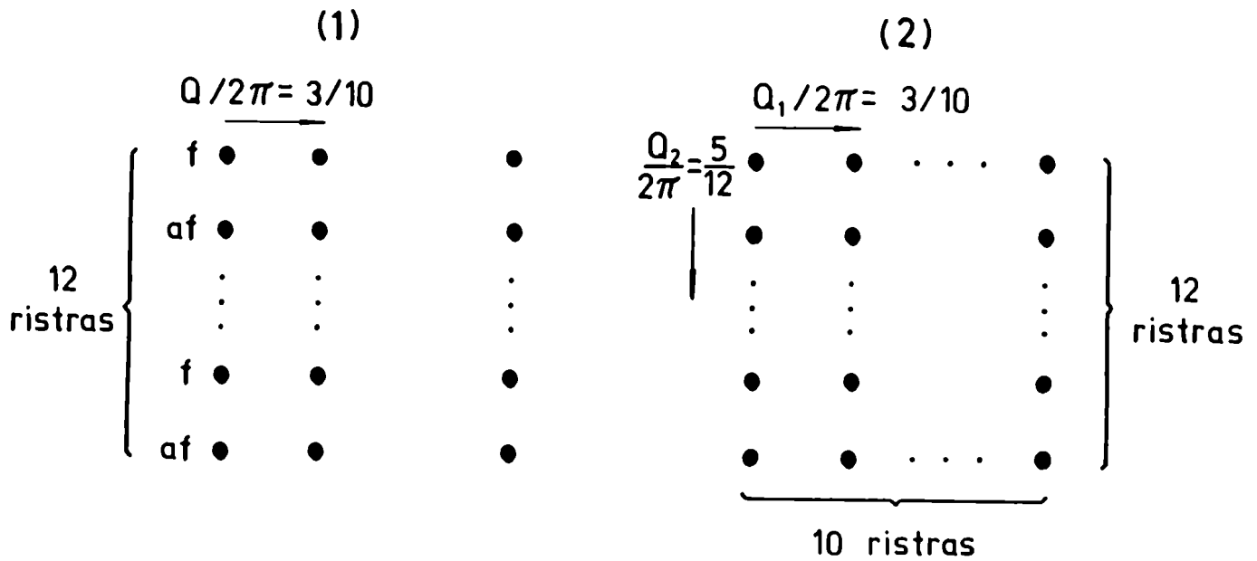
FIGURA VII.9: (1) Sistema en antifase (f:fase, af=antifase), formado por 12 ristras según "y" y 10 según "x". La modulación según "x" viene dada por Q/2\pi:3/10 .
