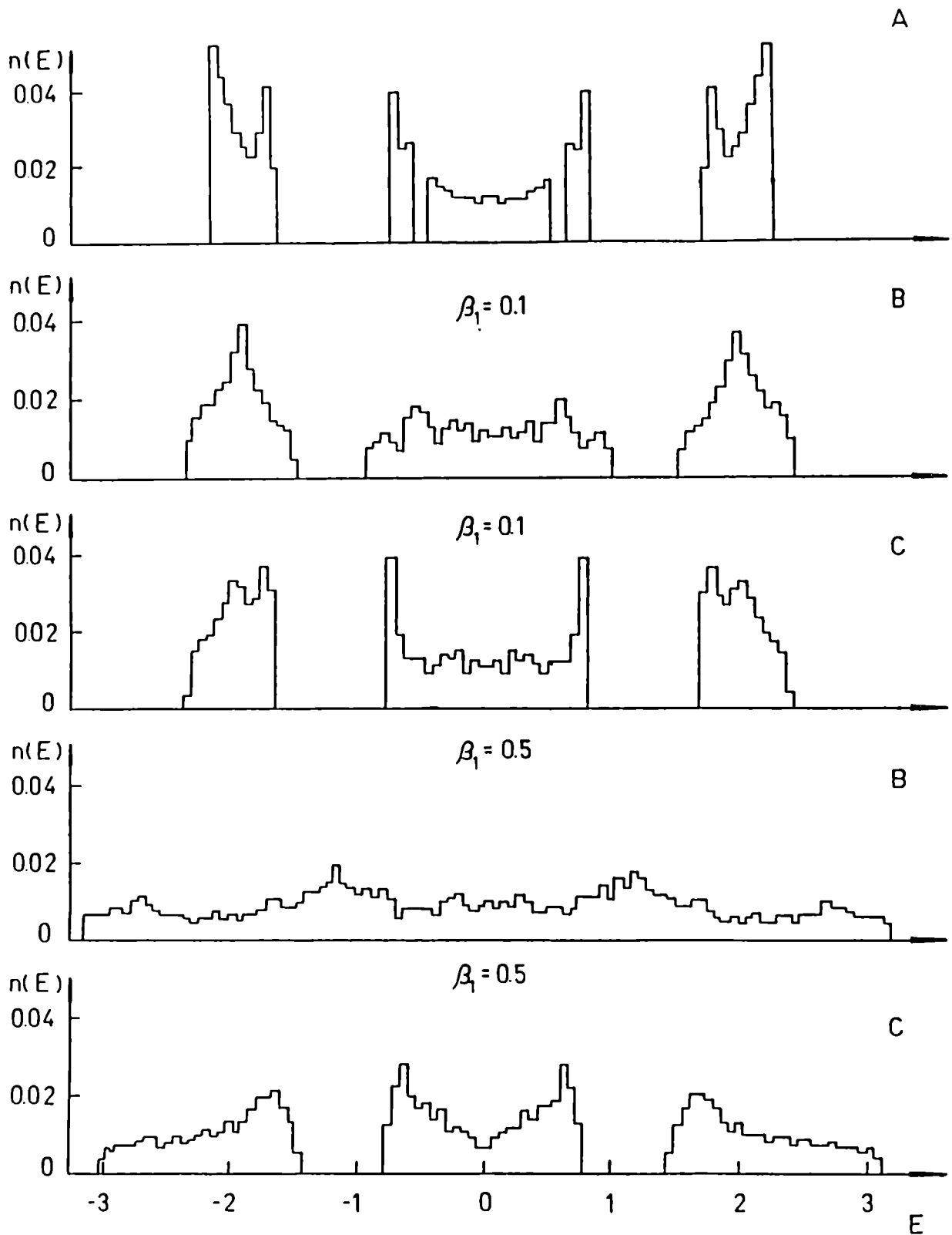
FIGURA VII.4: n(E) para: (A) cadena unidimensional con modulación tipo coseno (B) modelo bidimensional en fase, (C) modelo bidimensional en antifase. \Delta\alpha = \beta_2 = 1 . y Q/2\pi = (\sqrt{13} - 3)/2 .
