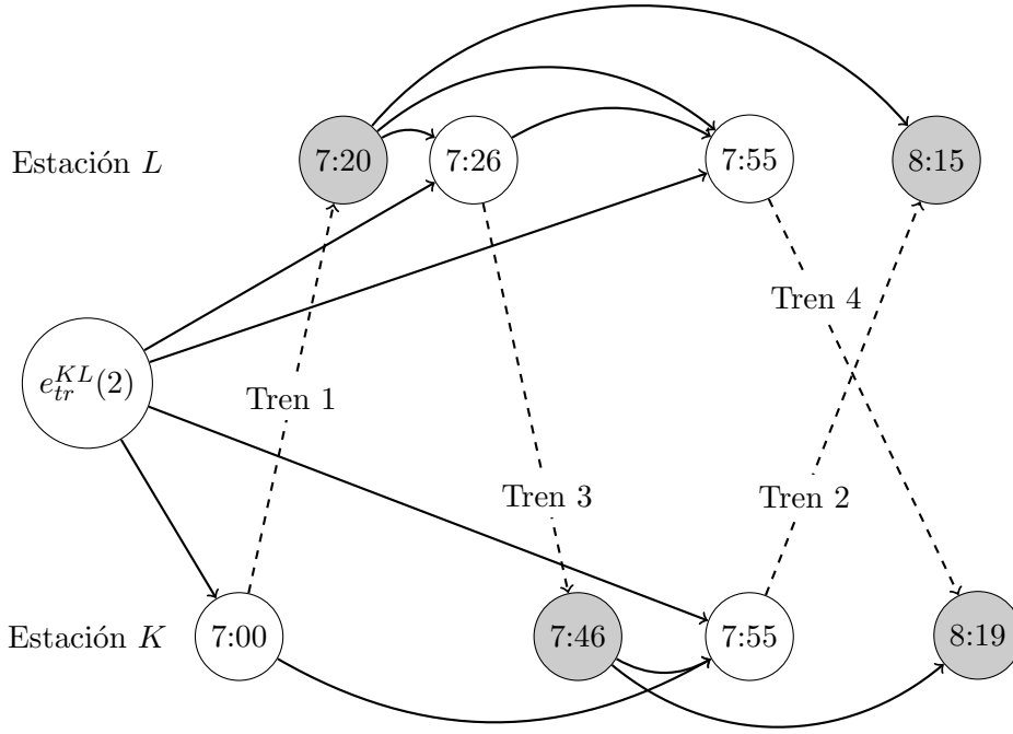
Fig. 3.4: Eventos y actividades relacionadas con el recurso de vías de tramo para el tramo (K, L) del cronograma ejemplo 3.1. Los eventos se organizan horizontalmente según su horario programado y verticalmente según su estación correspondiente. Los eventos correspondientes a salidas son blancos y los arribos grises. Las actividades del recurso de vías de tramo se dibujan con un eje normal mientras que las actividades de tren se dibujan con una línea punteada. El evento de inventario del tramo de vías se incluye a la izquierda y entre paréntesis figura su capacidad.
