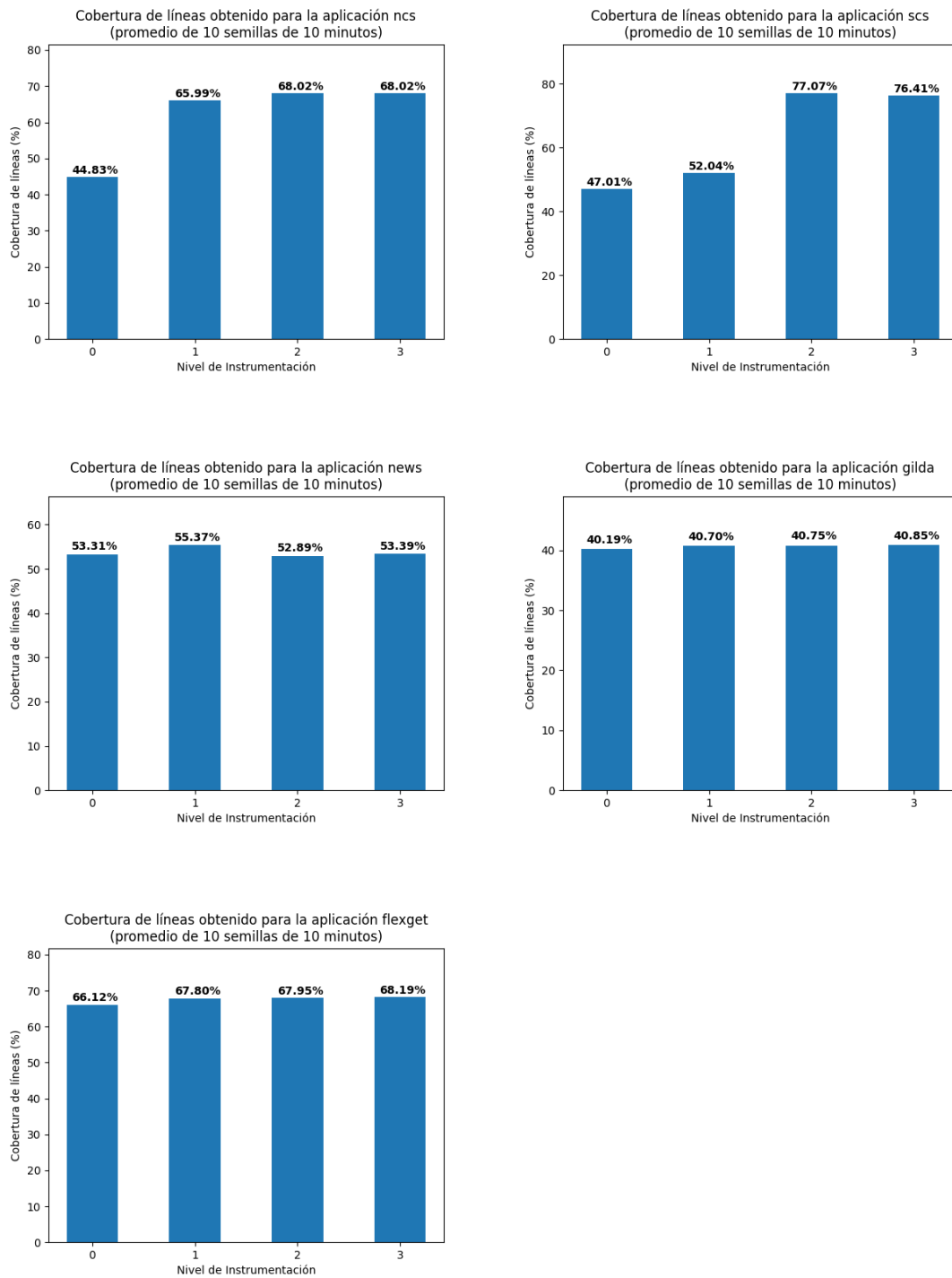
Fig. 4.1: Porcentaje de cobertura de líneas por aplicación para cada nivel de instrumentación
