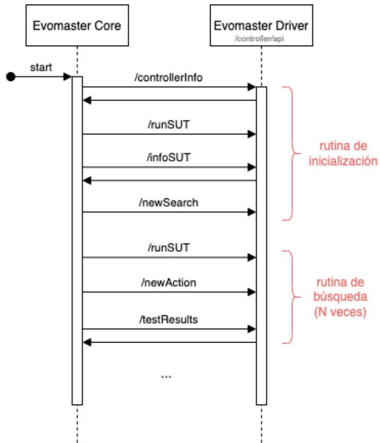
Fig. 3.1: Diagrama de secuencia del protocolo de comunicación de Evomaster
