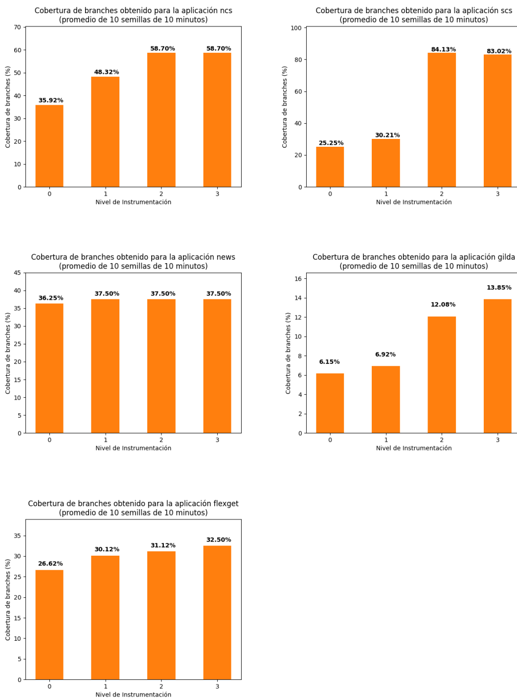
Fig. 4.2: Porcentaje de cobertura de branches por aplicación para cada nivel de instrumentación
