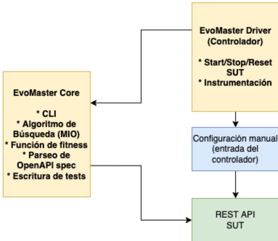
Fig. 2.1: Arquitectura de EvoMaster
