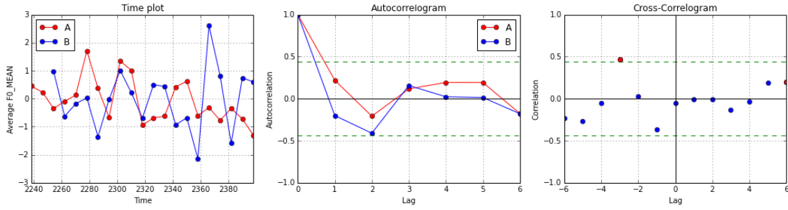
Fig. 2.6: Time-plot generado por el método TAMA, junto a su autocorrelograma y correlograma cruzado
