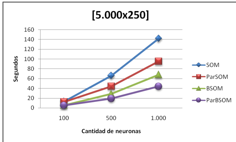
Figura 4.9: Tiempos para 5.000 muestras de dimensión 250
