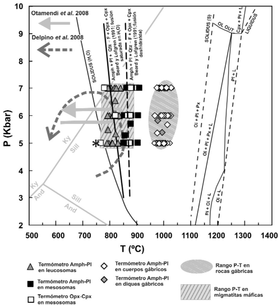
Figura 7: Diagrama P-T construido a partir de las condiciones de presión y temperatura inferidas a partir de las rocas ígneas máficas y las migmatitas máfica. Curvas de reacción Amph + Pl + Qtz = líquido + Opx + Cpx saturada en H 2 O y por fusión deshidratada según Beard y Lofgren, (1991); Solidus (S) , liquidus y campos de cristalización de fases minerales para el sistema basáltico seco según Cohen et al. (1967). Solidus (H 2 O) para el sistema basáltico según Yoder y Tiller (1962). Asterisco: corresponde al solidus a P H 2 O = 5 kbar según Helz (1976). Las flechas en línea de puntos y continuas representan las sendas P-T establecidas a partir de otros tipos litológicos por Delpino et al. 2008 y Otamendi et al. 2008.
