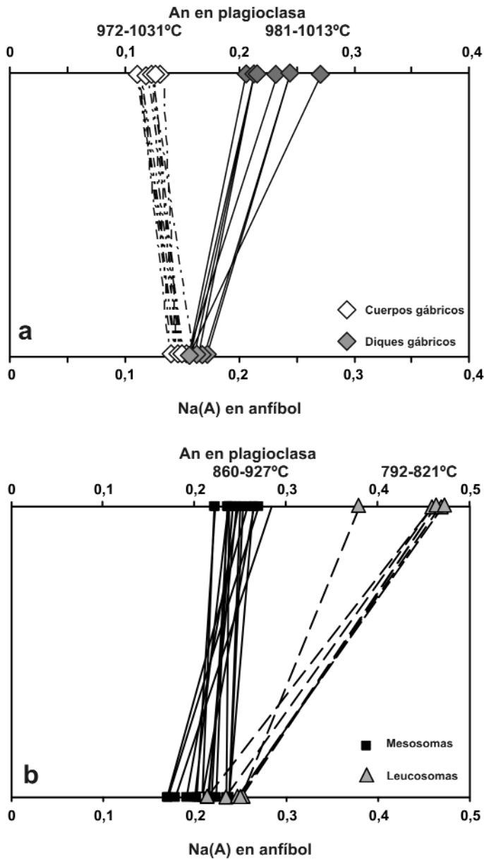
Figura 6: Comparación de plagioclasas y anfíboles coexistentes. Las líneas unen la concentración de albita en plagioclasa con la concentración de Na en sitios A de los anfíboles, el paralelismo observado en la mayoría de los pares minerales sugiere equilibrio químico para la mayoría de las muestras. Los rangos de temperatura se basan en el termómetro Amph-Pl de Holland y Blundy (1994); a) Corresponde a los cuerpos y diques máficos; b) Mesosomas y leucosomas en migmatitas máficas. Los símbolos corresponden a las figuras previas.
