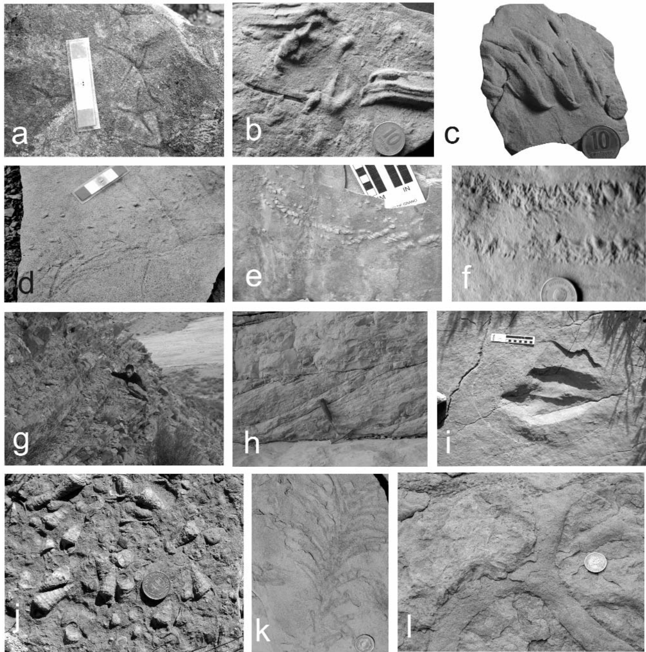
Figura 2: Rasgos sedimentológicos e icnológicos: a) Asteriacites , epirrelieve negativo, Vega de Escalone, foto de campo; b) Vega de Escalone: scratches de vertebrados subácueos-arrastre, con impresión terminal de dedos (CPBA 20677), trazas en hiporrelieve de Gyrochorte (CPBA 20678), cortadas por los scratches semejantes a Characichnos , hiporrelieve positivo; c) Puerta Curaco, hiporrelieve positivo scratch tridígito. CPBA 20679; d) Vega de Escalone: CPBA 20680, trazas de locomoción de artrópodos ( Diplichnites ?) que cortan a Gyrochorte (CPBA 20681), hiporrelieve positivo; e) Vega de Escalone: trazas de locomoción de artrópodos, mostrando desplazamientos laterales, hiporrelieve positivo, foto de campo; f) Vega de Escalone: traza de locomoción de un posible artrópodo con apéndices indiferenciados, hiporrelieve positivo CPBA 20682; g) Vega de Escalone: vista de superficie heterolítica con acreción lateral; h) superficies de reactivación con cortinas de fango; i) huella tridáctila de terópodo en cerro Rayoso, hiporrelieve positivo; j) Bajada del Agrio: coquina integrada por gastrópodos potamídeos con coberturas de briozoarios y serpúlidos, foto de campo; k) Mina La Continental: formas ramosas de Hillichnus hiporrelieve, foto de campo; l) Bajada del Agrio, Ophiomorpha en hiporrelieve, obsérvense los moldes de pellets en el sector superior y las bifurcaciones horizontales, foto de campo.
