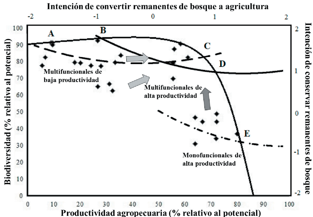
Figura 3. Intersección de las curvas de indiferencia para tres tipos distintos de productores agropecuarios y la curva empírica de compromiso entre conservación y producción (línea llena) en el Chaco Seco argentino. Las letras C y D indican estados del sistema que son, a la vez, biofísicamente posibles y socialmente deseables para los productores multifuncionales de baja productividad (línea de guiones), aunque posibles, pero no deseables, para los productores monofuncionales de alta productividad (línea de guiones y puntos).
