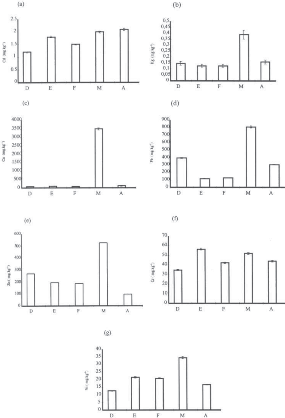
Figura 1. Niveles (mg kg -1 ) de cadmio (a), mercurio (b), cobre (c), plomo (d), cinc (e), cromo (f) y níquel (g) durante el período de muestreo.
