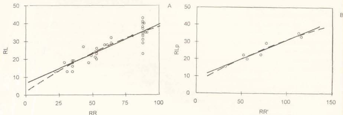
Figura 2. Relación entre la riqueza de especies arbóreas regional y local para las Yungas de Argentina. Línea continua=modelo lineal; línea segmentada=polinomio de segundo orden. (A) considerando todas las localidades (RL) y la riqueza regional según el sector latitudinal y la altitud (RR). Regresión lineal: R^2=0.79 , F=159.8 , P<0.0001 . Polinomio de segundo orden: R^2=0.8 , F=79.6 , P<0.0001 . (B) considerando el promedio de riqueza local para cada piso de vegetación y sector latitudinal (RLp) y la riqueza regional de cada piso y sector (RR'). Regresión lineal: R^2=0.92 , F=57.7 , P<0.001 . Polinomio de segundo orden: R^2=0.92 , F=24.2 , P<0.005 .
