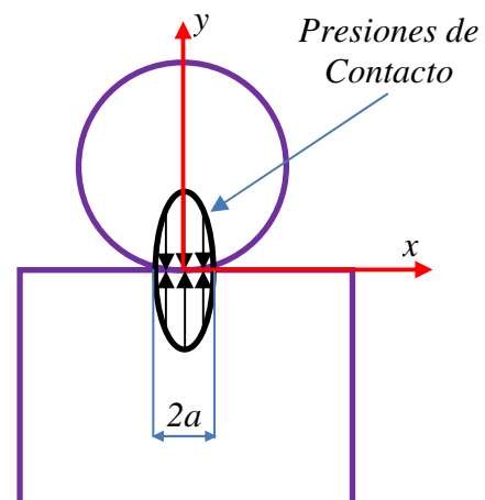
Figura 4 – Geometra y Presiones de contacto en un sistema cilindro contra plano.
